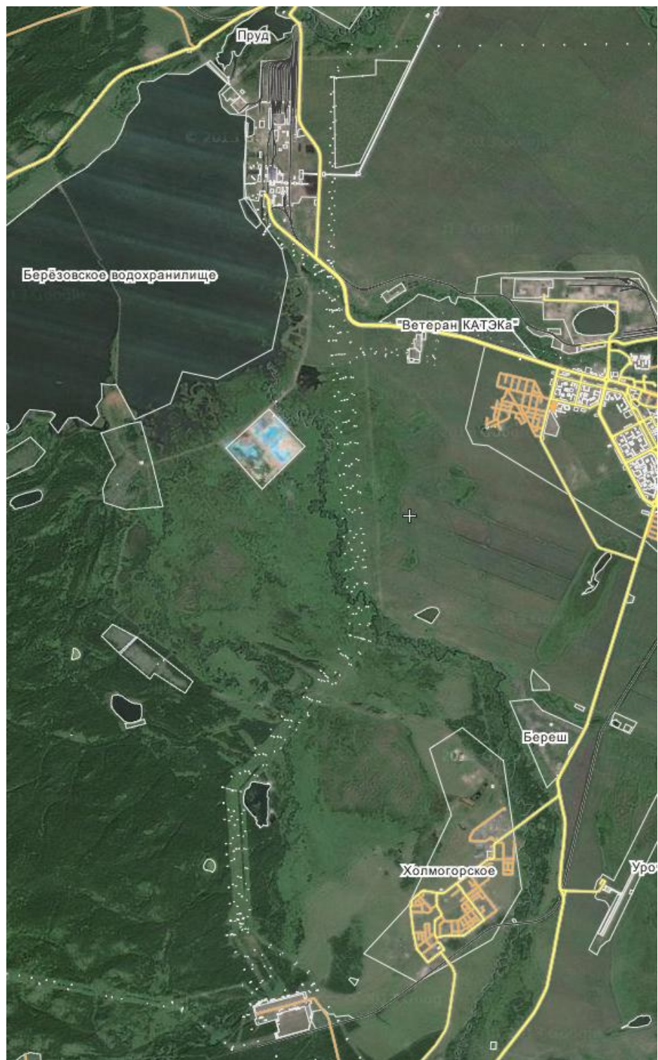
Рисунок 1- Трасса ВЛ 500 кВ Берёзовская ГРЭС- ПС «Итатская»
