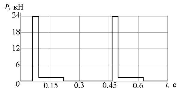
Рис. 5. График изменения силы ударного импульса по времени при использовании встроенного упругого элемента в промежуточной полости. Упругая среда
