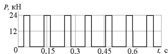
Рис. 3. График изменения силы ударного импульса по времени при использовании встроенного упругого элемента в промежуточной полости. Упругая среда
