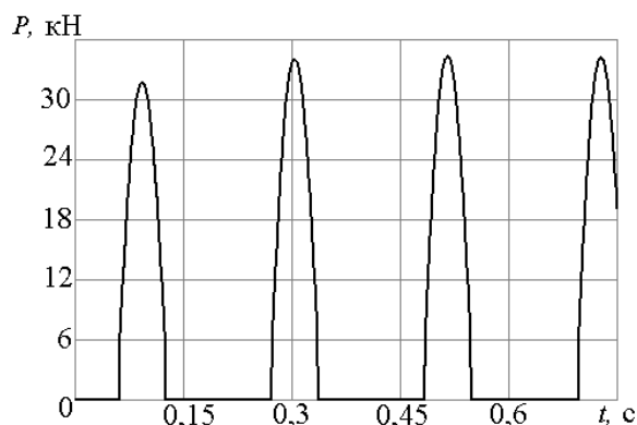
Рис. 2. График изменения силы ударного импульса по времени при использовании встроенного упругого элемента в промежуточной полости. Упругая среда
