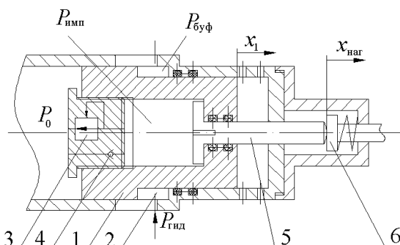
Рис. 4. Принципиальная схема промежуточной полости с встроенным регулируемым клапаном: 1) поршень-боек; 2) гидравлическая полость; 3) регулируемый клапан; 4) обратный клапан; 5) промежуточный боек; 6) наголовник
