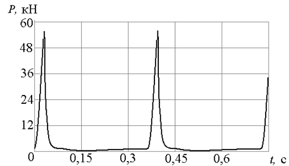
Рис. 7. График изменения силы ударного импульса по времени при использовании встроенного дросселя в промежуточной полости. Вязкоупругая среда
