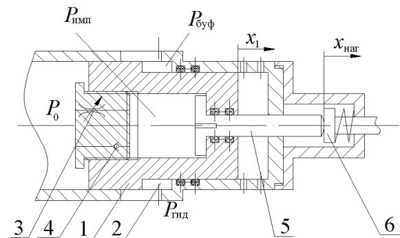
Рис. 6. Принципиальная схема поршня-бойка с встроенным регулируемым дросселем: 1) поршень-боек; 2) гидравлическая полость; 3) регулируемый дроссель; 4) обратный клапан; 5) промежуточная полость; 6) наголовник
