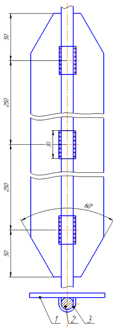
Рисунок 9 – Скребок пластинчатый
