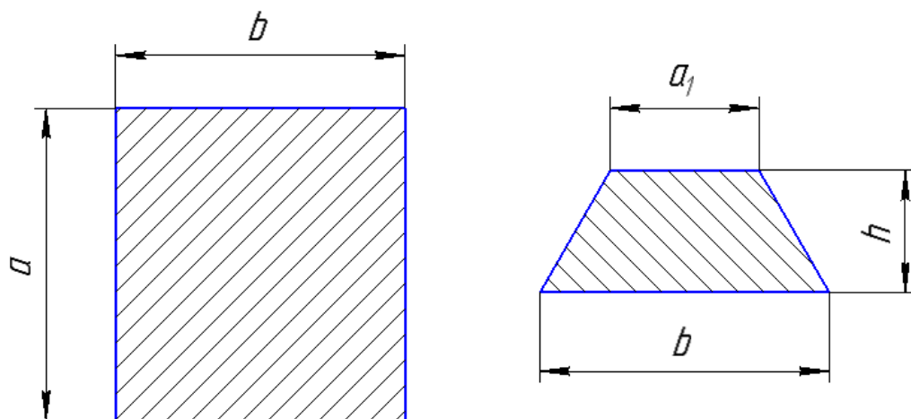
Рисунок 12 – Геометрические параметры пластинчатого скребка
