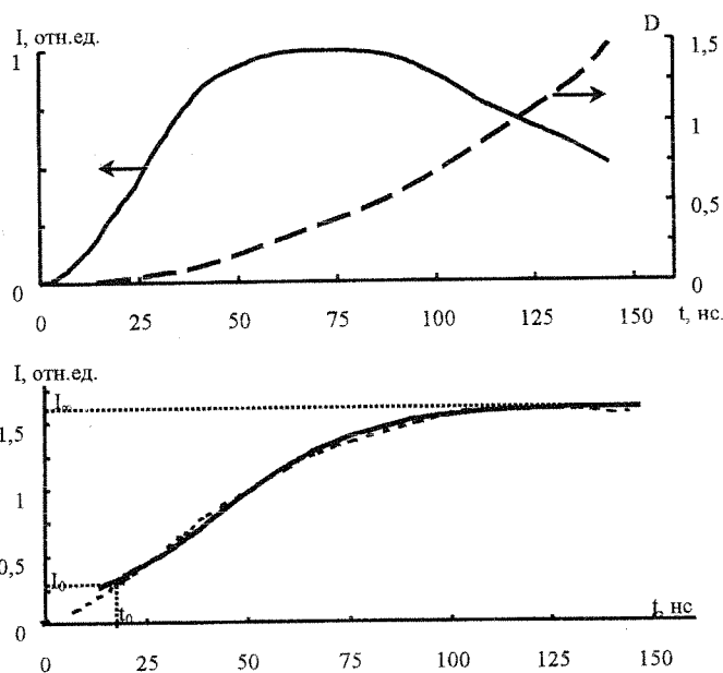
Рис. 6. Кинетика предвзрывной люминесценции нитевидного кристалла азидо серебра при \lambda = 550 \text{ нм} . (Иницирование импульсом лазера) а – люминесцентный сигнал (сплошная линия) и оптическое поглощение (пунктир).
