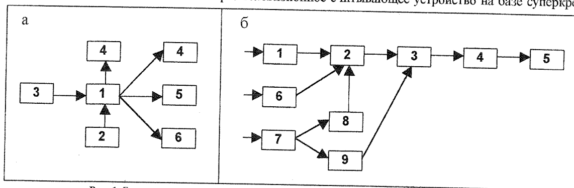
Рис. 1. Блок-схема экспериментального комплекса для исследования взрывного разложения.
