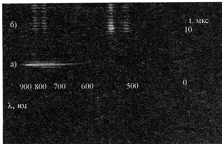
Рис. 4. Изображение спектра (ЭОПограмма) взрывного свечения макрокристалла \text{AgN}_3 на экране фотохронографа.
