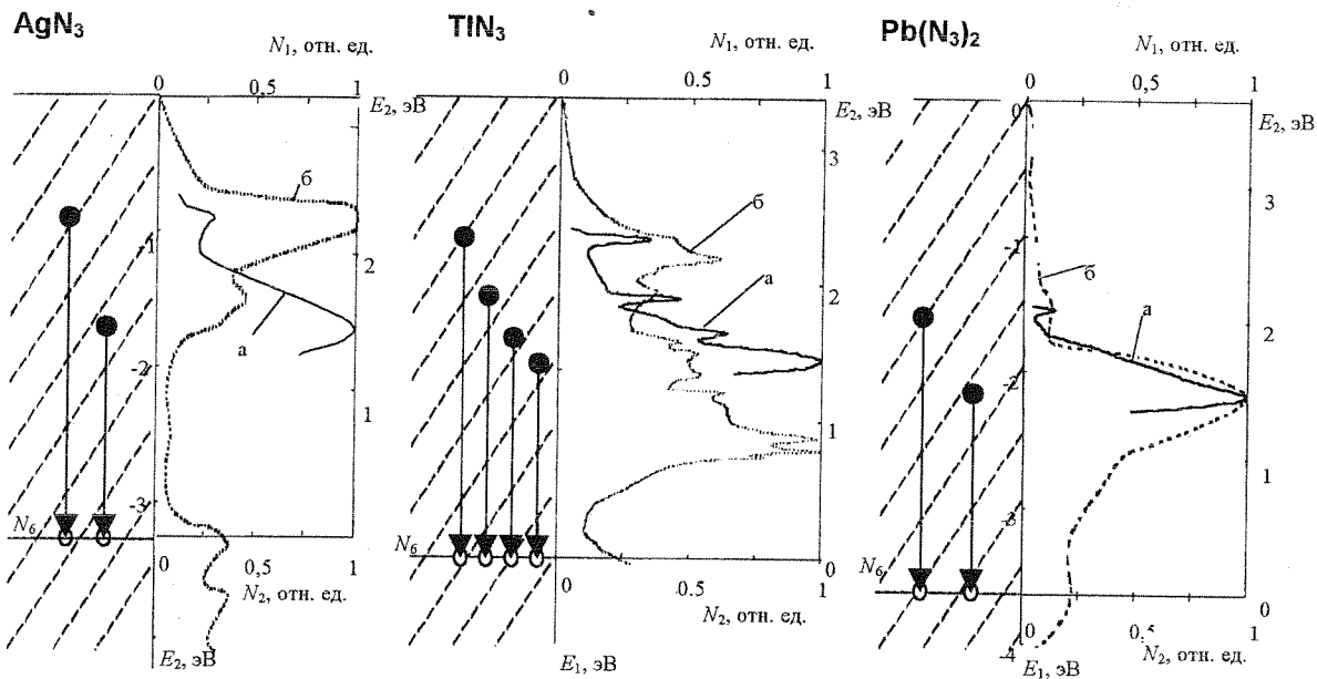
Рис. 7. Сопоставление спектров предвзрывной люминесценции (а) и плотности состояний в валентной зоне (б) для азидов серебра, таллия и свинца.
