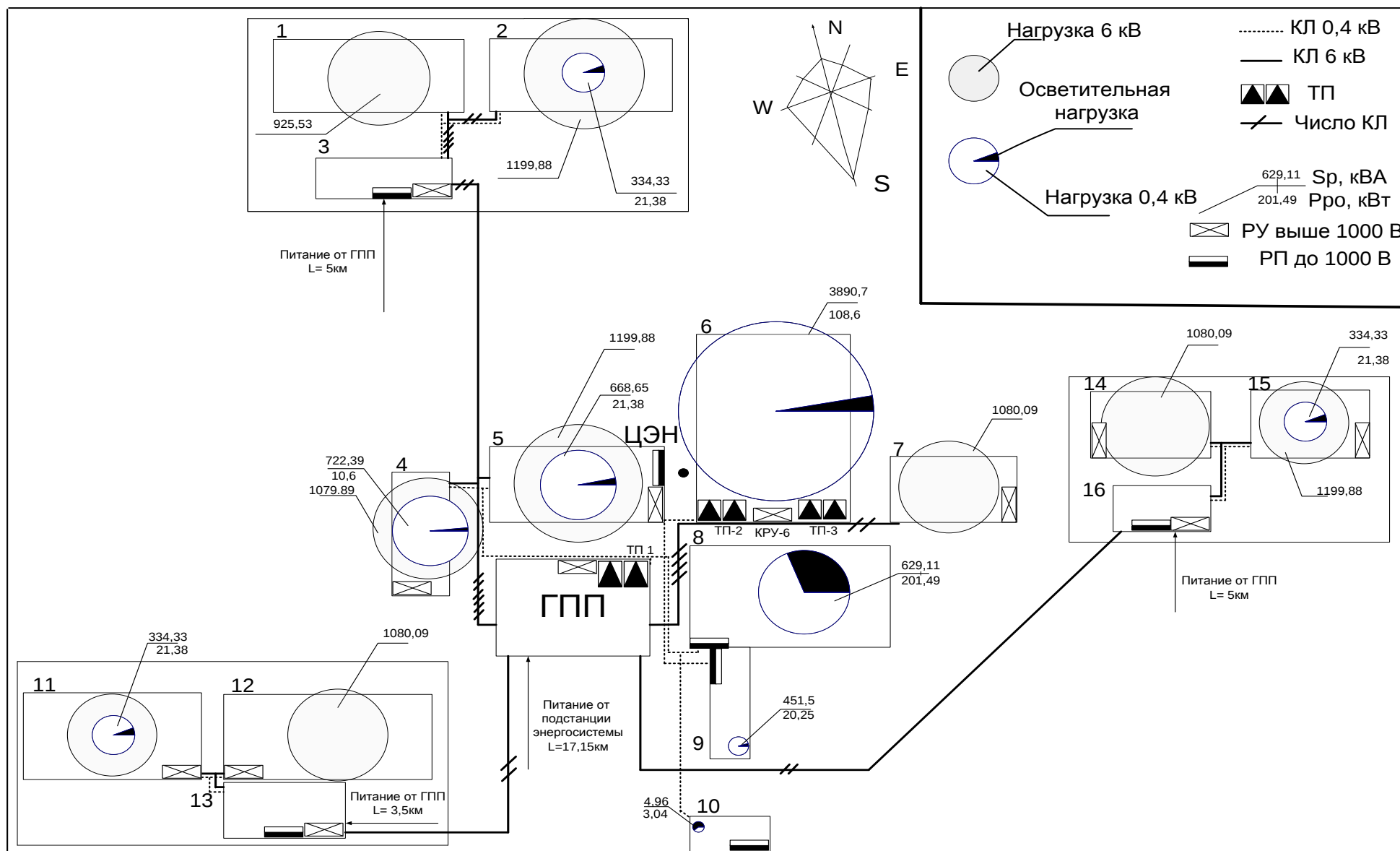
Рисунок 3 - Картограмма электрических нагрузок
