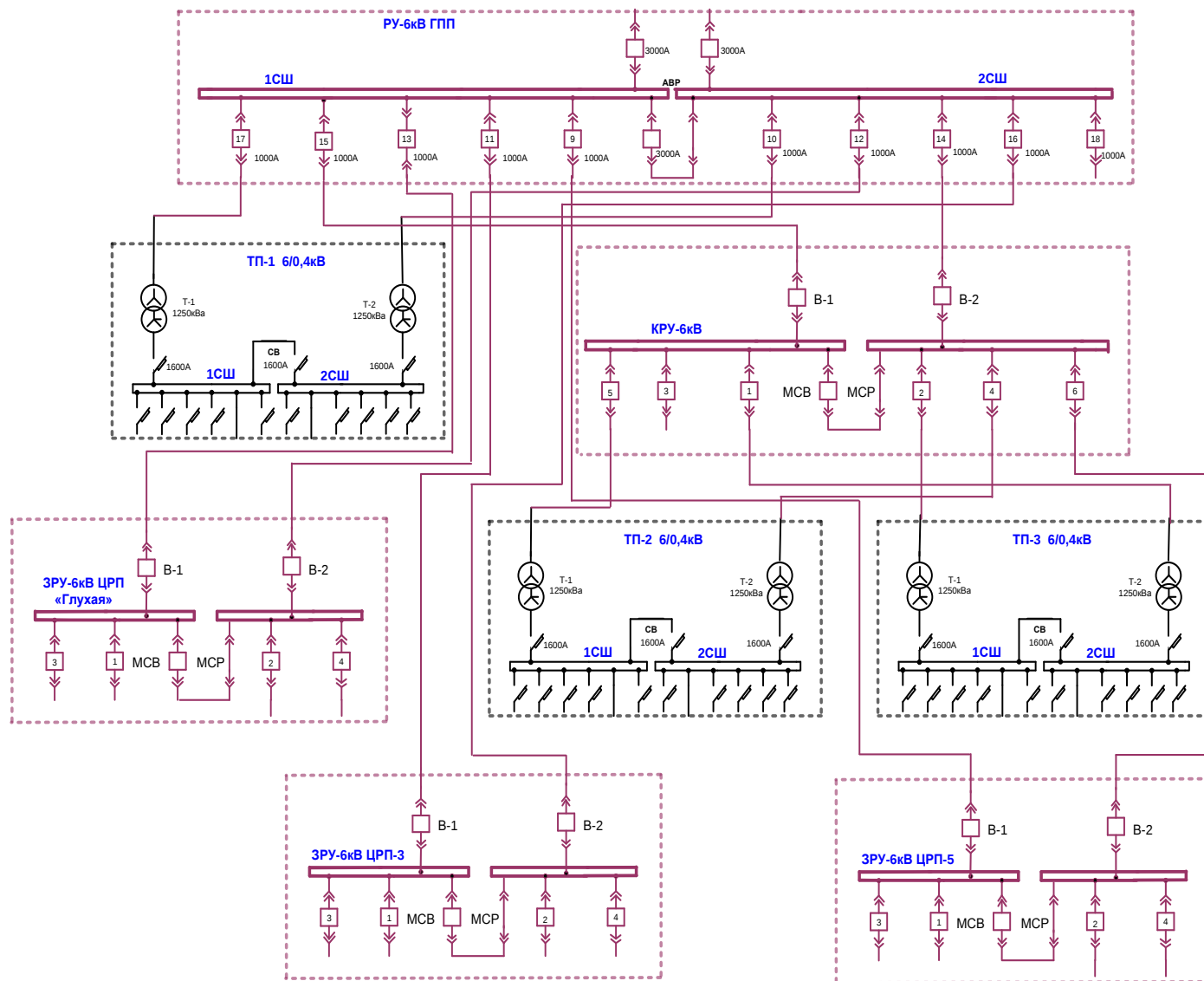
Рисунок 4 - Схема внутризаводского электроснабжения
