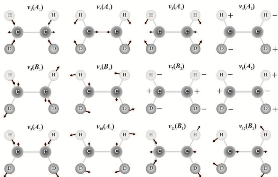
Рисунок 2 – Нормальные координаты колебаний \text{cis-C}_2\text{H}_2\text{D}_2 молекулы (группа симметрии C_{2v} )
