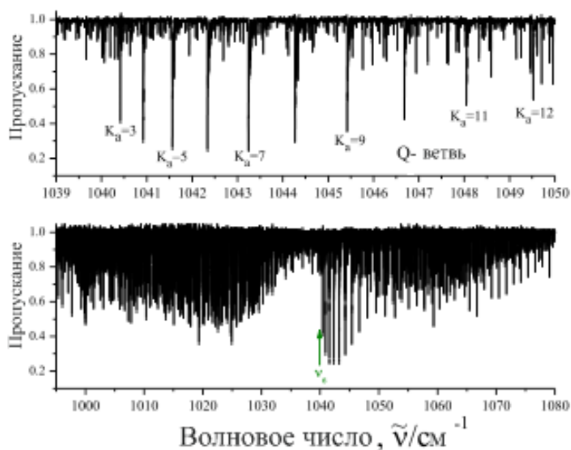
Рисунок 6 – Верхняя часть: фрагмент экспериментального спектра высокого разрешения \text{cis-C}_2\text{H}_2\text{D}_2 в области Q – ветви полосы \nu_7 . На рисунке обозначен набор переходов относящихся к Q – ветви серии K_a = 3 полосы \nu_7 . Нижняя часть экспериментальный спектр полосы \nu_7 .
