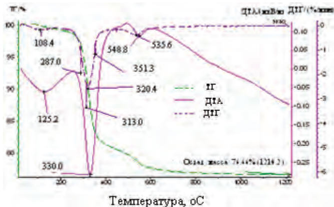
Рис. 1. Кривые термического анализа высокожелезистого боксита
