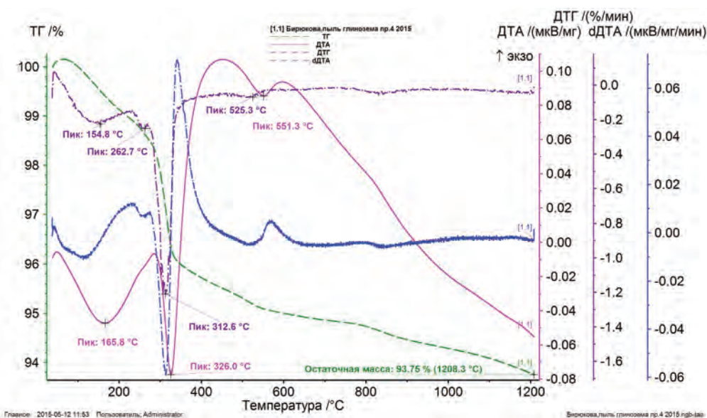
Рис. 2. Кривые термического анализа глиноземистой пыли
