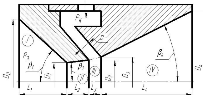
Рис. 1. Расчетная схема эжекторного волоконобразующего устройства
