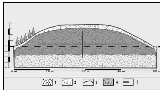
Рис. 1 Схема строения гряды: 1 – пески, 2 – льдонасыщенные опалиты, 3 – граница сезонного талого слоя, 4 – «ядро» гряды с максимальными значениями льдистости, 5 – уровень поверхности
