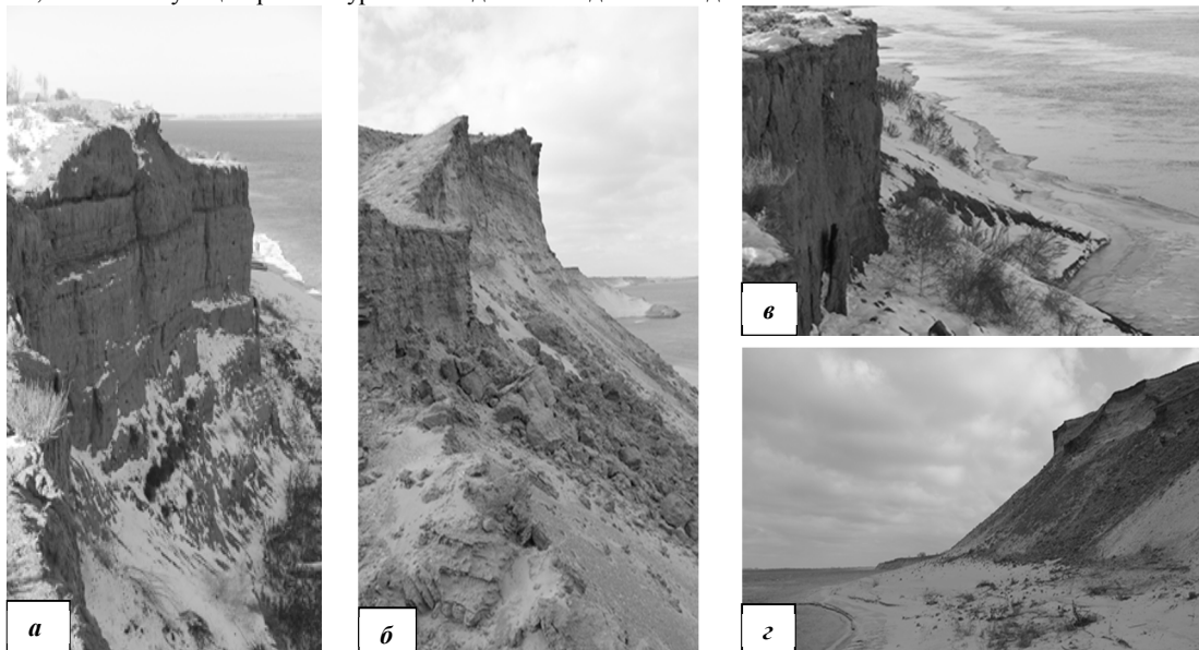
Рис. 2. Морфологические типы береговых уступов
