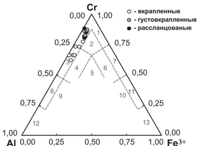
Рис. 1. Составы акцессорных и рудных хромшпинелидов в породах Харчерузского блока массива Сьумкеу (Полярный Урал) и их зависимость от густоты вкрапленности на классификационной диаграмме Н.В. Павлова [2]. Шпинелиды: 1 – хромит, 2 – субферрихромит, 3 – аллюмохромит, 4 – субферриаллюмохромит, 5 – ферриаллюмохромит, 6 – субаллюмоферрихромит, 7 – феррихромит, 8 – хромпикотит, 9 – субферрихромпикотит, 10 – субаллюмохром-магнетит, 11 – хроммагнетит, 12 – никотит, 13 – магнетит
