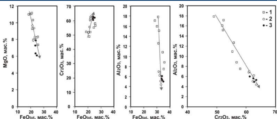
Рис. 2. Связь между содержанием Cr_2O_3 , Al_2O_3 , MgO и содержанием FeO_{tot} (общее) в хромшпинелидах из пород Харчерусского блока: 1-3 – хромшпинелиды по степени вкрапленности: 1 – акцессорные вкрапленные, 2 – густовкрапленные, 3 – густовкрапленные расланцованные
