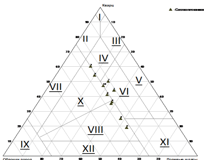
Рис 1. Классификационная диаграмма В.Д. Шутова с результатами количественно-минералогического анализа. Поля на диаграмме, песчаники: I – мономиктовые кварцевые, II – кремнекlasto-кварцевые, III – полевошпато-кварцевые, IV – мезомиктовые кварцевые, V – собственно аркозовые, VI – граувакковые аркозы; VII – граувакки кварцевые, VIII – полевошпато-кварцевые, IX – собственно граувакки, X – граувакки кварц-полевошпатовые, XI – полевошпатовые, XII – песчаники не терригенного происхождения
