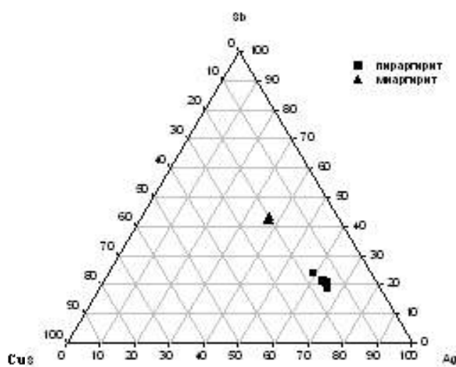
Рис. 4. Соотношение основных компонентов в сульфоантимонитах свинца и серебра
