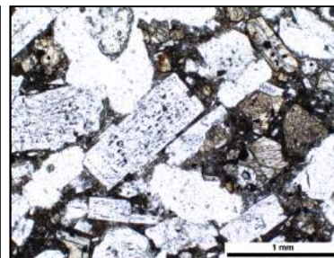
Рис. 2. Микроструктуры андезибазальтов: слева - порфировая и пилотаксовая (с анализатором), справа – стекловатая с порфировыми вкрапленниками (без анализатора)
