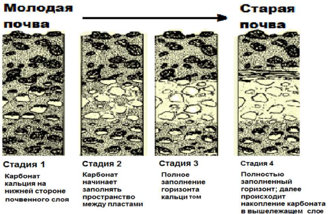
Рис. 1. Постадийное формирование скоплений каличе [6]
