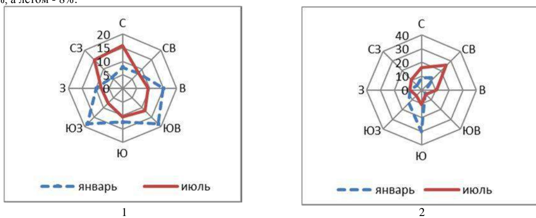
Рис.2 Розы ветров метеостанций Марресалья(1) и Салехард(2)
