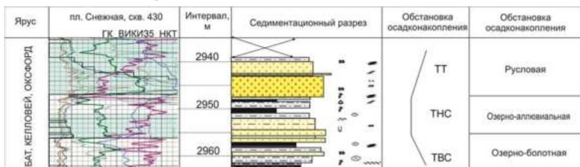
Рис. 1. Вертикальная седиментационная модель тюменской свиты
