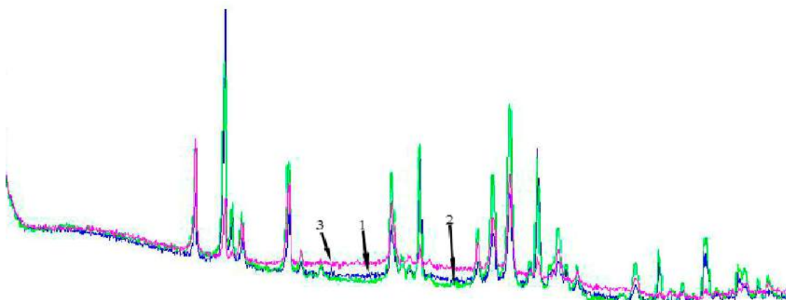
Рис. 2. Рентгенограмма урат-оксалатного уrolита: 1 – центральная слабо сцементированная зона; 2 – внешняя плотная зона; 3 – зона с ярко выраженными кристаллами (Центр коллективного пользования «Геохимии природных систем» (ЦКП «ГПС») ТГУ, аналитик Т.С. Небера)
