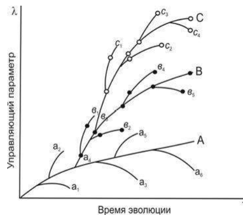
Рис. Схема последовательного усложнения состава водного раствора в ходе глобальной эволюции Материнские системы: А – вода – порода; В – вода – растения; С – вода – животные Дочерние системы: а 1 - а 5 -ветви А; b 1 - b 5 -ветви В; с 1 - с 4 -ветви С
