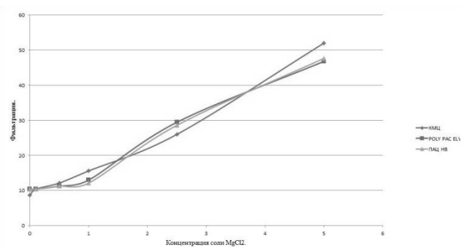
Рис 3. Зависимость фильтрации от концентрации соли \text{MgCl}_2 .
