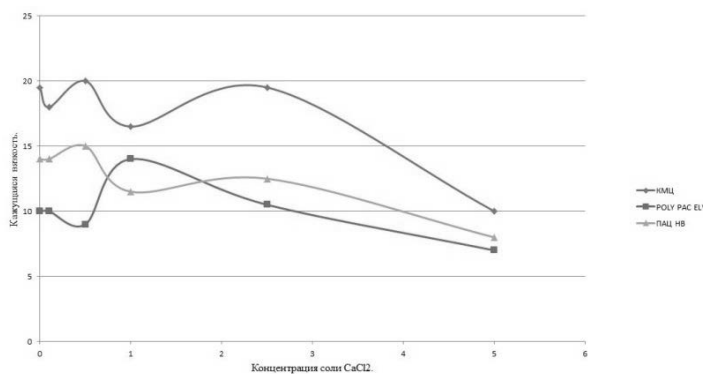
Рис 4. Зависимость Кажущейся Вязкости от концентрации соли \text{CaCl}_2 .
