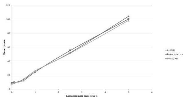
Рис 2. Зависимость фильтрации от концентрации соли \text{FeSO}_4 .
