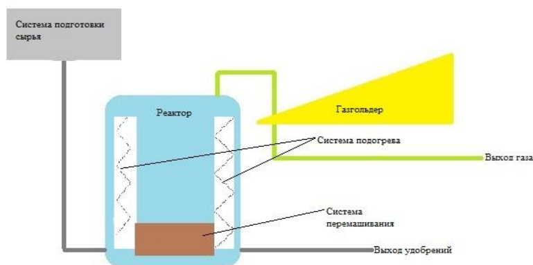
Рисунок 1– Принципиальная схема биогазовых установок
