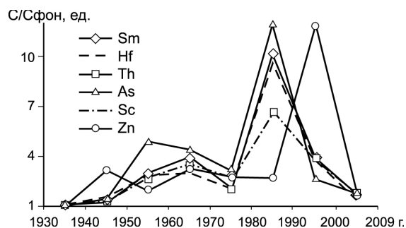
Рис. 2. Надфоновое содержание элементов (C/Сфон) в золе лиственницы из пункта Кайсын
