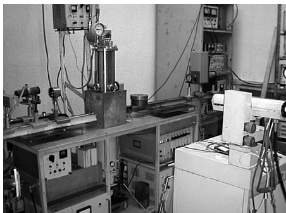
Рис. 2. Импульсный оптический спектрометр
