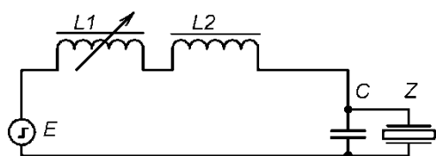
Рис. 5. Согласующий контур с перестраиваемым дросселем
