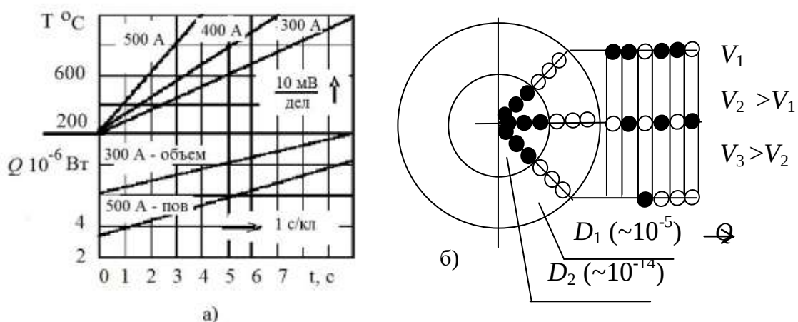
Рисунок 1. а) осциллограммы изменения температуры и потока кислорода от времени; б) условная схема перераспределения потоков газа при различных скоростях нагрева
