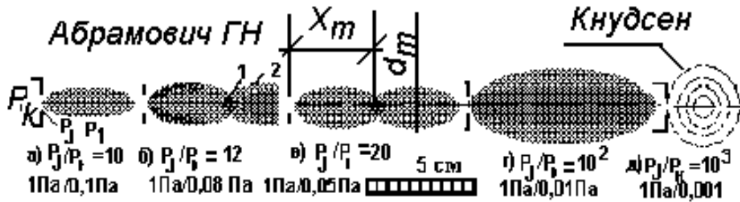
Рисунок 2 – Форма потока пара цинка при визуализации в тлеющем разряде
