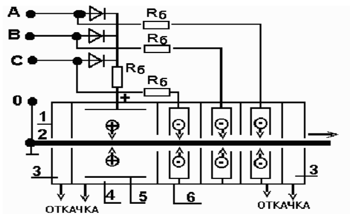
Рисунок 7 – Схема устройства для приоритетной электронной или ионной обработки стальных проволок. 1 – корпус, 2 – проволока, 3 – камера промежуточной откачки, 4 – генератор плазмы, 5 – анод, 6 – нагреватели.
