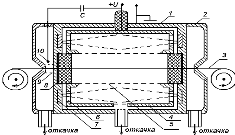
Рисунок 6 – Схема устройства для ионной очистки и отжига вольфрамовых проволок. 1 – корпус; 2 – камера промежуточной откачки; 3 – проволока; 4, 5 – цилиндры; 6 – анод; 7 – катод; 8 – держатели, 9 – сетка, 10 – электрод
