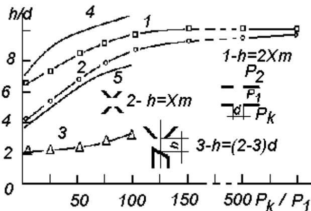
Рисунок 5 – Зависимость оптимального расстояния между элементами от перепада давления на первой ступени откачки. 1, 2, 3 – эксперимент; 4, 5 – расчет для плоских и острых выводных элементов
