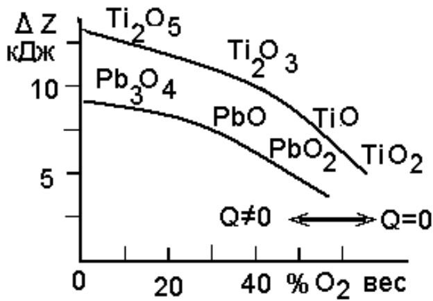
Рисунок 3 – Тенденция смещения диаграммы изобарного потенциала при изменении расхода напускаемого газа
