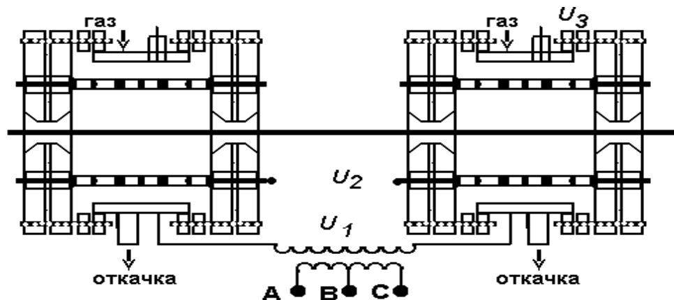
Рисунок 8 – Схема устройства для обработки электродной проволоки
