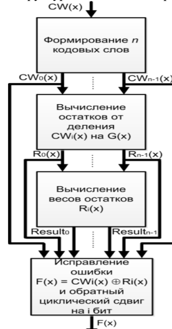
Рис. 3. Структурная схема декодера БЧХ-кода
