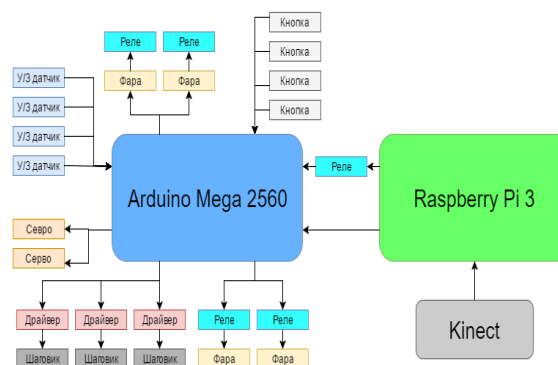
Рисунок 2 – Принципиальная схема
