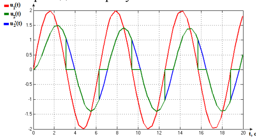
Рис.5 – Реакция НКУ на синусоидальный входной сигнал
