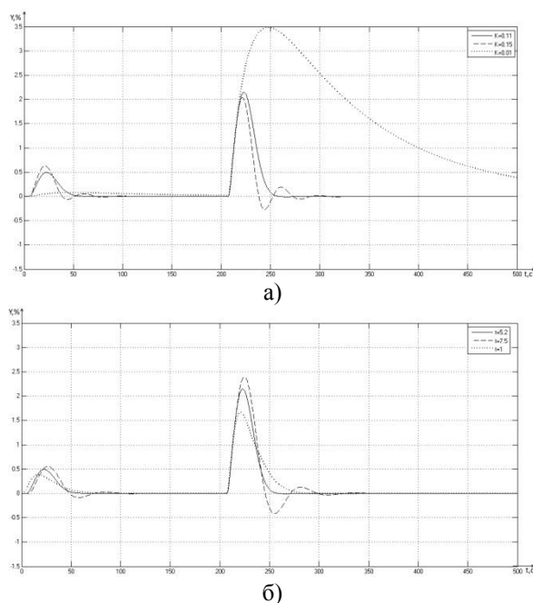
Рис. 4. Результаты моделирования САУ
