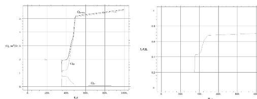
Рис. 3. Дебит и обводненность продукции на добывающей скважине при закачке оторочки
