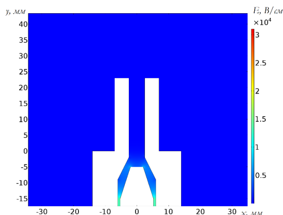
Рис. 2. Картина напряженности электрического поля плазмотрона
