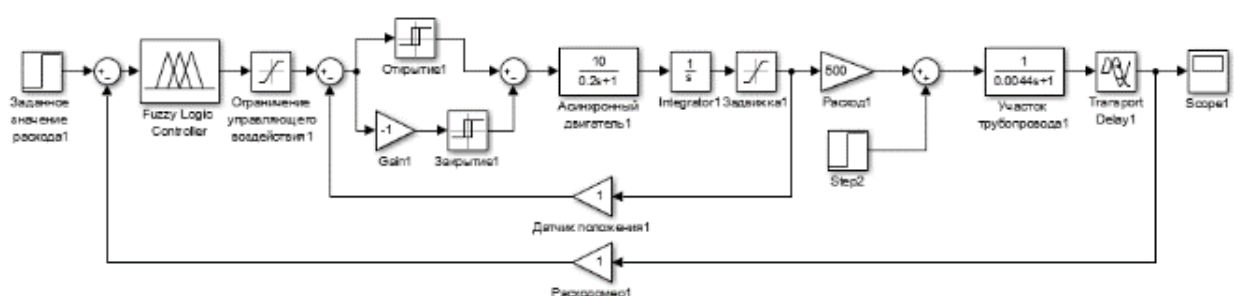
Рис. 1. Система с нечетким регулятором
