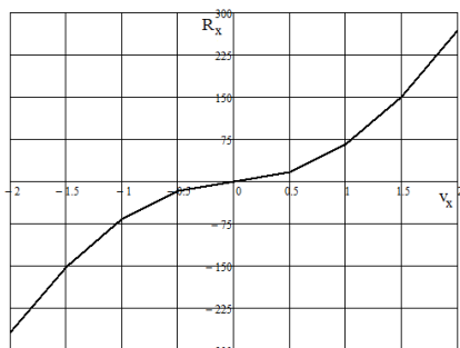
Рис. 3. Зависимость силы лобового сопротивления исследуемого ТНПА R_x от скорости движения v_x
