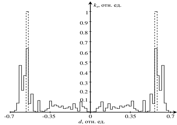
Рис. 2. Распределения нормированной концентрации неоднородностей вдоль радиуса сердцевины GI-POF
