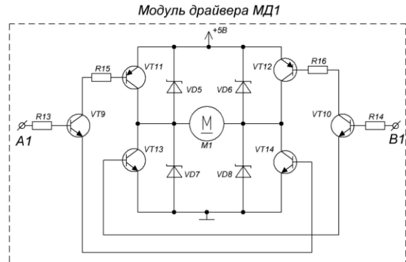
Рис. 1. Н-мост для управления первого двигателя
