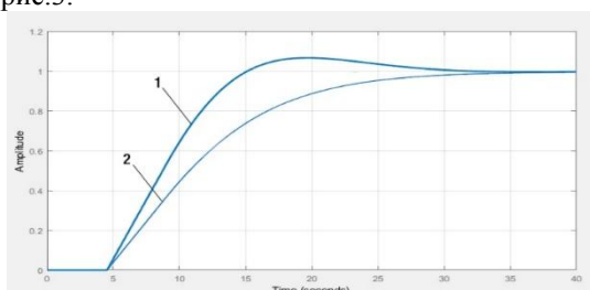
Рис. 3. Графики переходных процессов: 1 – ПИД-регулятор, 2 – нечеткий регулятор
