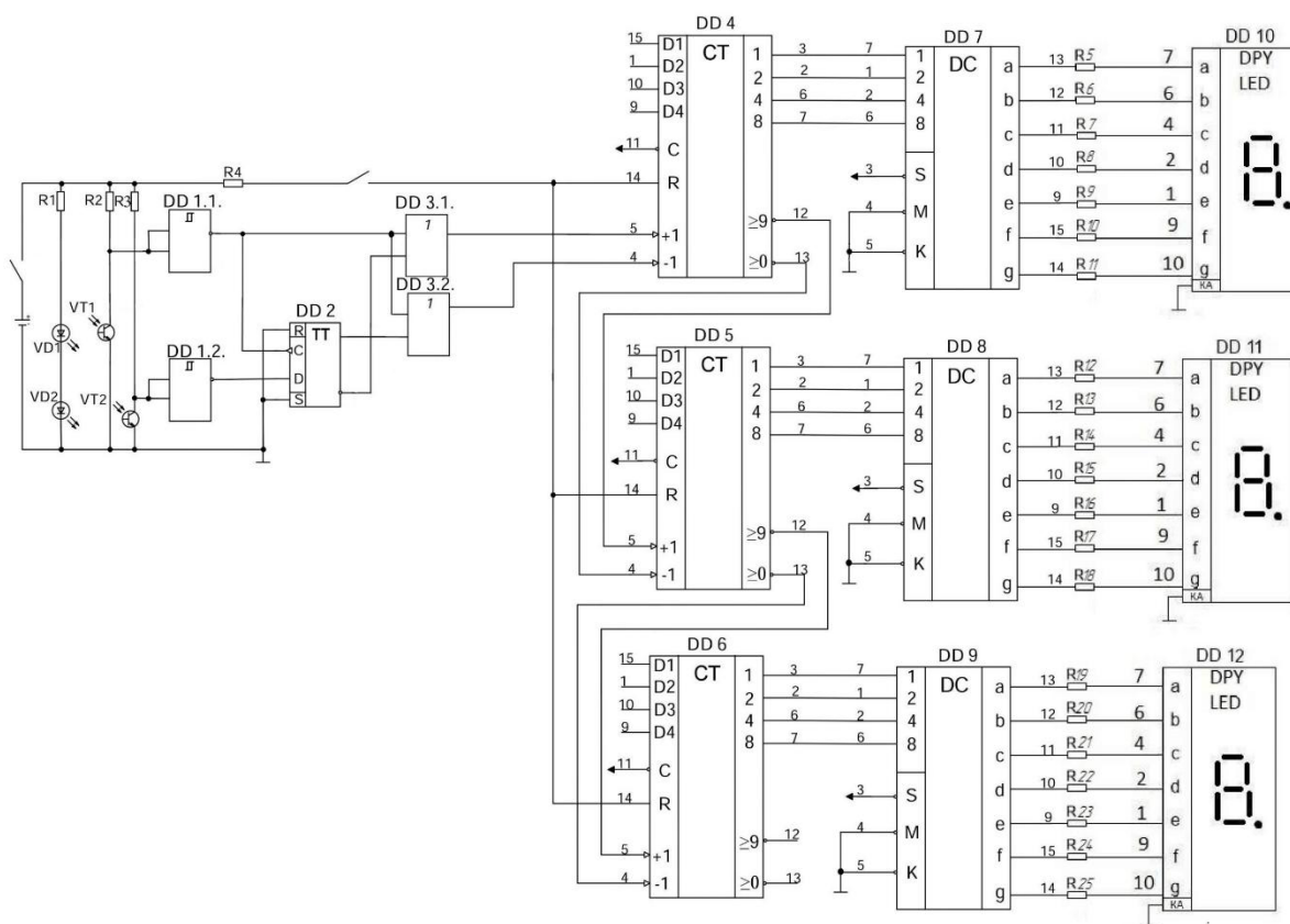
Рис. 2. Электрическая схема устройства роликового измерителя длины
