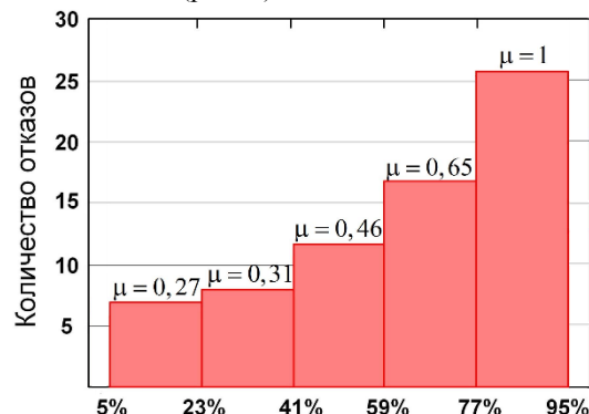
Рис. 1. Гистограмма плотности распределения отказов промышленных трубопроводов
