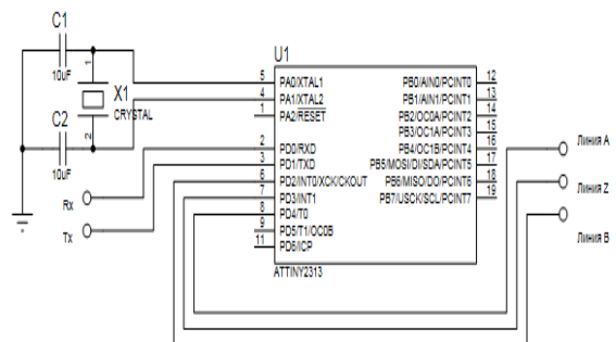
Рис.2. Принципиальная схема обработки значения энкодера
