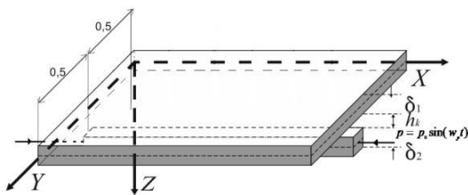
Рис.1 Расчетная схема.
