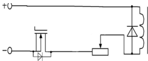
Рис. 3 Электромагнит
