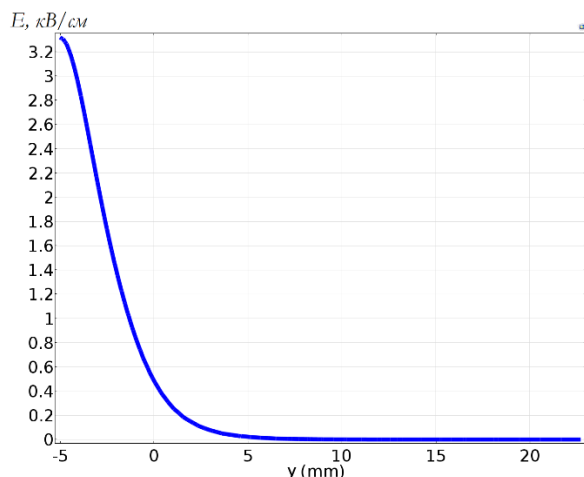
Рис. 3. Общий вид зависимости НЭП на оси плазматрона от расстояния до катода
