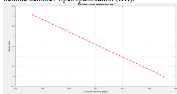
Рис. 1. ФЧХ
