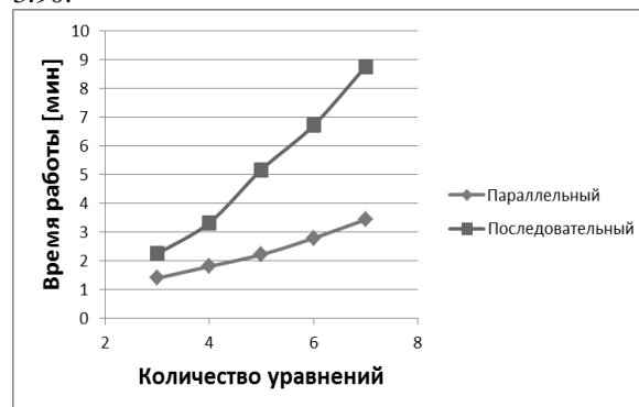
Рисунок 14. Зависимость времени работы алгоритма от количества уравнений
