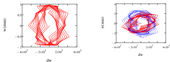
а) Пластика 2 б) Пластика 1 Рис. 9. Фазовые портреты
