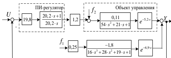
Рис. 1. Модель типовой САУ
