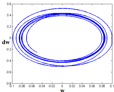
Рис. 2. Фазовый портрет нижней пластинки при нагрузке p_0 = 0.10145
