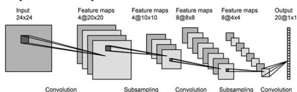
Рис. 1. Схема архитектуры свёрточной нейронной сети
