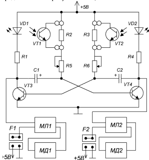
Рис. 3 Принципиальная электронная схема управляющей части платформы
