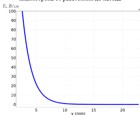
Рис. 4. Распределение НЭП в плазматроне (детально)
