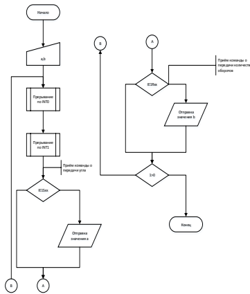
Рис.3. Блок-схема контроллера обработки данных с энкодера
