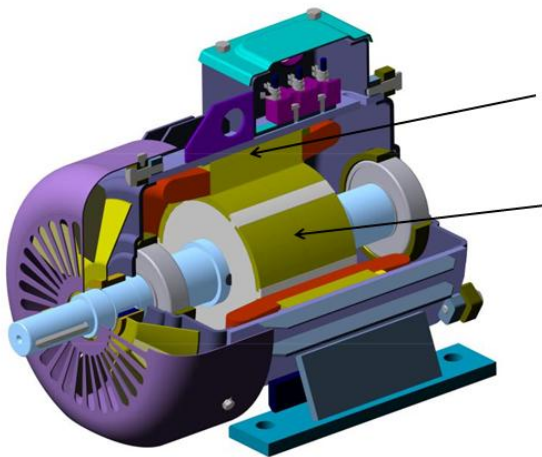
Рис. 1. Конструкция СДПМ
