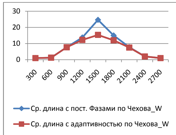
Рис. 5. График двух режимов по Чехова_W
