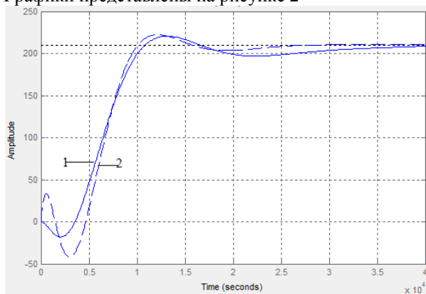
Рисунок 2. Графики переходных процессов желаемой (1) по ВИМ и синтезируемой (2) по Паде замкнутого контура
