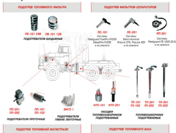
Рис. 1. Схема установки подогревательных элементов
