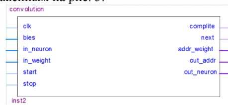
Рис. 3 Модуль свёрточного слоя
