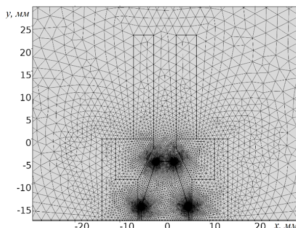
Рис. 1. Сетка конечных элементов
