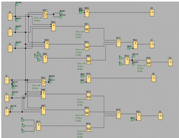
Рис. 5 - Программа на языке FBD
