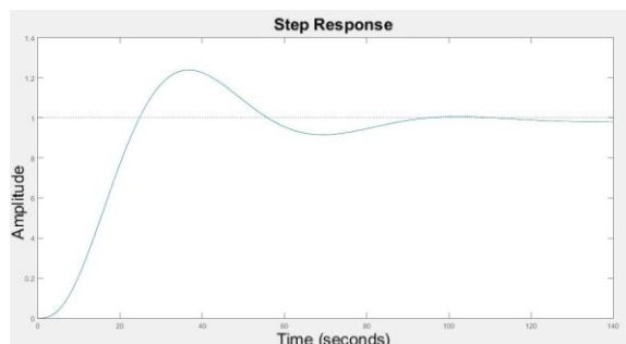
Рис. 12. Переходный процесс САР с ПИД-регулятором
