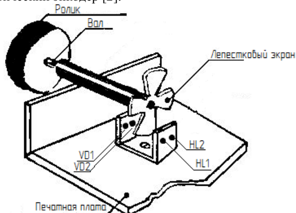
Рис. 1. Расположение оптопары и экрана
