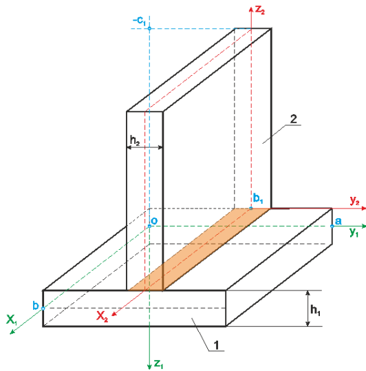
Рис.1. Расчетная схема
