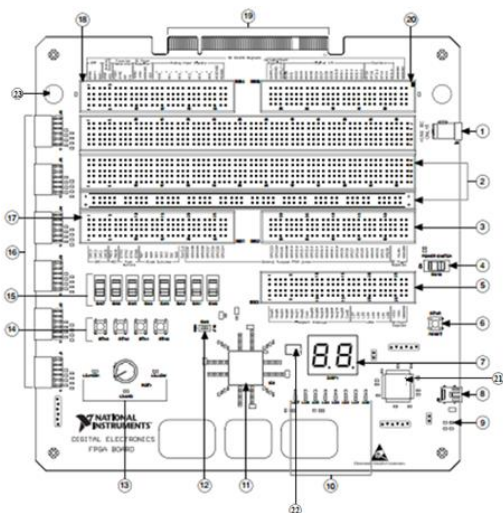
Рис. 2. Внешний вид платы NI Digital Electronics FPGA Board: 1– разъем питания (15В) ; 2–макетной платы для возможности создания дополнительной обвязки; 3– блок макетной платы BB2; 4– выключатель питания; 5– блок макетной платы BB3; 6– кнопка сброса; 7– семисегментные индикаторы; 8– USB-соединитель; 9– LD-G-светодиод; 10– светодиоды; 11– FPGA Xilinx Spartan 3E; 12– переключатель прошивки ПЛИС через ROM/JTAG ; 13– датчик угла поворота с кнопкой; 14– кнопки; 15– движковые переключатели; 16– 6 коннекторов типа PMOD (2x6); 17– блок макетной платы BB1; 18– блок макетной платы BB4; 19– (NI ELVIS)-соединитель; 20– блок макетной платы BB5; 21 – программатор; 22– кварцевый генератор 50МГц; 23– защита платы от статического электричества.
