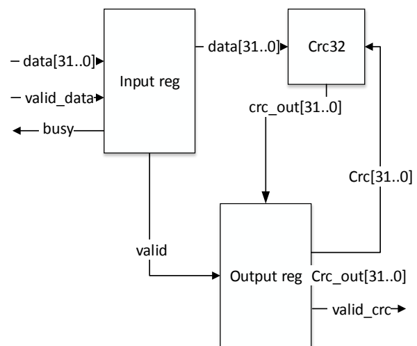
Рис. 1. Структурная схема модуля подсчета контрольной суммы CRC32 матричным методом с накоплением. Если количество обработанных слов меньше чем заданный параметр, контрольная сумма передается обратно в блок Crc32. После накопления суммы итоговая контрольная сумма инвертируется и отправляется дальше (Crc_out). Valid_crc указывает на актуальность записанной в регистре контрольной суммы.
