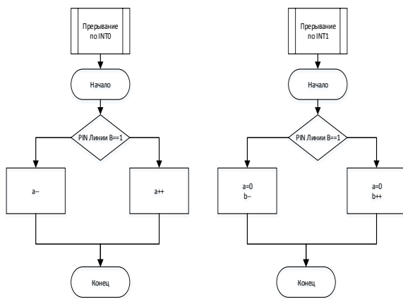
Рис.4. Блок-схема контроллера обработки данных с энкодера (продолжение)
