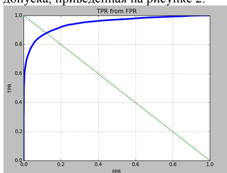
Рис. 2. Зависимость доли истинно-положительных (TPR) от доли ложно-положительных (FPR) срабатываний
