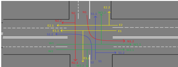
Рис. 8. План-схема перекрестка
