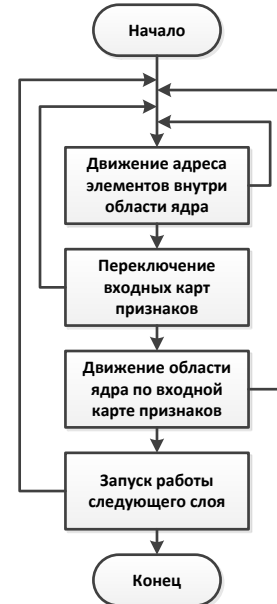
Рис. 2 Алгоритм работы блока контроллера памяти
