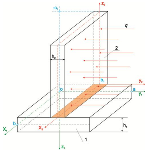
Рис. 1. Расчетная схема.
