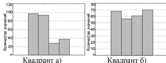
Рис. 3. Гистограммы распределений значений фаз по квадрантам для фреймов со вставкой (а) и без вставки (б)
