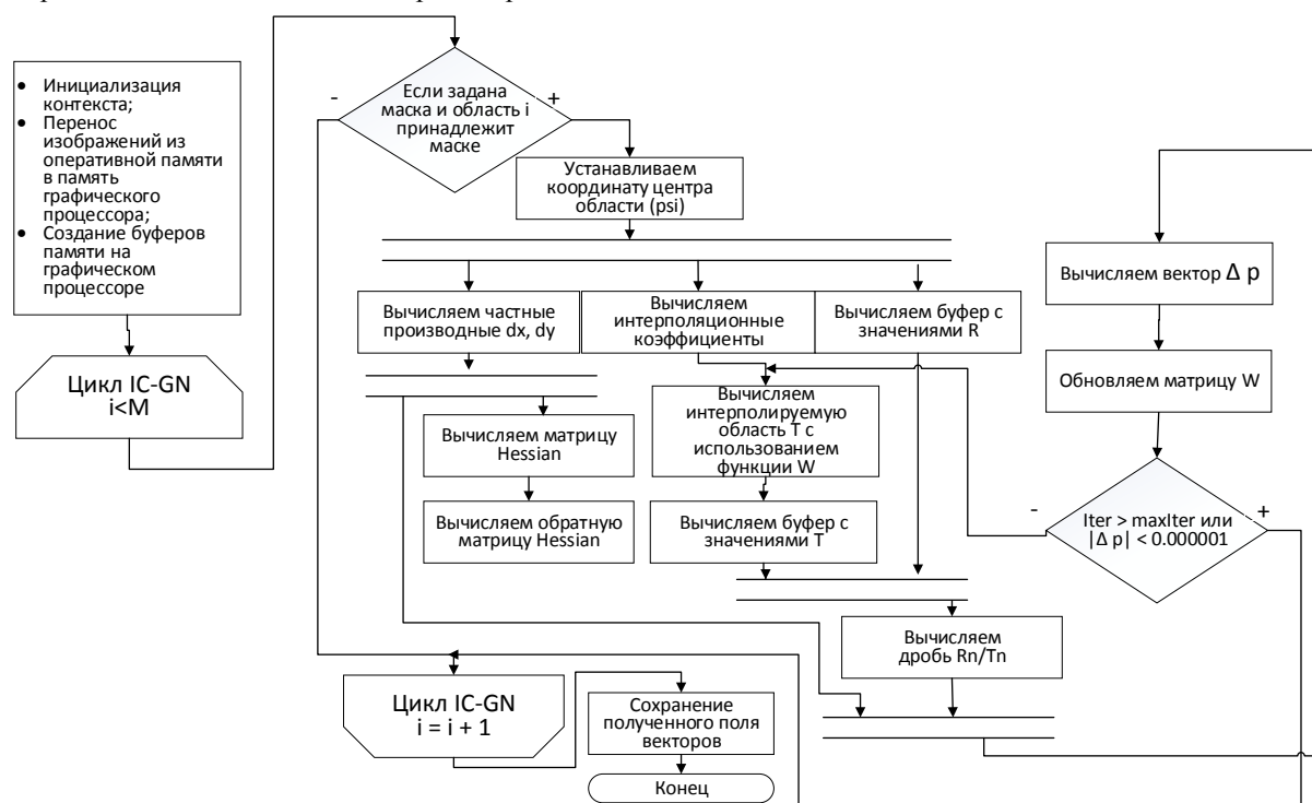
Блок-схема многопоточного алгоритма
