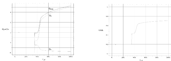
Рис. 2. Дебит и обводненность продукции на добывающей скважине при закачке реагента
