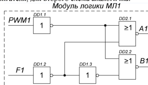
Рис. 2. Логика управления двигателем
