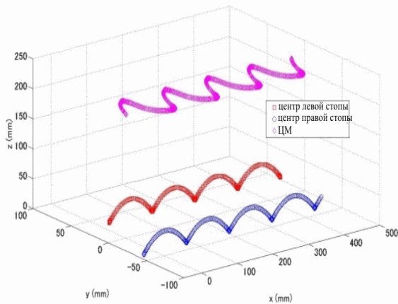
Рис. 3. Траектория движения стоп и ЦМ
