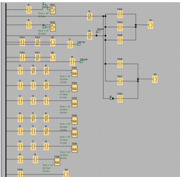
Рис. 6 – Программа на языке LAD
