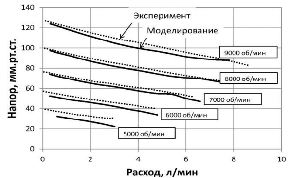
Рис. 3 – Расходно-напорные характеристики численного моделирования и натурального эксперимента.
