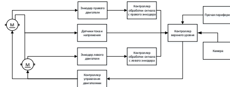
Рис.1. Структурная схема мобильного робота
