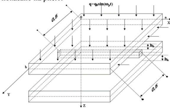
Рис. 1. Схема многослойной структуры из двух пластин и балки
