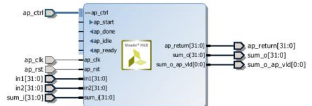
Рис. 3. RTL блок, полученный в результате синтеза примера.
