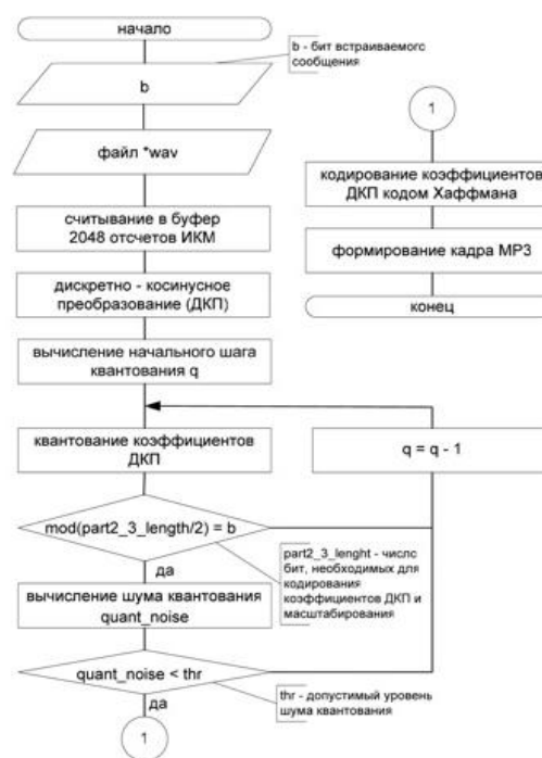
Рис. 1. Алгоритм сжатия информации
