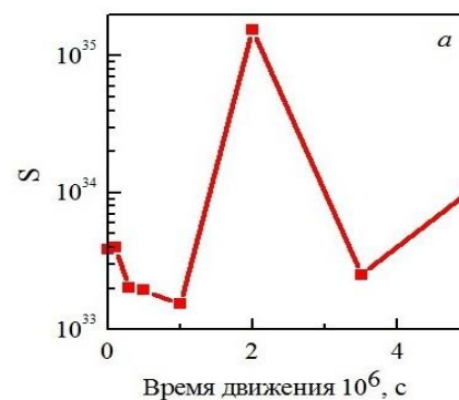
Рис. 1. Изменение на интервале интегрирования для задачи Коши [2-5] коэффициента жесткости S
