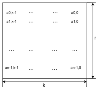
Рис. 1. Предварительно вычисленная матрица
