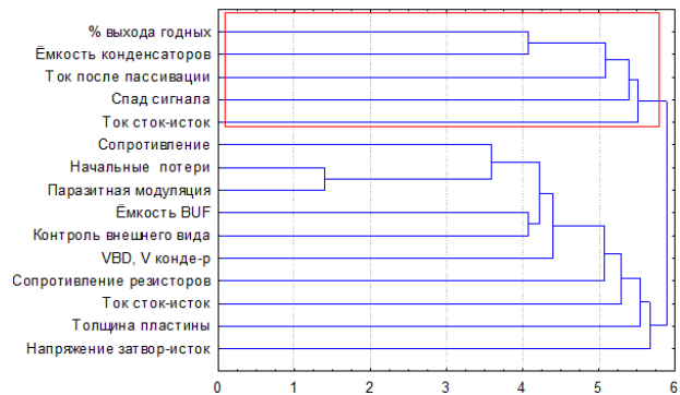
Рис.5. Дендрограмма
