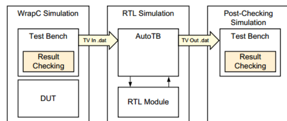
Рис. 1. Шаги RTL-верификации.
