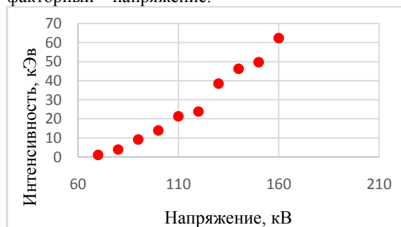
Рисунок 1. Диаграмма рассеивания
