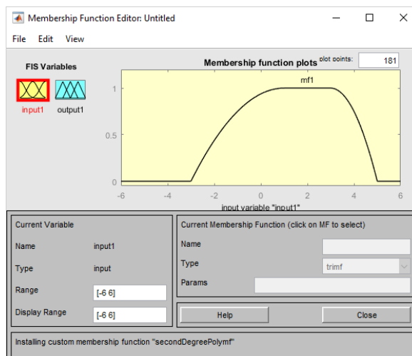
Рис. 3. Пример реализации пользовательской ФП
