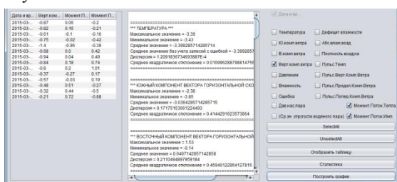
Рис. 1. Заполненный фрейм
