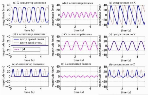
Рис. 2. Суперпозиция осцилляторов
