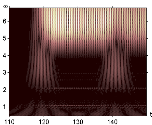
Рис.3 2D вейвлет-спектра для пластинки.
