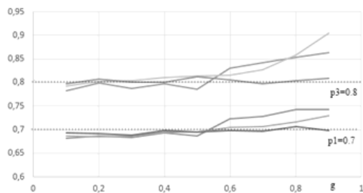
Рис.2. Зависимость рекомендуемых цен от g для T_1=0.5 , g=0.7
