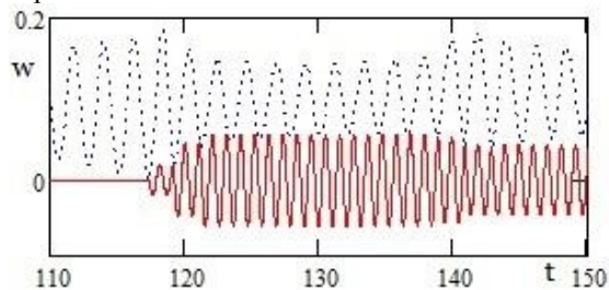
Рис.2 Сигналы балки (пунктир) и пластинки (сплошная линия) соответственно при \varepsilon = 0 .
