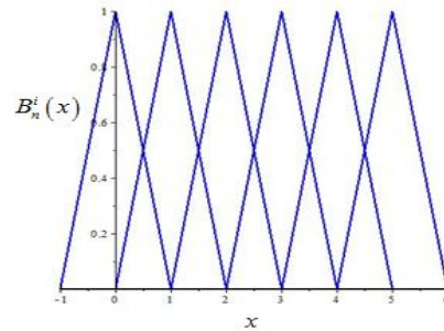
Рис.6. Система базисных функций B_1^i(x), i = \overline{-1, 4} .
