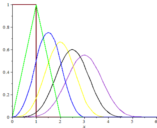
Рис. 3. Сплайны K_1, K_2, K_3, K_4, K_5 .
