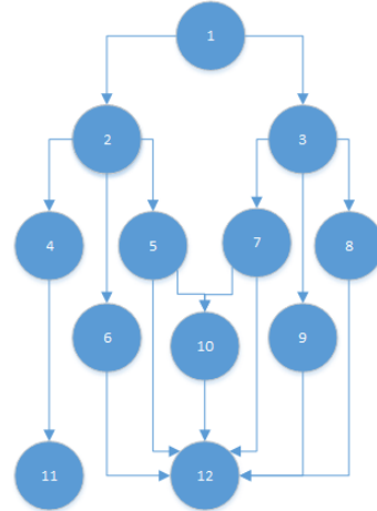
Рис. 1. Схема вычислений
