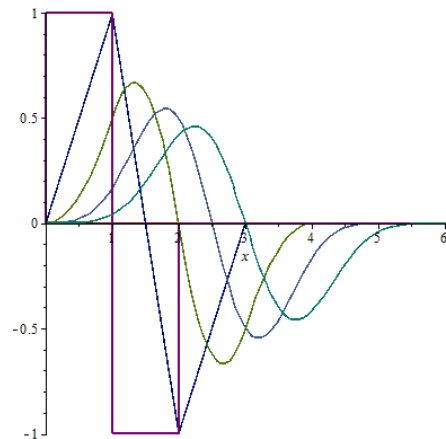
Рис.4. Производные сплайнов K_1, K_2, K_3, K_4, K_5 .
