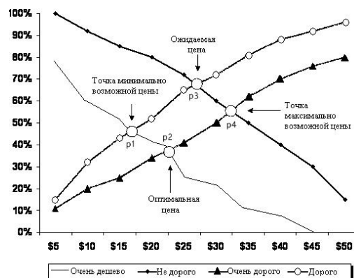
Рис.1. Метод PSM
