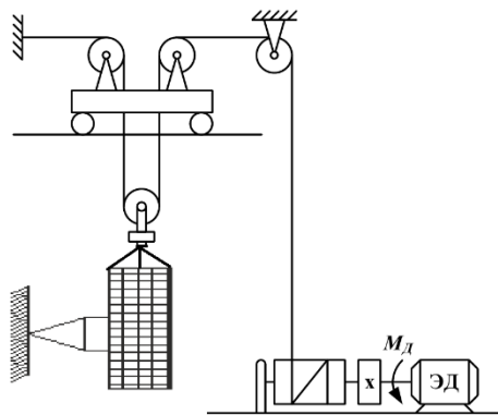
Рис. 1. Пример активной системы обезвешивания
