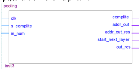
Рис. 4 Модуль слоя субдискретизации
