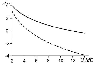
Рис. 2. Зависимость относительной координаты границы эмиссии от отношения U_d/dE ; 1 – r_0 = 0,15 мм; 2 – 0,3 мм
