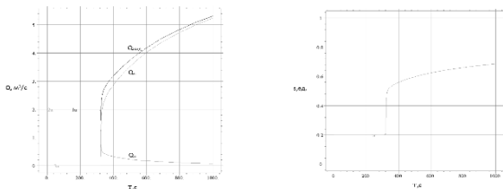
Рис. 1. Дебит и обводненность продукции на добывающей скважине при закачке воды
