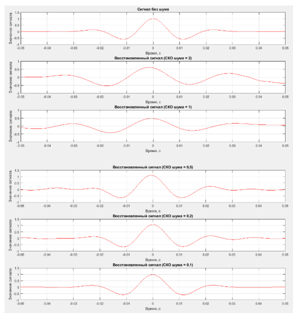
Рис. 3. Восстановленные сигналы
