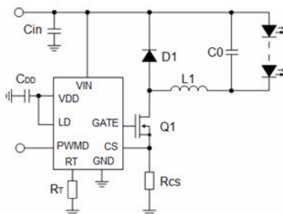
Рис. 1. Схема включения микросхемы HV9910
