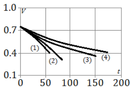
Рис. Изменение объема пластинки, подверженной одностороннему коррозионному износу с течением времени.
