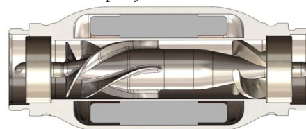
Рисунок 2 – Трехмерная твердотельная модель насоса АВК-Н "Спутник"
