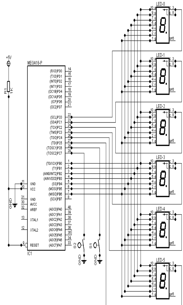
Рис. 6 схема часов
