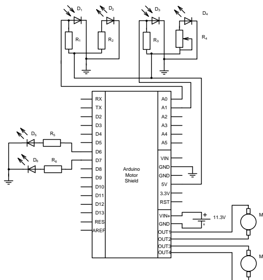
Рис. 1. Принципиальная схема колесного робота
