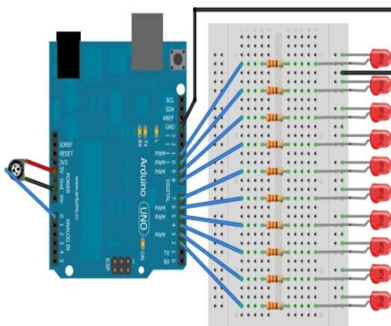
Рис.2. Иллюстрация проекта, выполненного в программе Fritzing.
