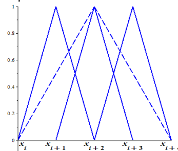
Рис.2 Сплайны с носителем 2h и 4h .
