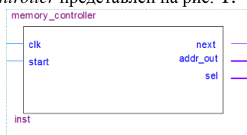
Рис. 1 Модуль memory_controller
