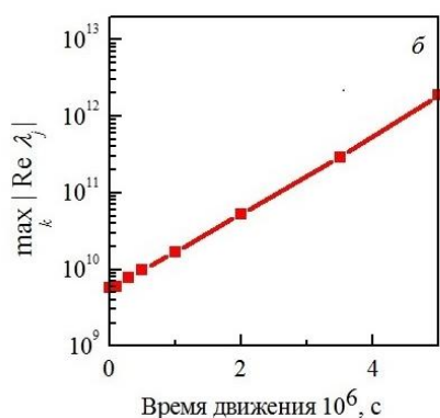
Рис. 2. Изменение на интервале интегрирования для задачи Коши [2-5] значение \max_k |\operatorname{Re} \lambda_j|
