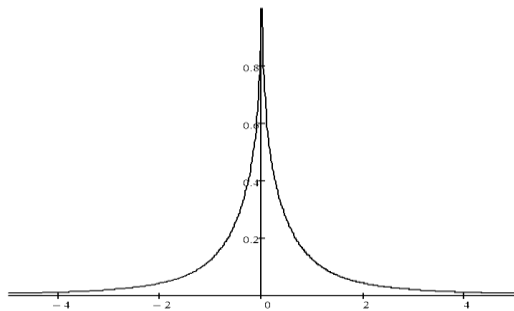
Рис. 1. График функции плотности (4)
