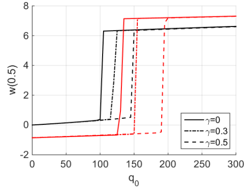
Рис. 5. w(0.5)[q_0]
