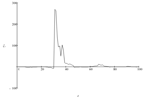
Рис. 2. График значений \xi_t при n = 100
