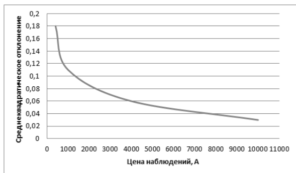
Рис. 1. Изменение среднеквадратического отклонения. Последовательное оценивание.
