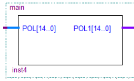
Рис. 4. Модуль main
