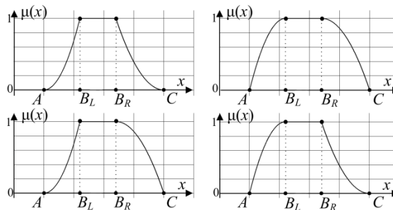
Рис. 1. Возможные формы полиномиальной ФП 2-го порядка
