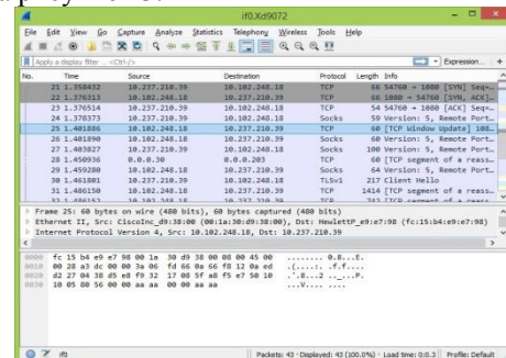
Рис. 13 Скриншот из программы Wireshark
