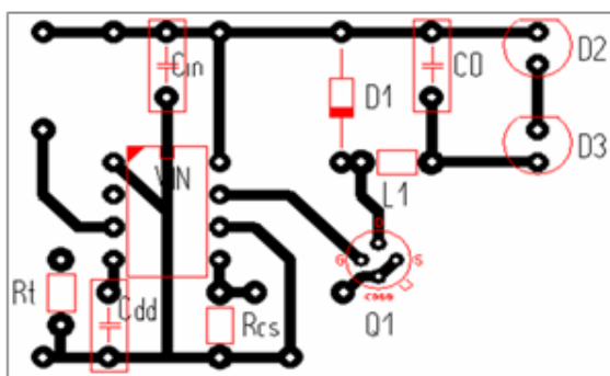
Рис. 2. Внешний вид печатной платы
