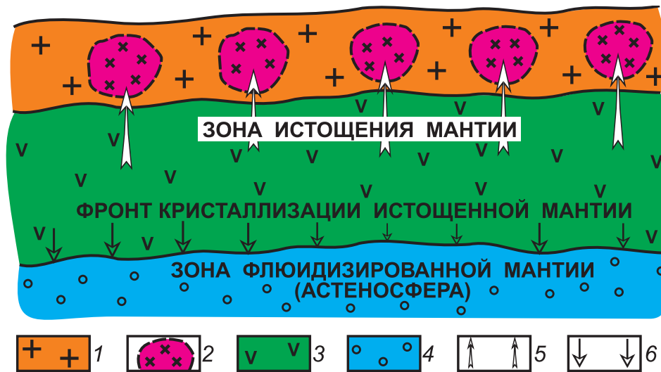
Рисунок. Модель формирования континентальной литосферы: 1) гранитогнейсовая кора; 2) гранитогнейсовые купола; 3) истощенная мантия; 4) флюидизированная мантия (астеносфера); 5) направление восходящих потоков флюидных и гранитизирующих компонентов; 6) направление нисходящих перед фронтом кристаллизации флюидных и сверхстехиометрических компонентов
