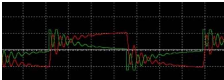
Рис. 8 Формы сигнала на выходе ОУ (красная кривая) и сумматора (зеленая кривая), полученные в Multisim. Масштаб: X – 20 мс/дел, Y – 10В/дел.
