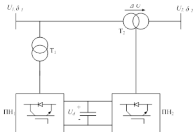
Рисунок 3 – Схема объединённого регулятора потоков мощности
