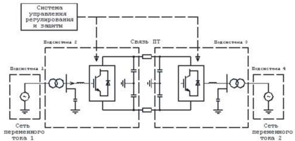
Рисунок 2 – Осуществление межсистемной связи с применением ВПТ
