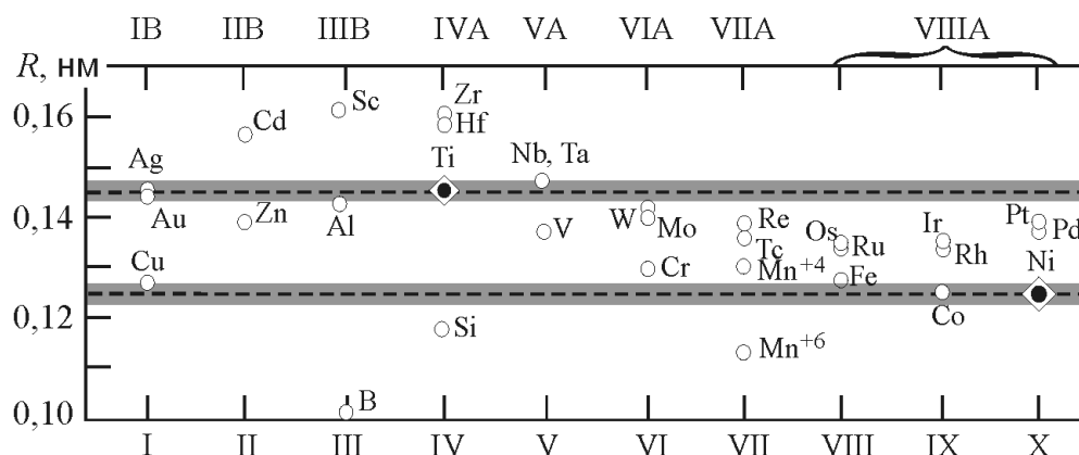
Рис. 1. Диаграмма распределения размеров атомов основных сплавообразующих элементов Ti и Ni относительно легирующих элементов в зависимости от положения в Периодической системе (IB-VIIIA). Верхняя шкала отражает нумерацию групп в Периодической системе элементов по рекомендации ИЮПАК (1989)
