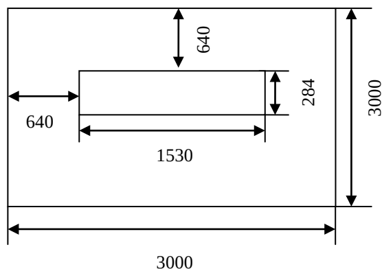
Рисунок 7 – Расположение светильника в кабинете
