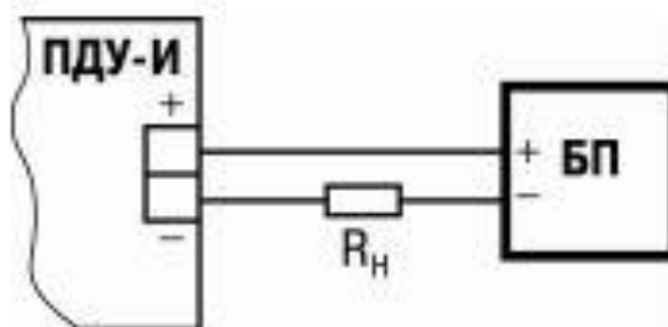
Рисунок 20 –схема подключения датчика ПДУ-И ОВЕН
