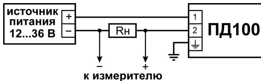
Рисунок 14 – Схемы подключения ОВЕН ПД100-ДИ115
