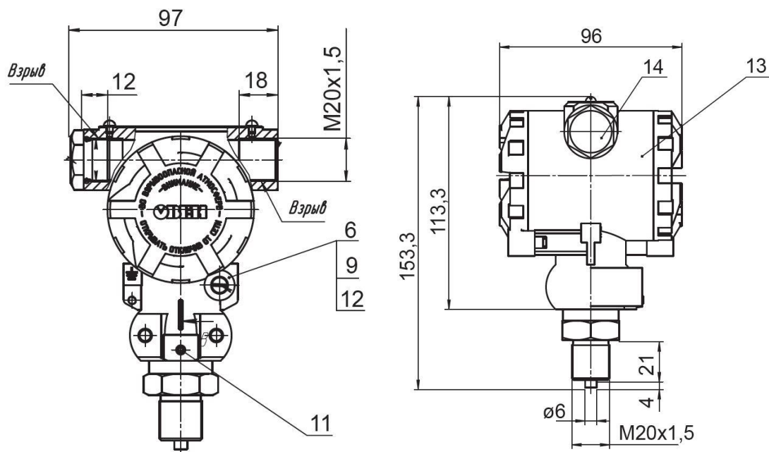
Рисунок 13 – Установочно присоединительные размеры
