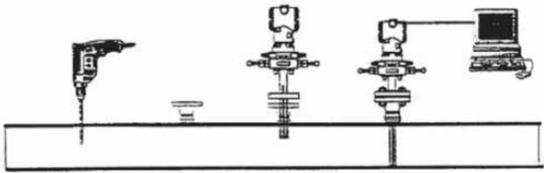
Рисунок 7 – Монтаж расходомера Метра-350
