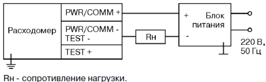
Рисунок 10 – Схема подключения Расходомера Метран-350 к источнику Необходимо так же заказать закладную конструкцию для крепления к трубопроводу (рисунок 11):
