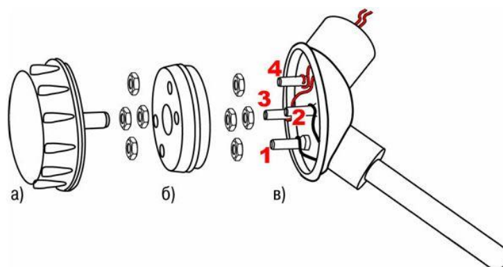
Рисунок 17 – схемы подключения датчика ДТП.И ОВЕН
