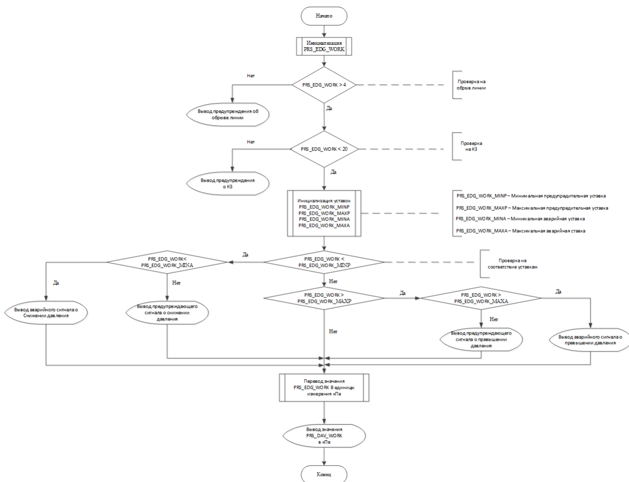
Рисунок 26 – Алгоритм сбора данных
