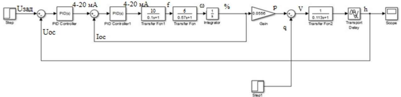
Рисунок 28 – Модель САР
