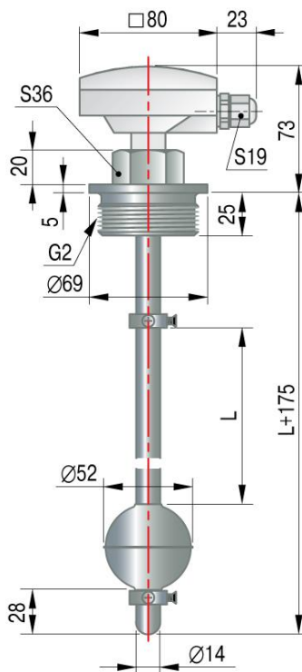
Рисунок 19 –габаритно установочные размеры ПДУ-И ОВЕН
