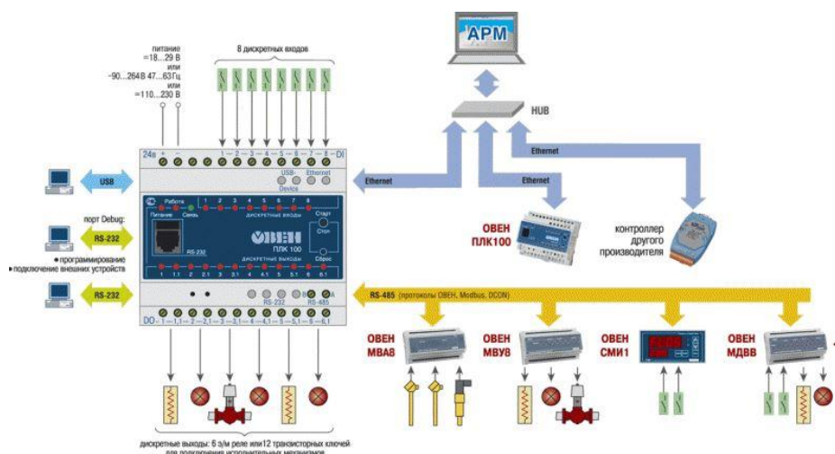
Рисунок 5 – возможная работа контроллера ОВЕН ПЛК 100
