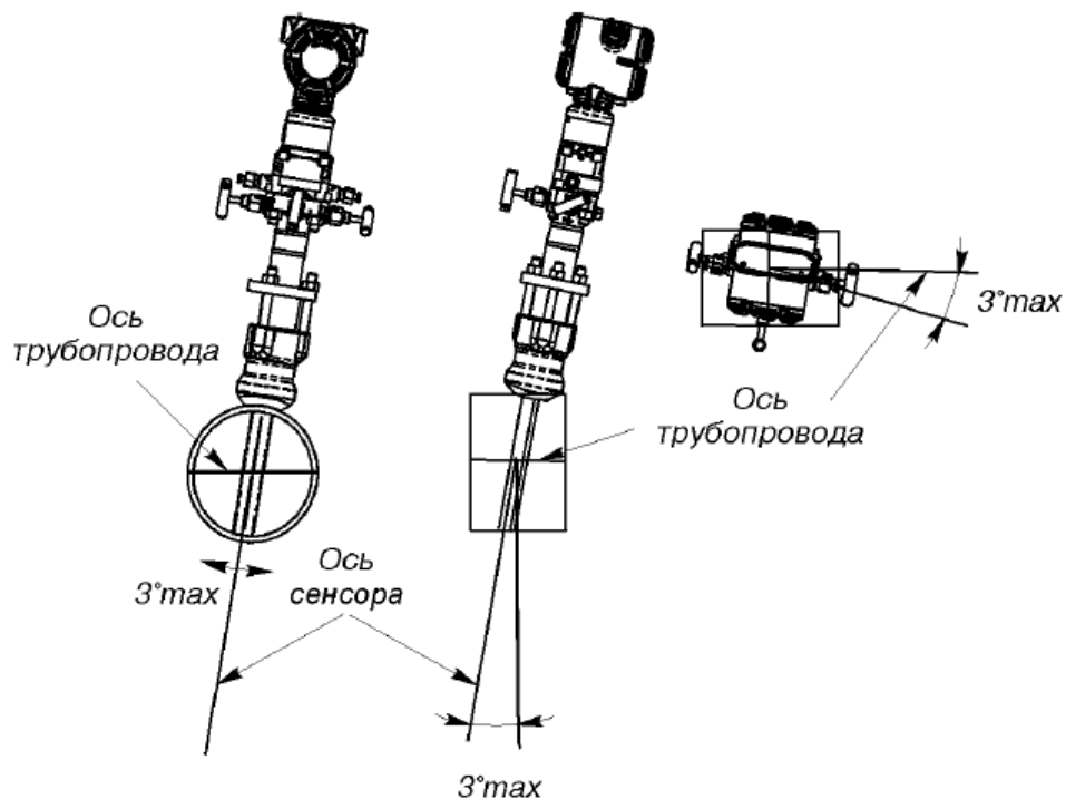
Рисунок 9 – допускаемые отклонения ориентации расходомера Метран-350 Схема подключения к источнику питания приведена на рисунке 10:
