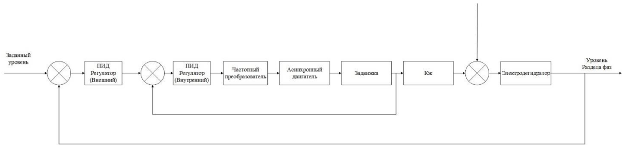
Рисунок 27 –функциональная схема САР
