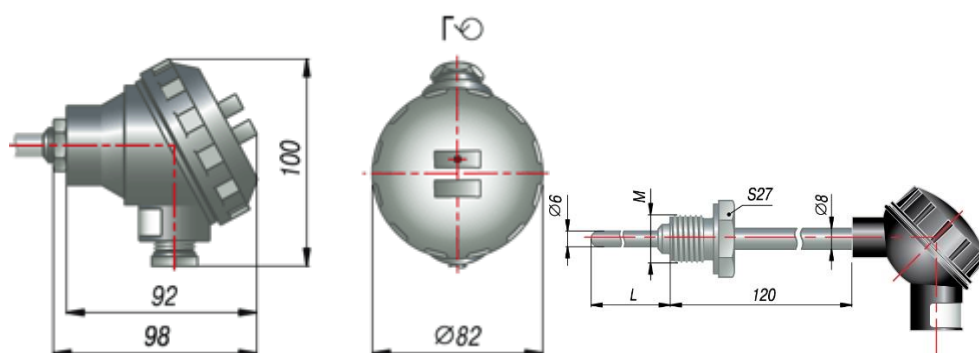
Рисунок 16 – Габаритные размеры датчика ДТП.И ОВЕН
