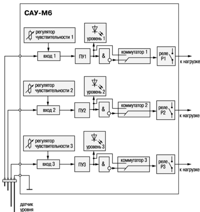
Рисунок 23 – Функциональная схема прибора САУ-М6
