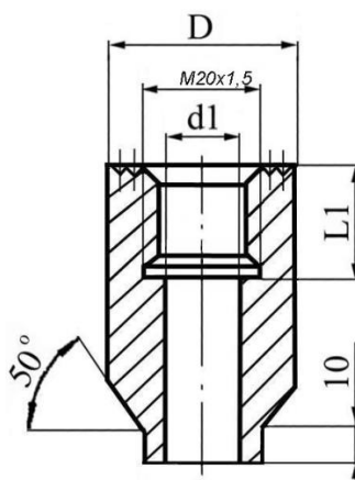
Рисунок 11 – крепление к трубопроводу
