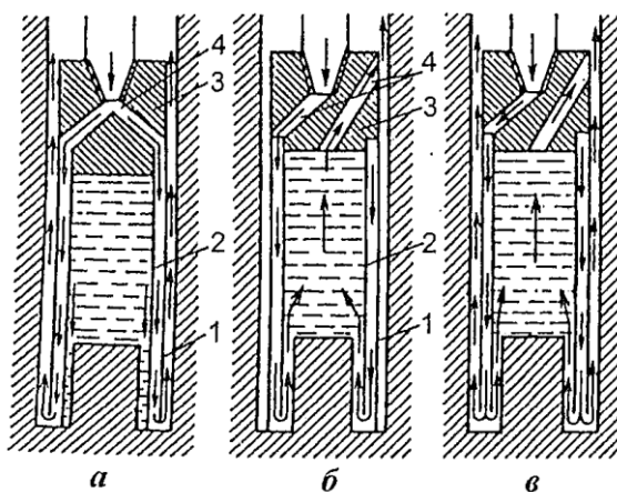
Рисунок 5.1 – Схемы циркуляции очистного агента в ДКС:
