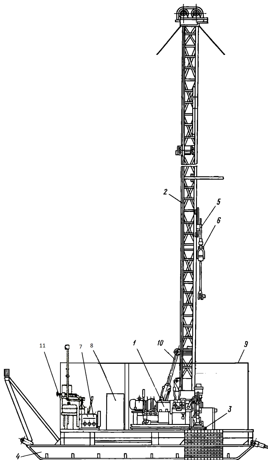
Рисунок 2.3 – Передвижная буровая установка УКБ-200/300: 1 – буровой станок; 2 – мачта; 3 – труборазворот; 4 – санное основание; 5 – каретка; 6 – полуавтоматический элеватор; 7 – буровой насос; 8 – электрический шкаф; 9 – укрытие; 10 – гидроцилиндр; 11 – дизель-генератор
