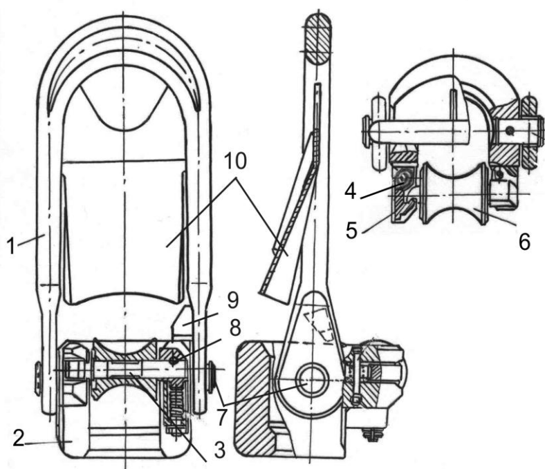
Рисунок 2.8 – Полуавтоматический элеватор МЗ-50-80:
