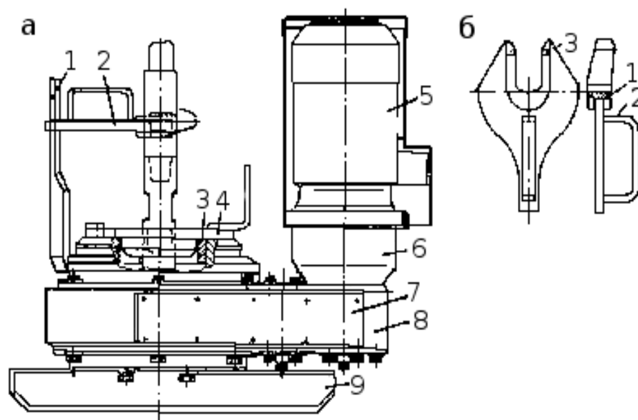
Рисунок 2.7 – Схема трубопозвора РТ-1200М:
