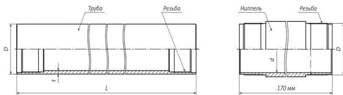
Рисунок 2.5 – Обсадные трубы ниппельного соединения
