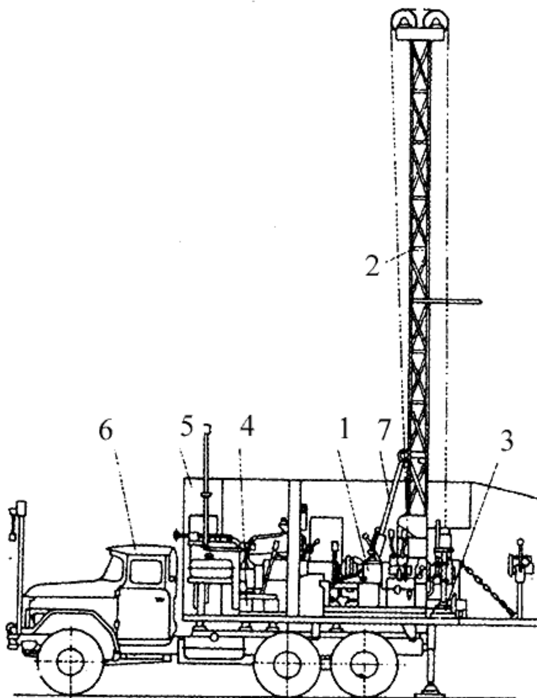
Рисунок 2.2 – Самоходные буровая установка УКБ-200/300С: 1 – буровой станок; 2 – мачта; 3 – труборазворот; 4 – буровой насос; 5 – укрытие; 6 – кабина; 7 – гидроцилиндр
