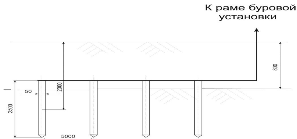
Рисунок 3.1 – Развернутый вид заземляющего контура в грунте
