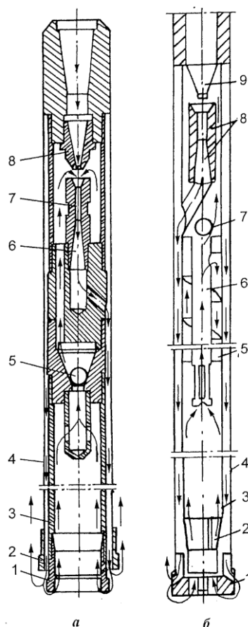
Рисунок 5.4 – Двойные колонковые эжекторные снаряды:
