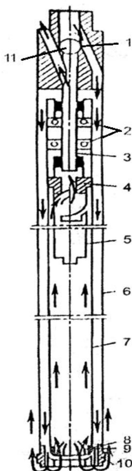
Рисунок 2.6 – Схема ДКС с не вращающимся керноприемником ДКНТ-ВП-0:
