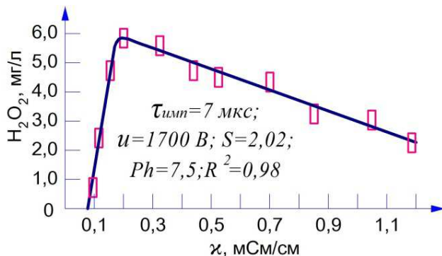
Рис. 8. Выход H_2O_2 в зависимости от проводимости модельного раствора
