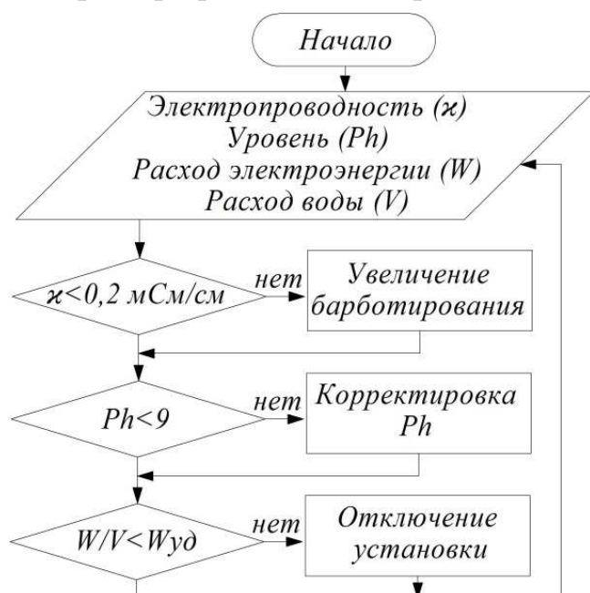
Рис. 15. Алгоритм управления системой дезинфекции воды
