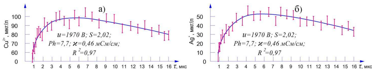
Рис. 10. Образование ионов \text{Cu}^{2+} (а) и \text{Ag}^+ (б) в зависимости от длительности импульсов напряжения
