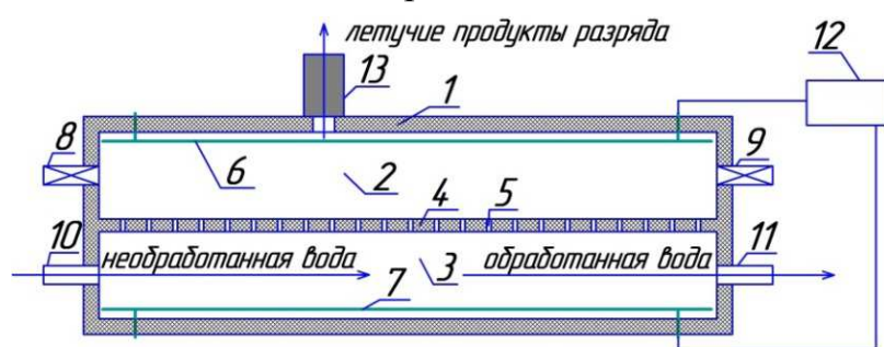
Рис. 1. Схема реактора ДЭР
