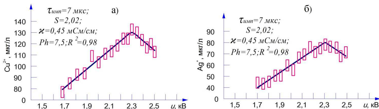
Рис. 9. Выход ионов меди (а) и серебра (б) в зависимости от мгновенного импульсного напряжения
