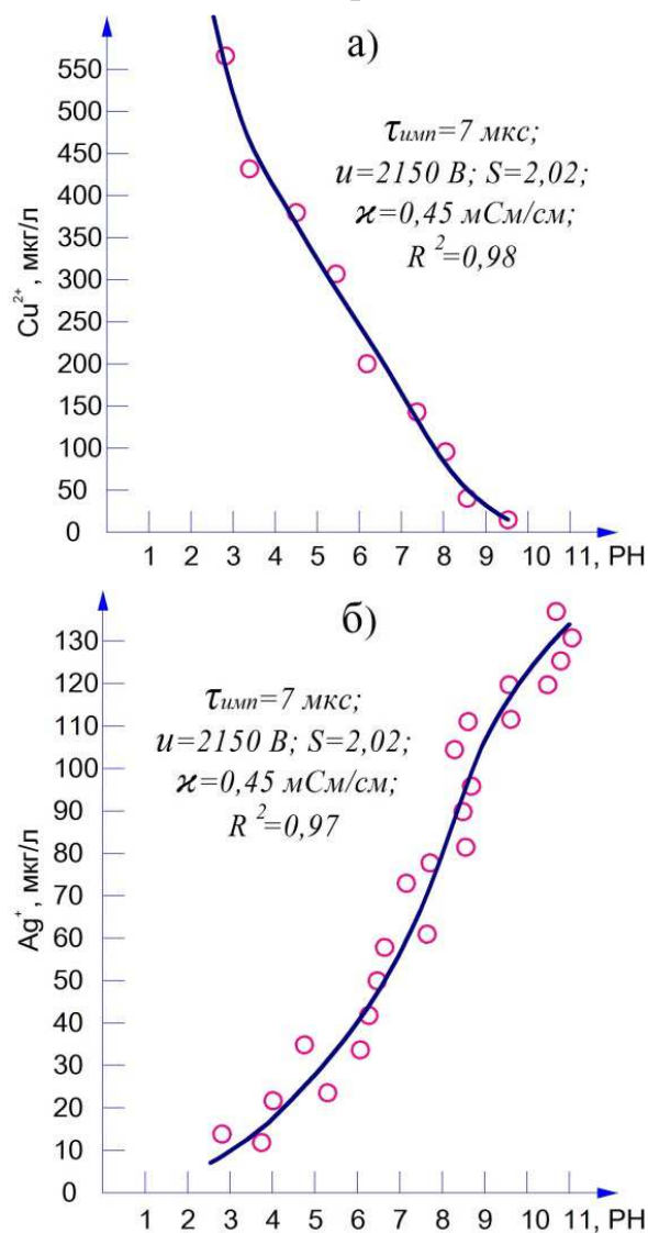
Рис. 12. Образование \text{Cu}^{2+} (а) и \text{Ag}^+ (б) от РН модельного раствора
