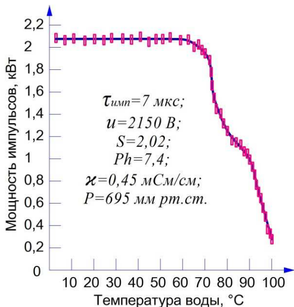
Рис. 5. Потребляемая мощность реактора ДЭР в зависимости от температуры воды
