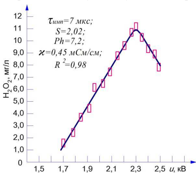
Рис. 6. Выход перекиси водорода в зависимости от амплитуды импульсного напряжения
