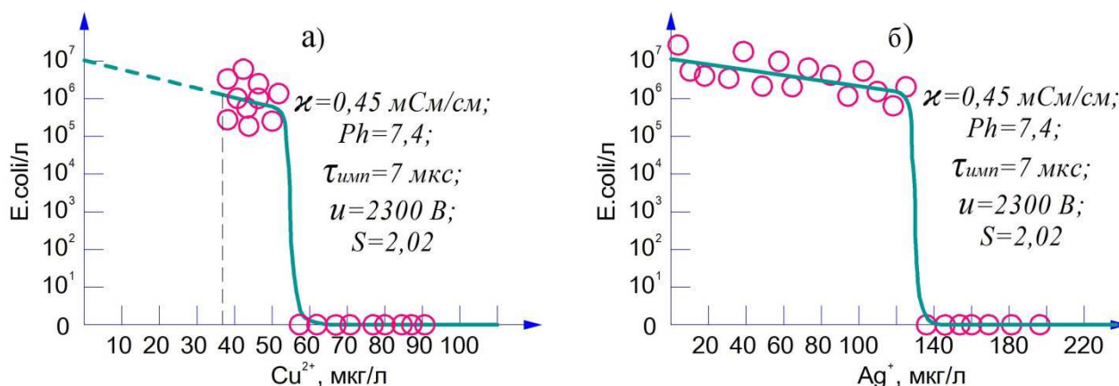
Рис. 14. Зависимости отмирания E. coli от концентрации \text{Cu}^{2+} (а) и \text{Ag}^+ (б)
