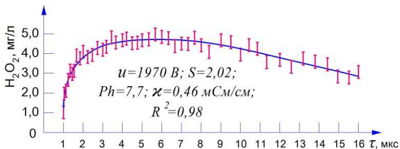
Рис. 7. Зависимость генерирования перекиси водорода H_2O_2 от длительности импульсов напряжения
