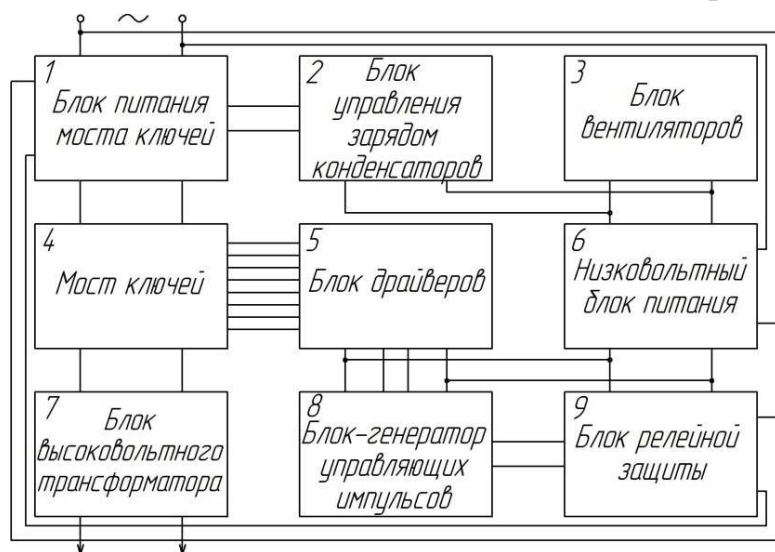
Рис. 2. Блок - схема ВИИП
