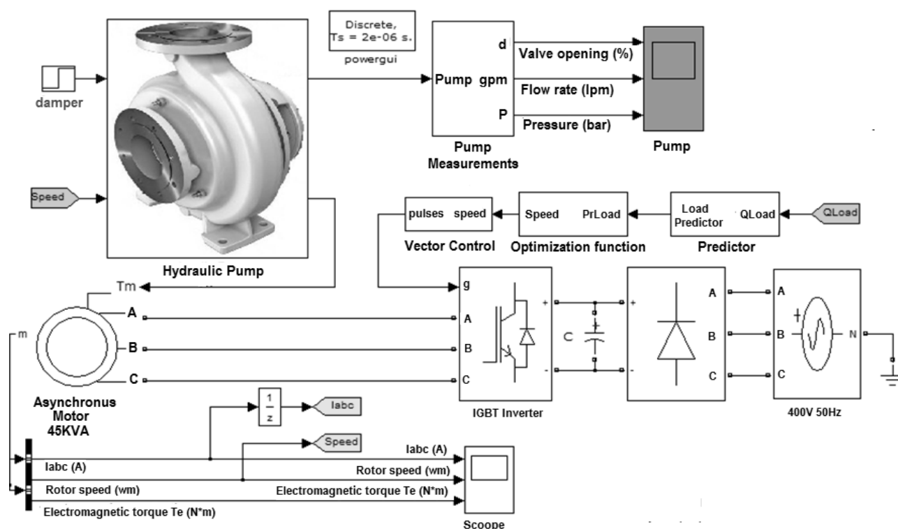
Рисунок 9 – Имитационная модель насосного агрегата с прогнозной оптимизацией
