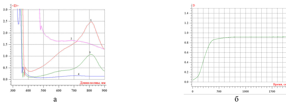
Рис. 1. (а) Оптические свойства синей формы КМК, полученной при действии различных восстановителей: 1 – N_2H_6SO_4 , 2 – SnCl_2 , 3 – C_6H_8O_6 , 4 – Na_2SO_3 ; (б) кинетика образования синего комплекса
