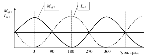
Рис. 6. Кривые изменения взаимной индуктивности обмотки якоря и обмотки возбуждения M_{af1} и изменения собственной индуктивности обмотки якоря L_{a1} в зависимости от угла поворота ротора \gamma
