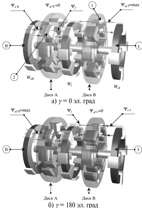
Рис. 5. Принцип действия многополюсного коммутаторного генератора
