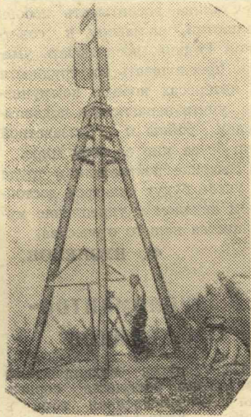
Наблюдение вертикальных углов на точке «Мысовая».
