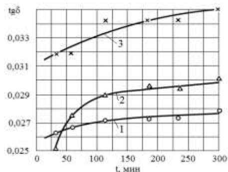
Рисунок 5 - Изменение тангенса угла диэлектрических потерь в процессе твердения цементной суспензии при различном содержании диабаза и известняка: 1 – 2 мас.% диабаза; 2 – 7 мас. % диабаза; 3 – 9 мас.% известняка
