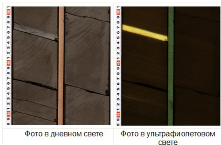
Рис. 1. Прослои в породах баженовской свиты с anomalно люминесцирующим свечением в ультрафиолетовом свете
