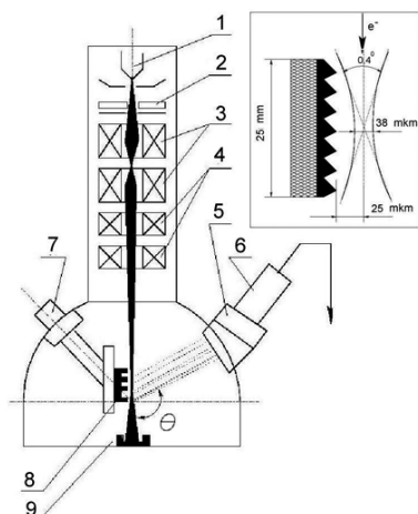
Рис. 2. Экспериментальная установка: 1) катод; 2) анод; 3) конденсоры; 4) система перемещения; 5) монохроматор; 6) ФЭУ; 7) микроинт; 8) решетка; 9) цилиндр Фарадея
