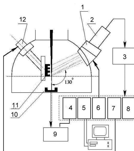
Рис. 8. Схема эксперимента: 1) монохроматор; 2) ФЭУ; 3) усилитель; 4) аналого-цифровой преобразователь; 5) контроллер; 6, 7) блоки управления двигателем; 8) счетчик; 9) усилитель; 10) цилиндр Фарадея; 11) решетка; 12) микровинт
