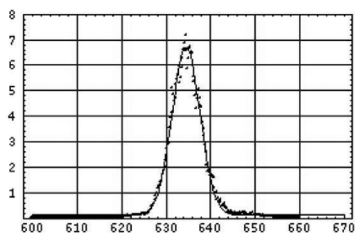
Рис. 7. Спектр лазерного излучения, полученного при помощи монохроматора
