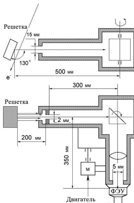
Рис. 6. Монохроматор
