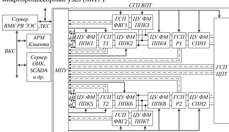
Рисунок 2 – Структурная схема СГП ВПТ
