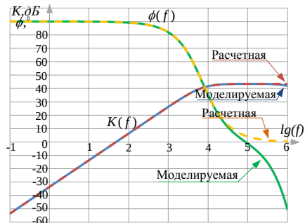
Рисунок 9 – Логарифмические амплитудно- частотные (ЛАЧХ) и фазо-частотные характеристики (ЛФЧХ) модели КБ ЦПТ при C_{KB} = 2240 \text{ мкФ} и R_{KB} = 0,01 \text{ Ом}
