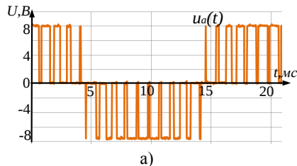
Рисунок 12 – Осциллограммы фазного (а) и линейного (б) напряжений на выходе ЦУ ФМ СПН на базе ЦУАК, функционирующего в режиме инвертора
