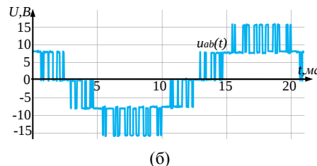
Рисунок 12 – Осциллограммы фазного (а) и линейного (б) напряжений на выходе ЦУ ФМ СПН на базе ЦУАК, функционирующего в режиме инвертора
