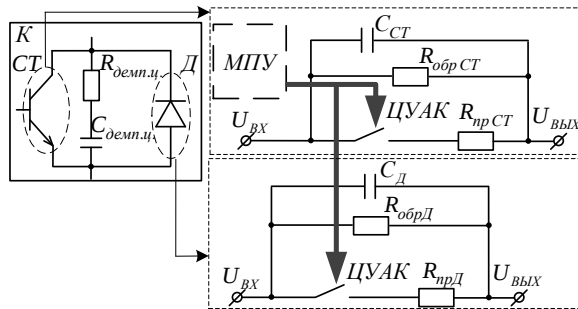
Рисунок 5 – ЦУ ФМ быстродействующего полностью управляемого полупроводникового i -го ключа ( K_i ), содержащая модели силового транзистора (СТ) (а) и обратного диода (Д) (б), а также демпфирующей цепи ( R_{\text{дем.ц.}}, C_{\text{дем.ц.}} )
