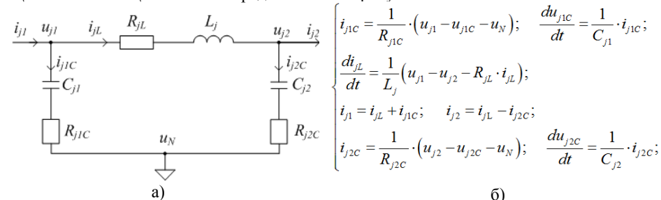
Рисунок 3 – Схема замещения (а) и система уравнений всережимной математической модели j-го полюса ЦПТ (б), где j – отрицательный или положительный полюс; R_{jL} и L_j – активное сопротивление и индуктивность сглаживающего реактора (СР) j-го полюса; R_{j1C} , R_{j2C} и C_{j1} , C_{j2} – активные сопротивления и емкости конденсаторных батарей (КБ) j-го полюса; u_{j1C} , u_{j2C} – напряжения на реактивных сопротивлениях конденсаторных батарей j-го полюса ЦПТ; u_N – напряжение нейтрали.
