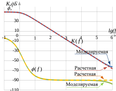
Рисунок 10 – ЛАЧХ и ЛФЧХ модели СР ЦПТ при L_{CP} = 500 \text{ мкГн} и R_{CP} = 4,9 \text{ мОм}
