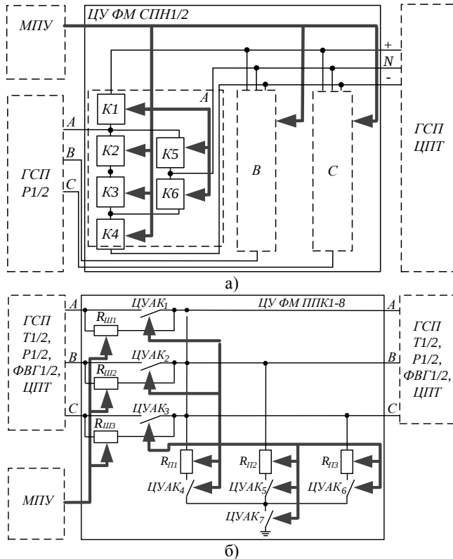
Рисунок 6 – Структурные схемы ЦУ ФМ СПН (а) и ЦУ ФМ ППК (б), где R_{\text{ш1-3}} – цифруемые сопротивления, позволяющие учитывать сопротивление шунтов выключателя; R_{\text{п1-3}} – цифруемые сопротивления, используемые для учета переходных сопротивлений КЗ
