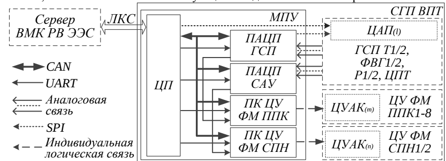
Рисунок 7 – Структурная схема МПУ СГП ВПТ, где шина CAN предназначена для широкополосных взаимодействий между процессорами МПУ, UART – для индивидуального взаимодействия между процессорами МПУ, SPI – для управления параметрами моделируемого оборудования, задаваемыми в ЦАП ГСП, ЛКС – информационно-управляющего взаимодействия ЦП с Сервером ВМК РВ ЭЭС
