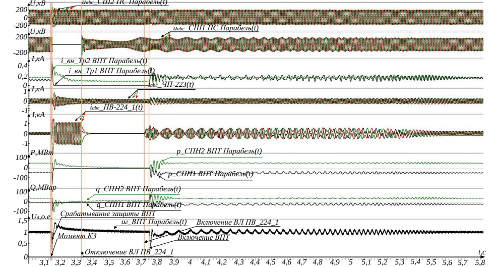
Рисунок 19 – Осциллограммы токов, напряжений и мощности при трехфазном КЗ на ВЛ ЧП_223 (ПС Каргасок – ПС Парabelь) с ВПТ
