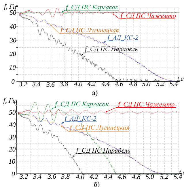
Рисунок 20 – Осциллограммы изменения частот вращений синхронных и асинхронных двигателей при трехфазном КЗ на ВЛ ЧП_223 (ПС Кargasок – ПС Парабель) с ВПТ (а) и без ВПТ (б)
