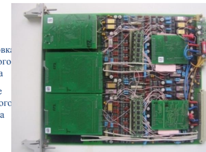
Рисунок 15 – Внешний вид СГП ВПТ
