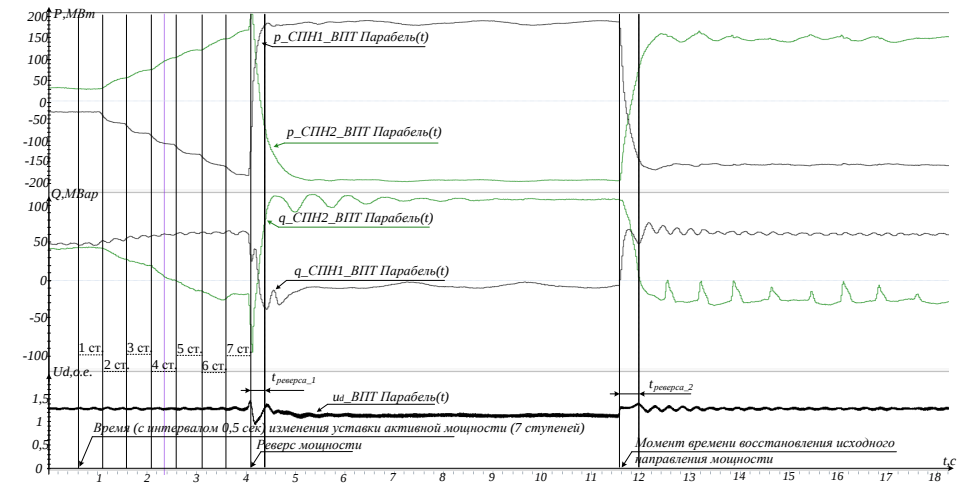
Рисунок 18 – Процессы регулирования перетока мощности через ВПТ
