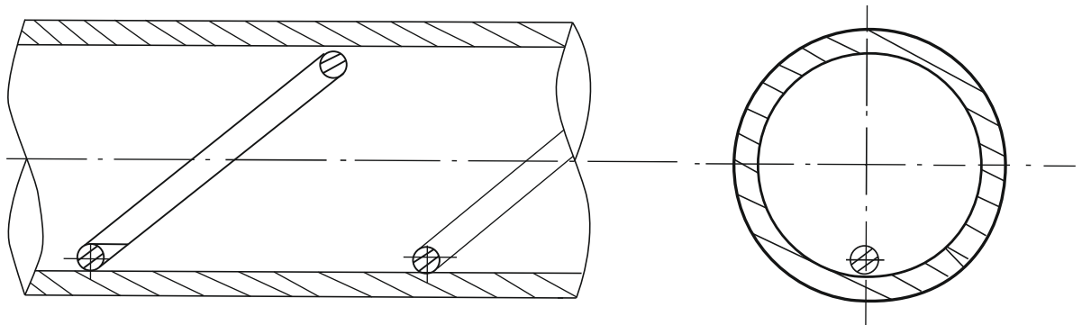
Рисунок 1.6 – Труба со спирально-винтовой проволочной вставкой.
