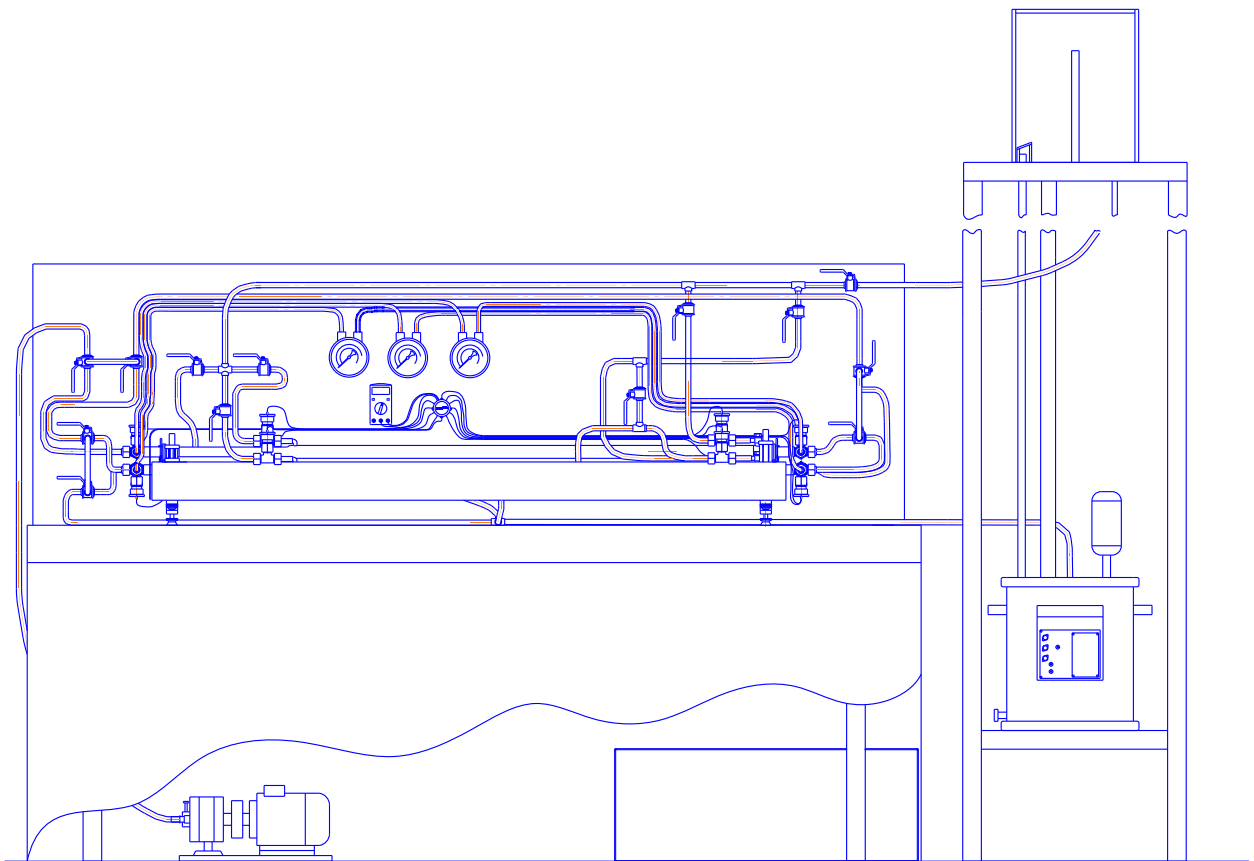
Рисунок 4.3 – Экспериментальная установка
