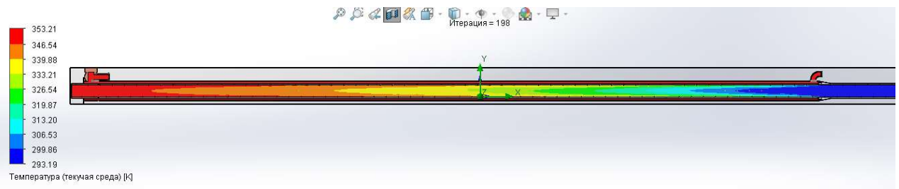
Рисунок 4.5 – Распределение температур теплоносителей по сечению рабочего участка при наличии винтовой проволочной вставки
