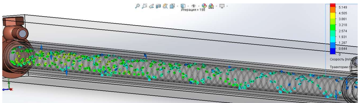
Рисунок 4.6 – Пространственное распределение скорости холодного теплоносителя по длине рабочего участка при наличии винтовой проволочной вставки
