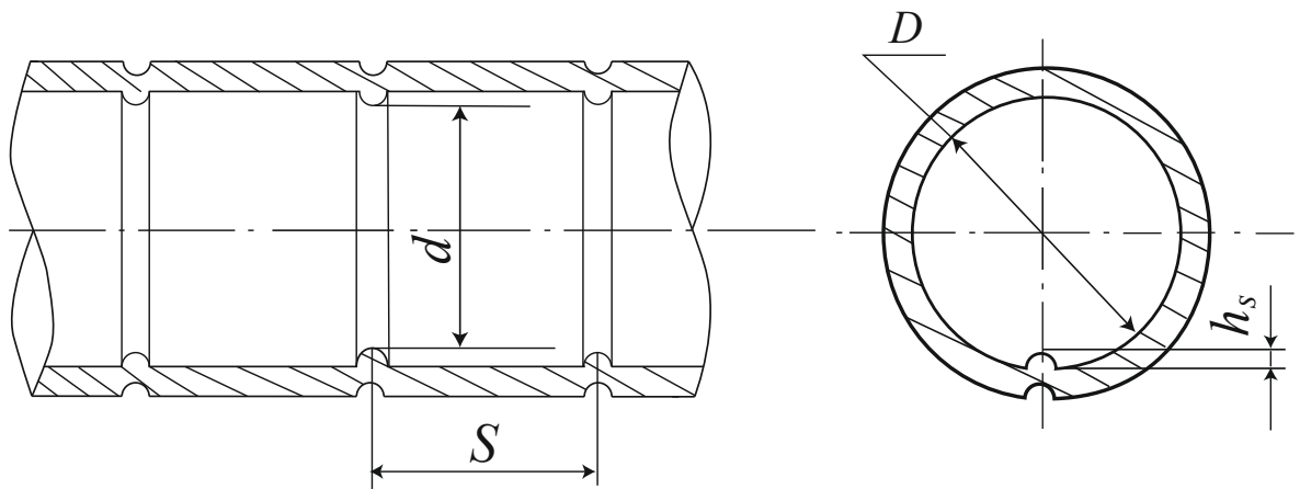
Рисунок 1.7 – Поперечно-кольцевая накатка.
