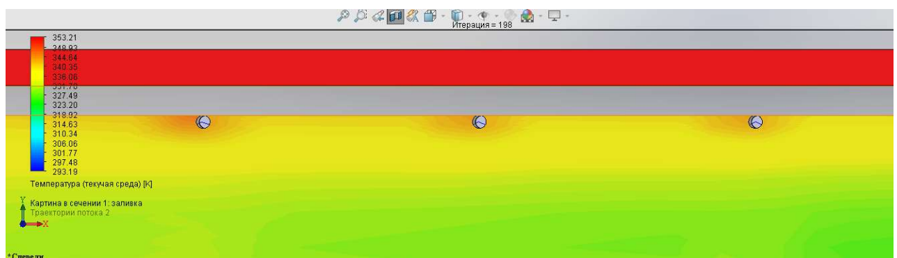
Рисунок 4.7 – Распределение температур вблизи винтовой проволочной вставки
