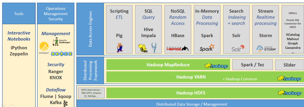
Рис. 1. Экосистема Hadoop [2]
