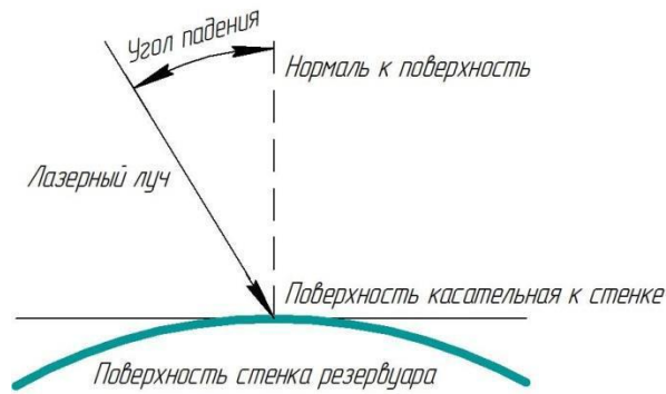
Рисунок 2.7 – Угол падения лазерного луча на поверхность
