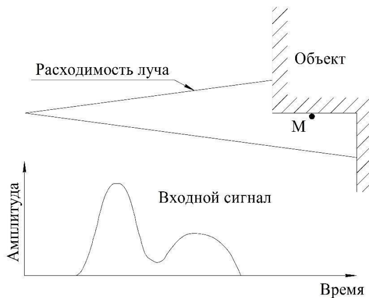
Рисунок 2.6 – Форма входного сигнала при попадании лазерного луча на границу
