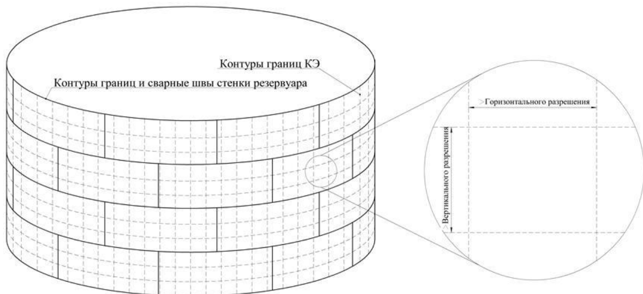
Рисунок 3.4 – Схема аппроксимации поверхности стенки резервуара конечными элементами
