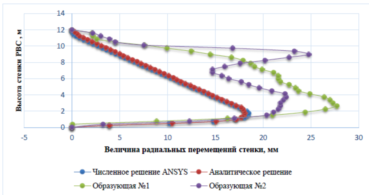
Рисунок 3.10 – Перемещения стенки в радиальном направлении
