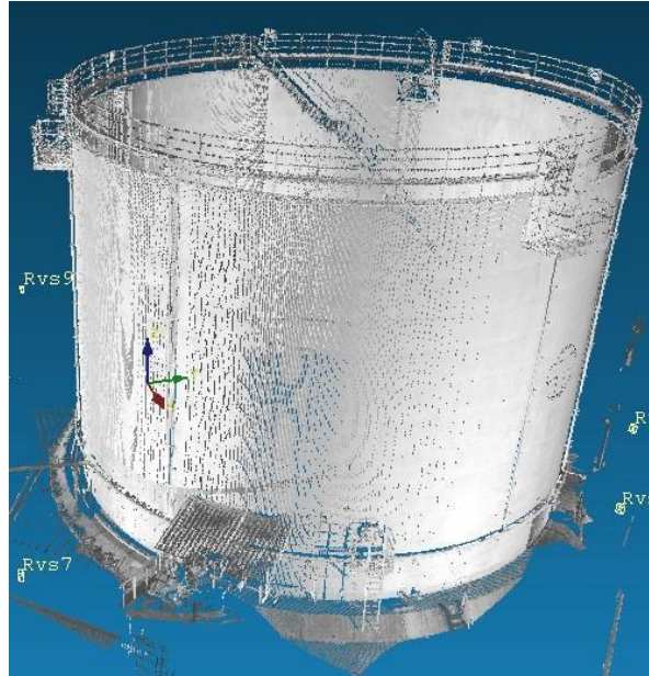
Рисунок 2.10 – Единая трехмерная точечная модель резервуара РВСП-7500
