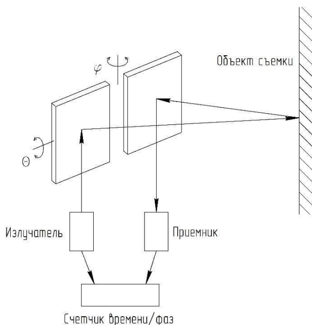
Рисунок 2.1 – Принципиальная схема работы НЛС
