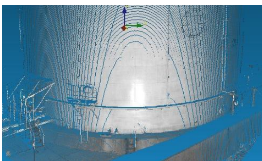
Рисунок 2.3 – Трехмерное представление результатов НЛС (облако точек)
