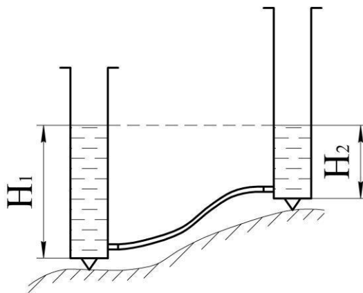
Рисунок 1.4 – Гидростатическое нивелирование
