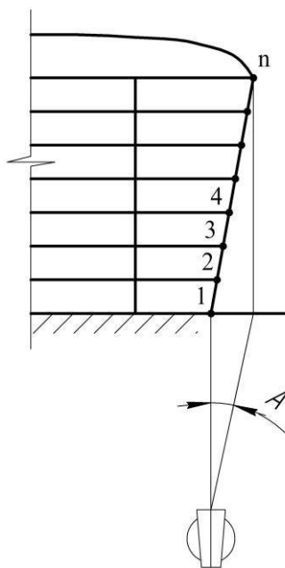
Рисунок 1.5 – Схема измерения горизонтальных смещений образующей стенки резервуара
