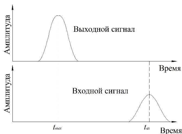
Рисунок 2.5 – Время распространения импульса в пространстве
