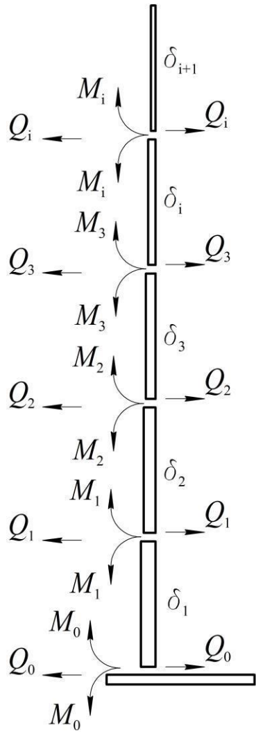
Рисунок 3.7 – Расчетная схема стенки резервуара с переменной толщиной поясов
