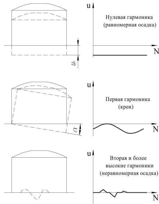
Рисунок 3.1 – Разложение осадки на гармоники
