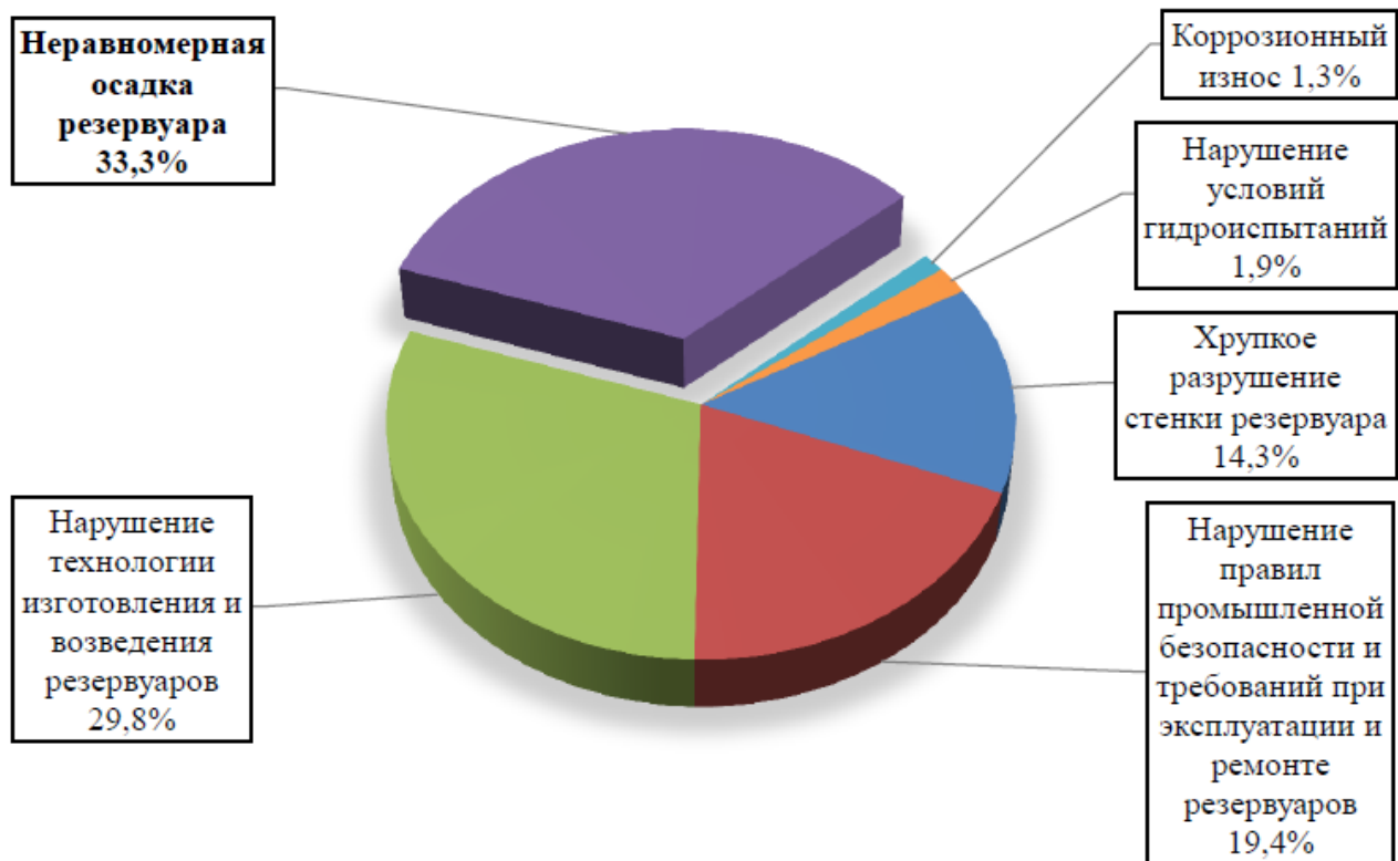
Рисунок 1.3 – Основные причины разрушения РВС
