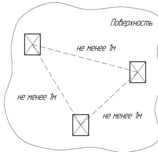
Рисунок 2.8 – Схема размещения плоских марок на поверхности стенки
