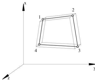
Рисунок 3.3 – Четырехузловой четырехугольный плоский КЭ
