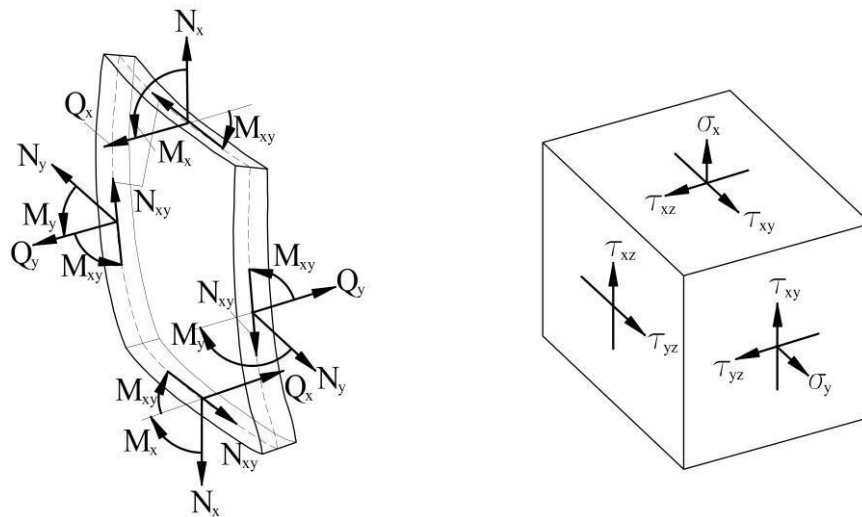
Рисунок 3.2 – Схема внутренних сил и напряжений в оболочке с учетом влияния поперечного сдвига
