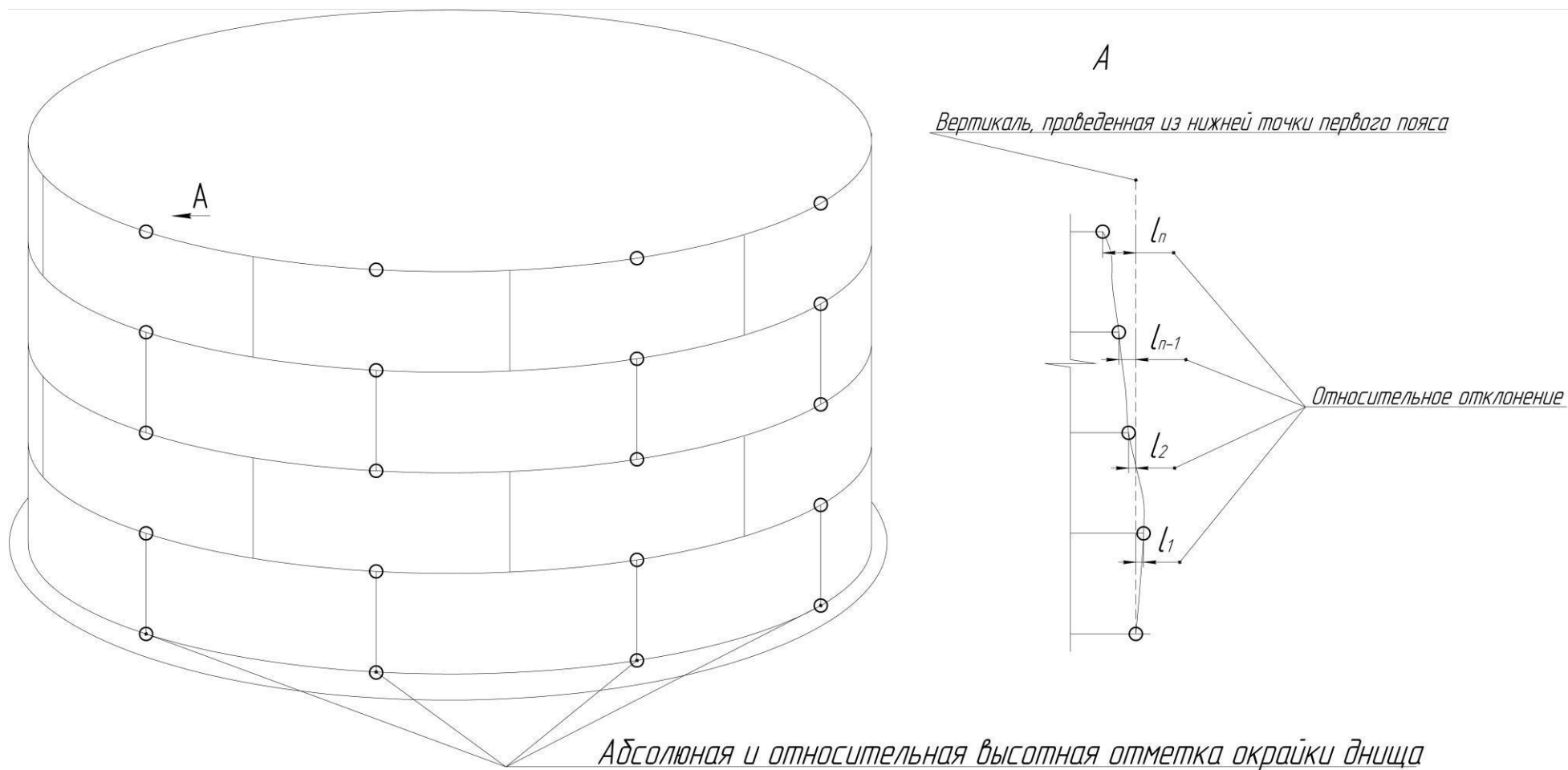
Рисунок 1.6 – Информация о пространственном положении и геометрической форме резервуара, получаемая при геодезическом обследовании
