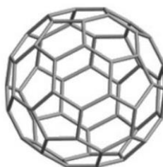
Рисунок 9 – Структура молекулы фуллерена C_{60}
