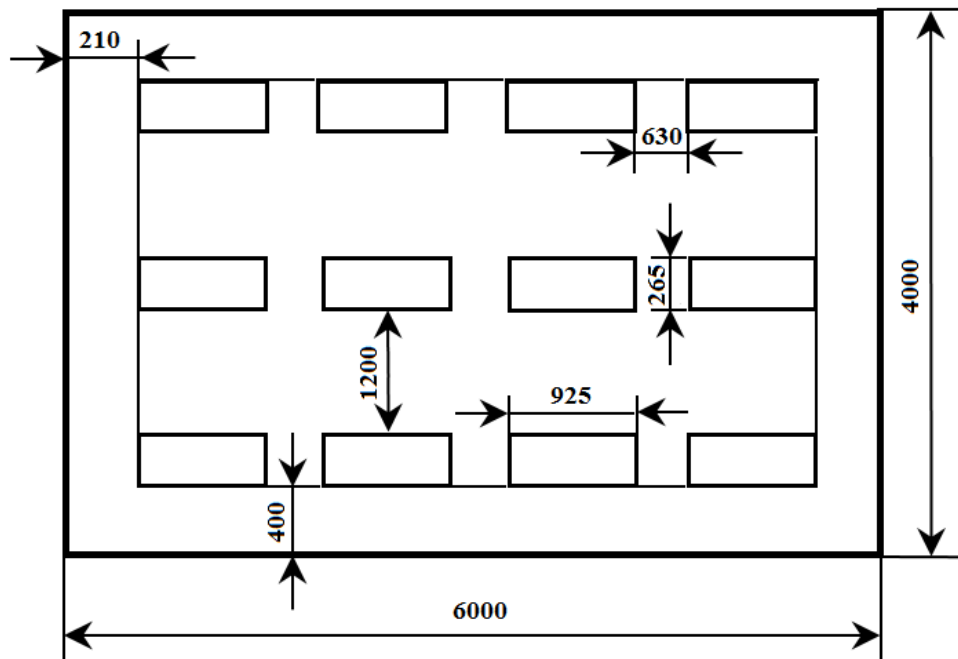
Рисунок 14 – План размещения светильников с люминесцентными лампами (размеры указаны в мм)
