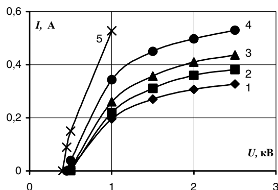
Рис. 4. ВАХ ионного источника при различных расходах газа через него: 1) 25; 2) 30; 3) 35; 4) 45; 5) 50 норм. см 3 /мин
