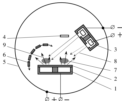
Рис. 1. Схема установки: 1) магнетрон; 2) мишень; 3) ионный источник; 4) подложка; 5) вакуумная камера; 6) положения пьезокарцевого датчика; 7) зона горения магнетронного разряда; 8) поток внешних ионов; 9) поток распыленных атомов
