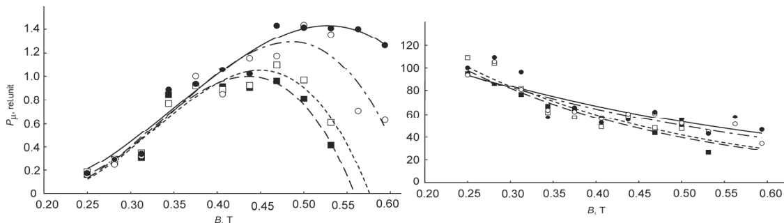
Рис. 6. Зависимости мощности (слева) и длительности (справа) СВЧ-импульса РМГ от величины индукции магнитного поля (■ — катод без экранов; □ — катод с экраном со стороны высоковольтного фланца; ○ — катод с экраном со стороны трубы дрейфа; ● — катод с двумя экранами)
