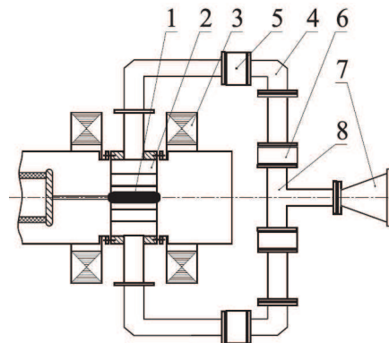
Рис. 2. Релятивистский магнетрон с волноводным каналом связи. 1 – катод; 2 – анодный блок; 3 – магнитная система; 4 – канал связи; 5, 6 – волноводные вставки; 7 – антенна
