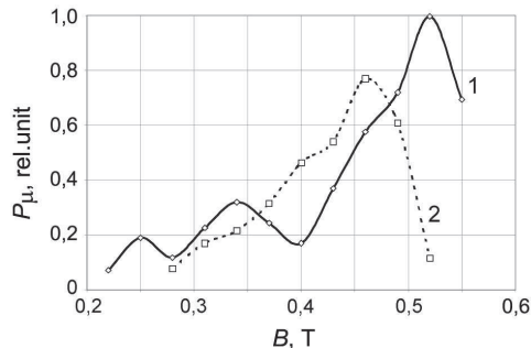
Рис. 3. Зависимость мощности 8-резонаторного РМГ от величины индукции магнитного поля с внешним каналом связи при антисимметричном включении (1) и симметричном включении (2) 3-дБ Н-тройника
