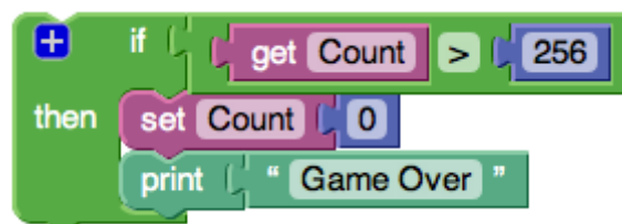
Рис. 3. Пример визуальной структуры Blockly
