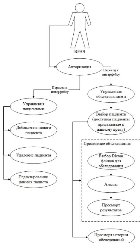
Рисунок 1 – Сценарий использования
