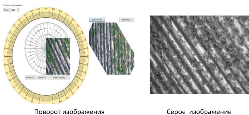
Рис. 2. Предварительная обработка
