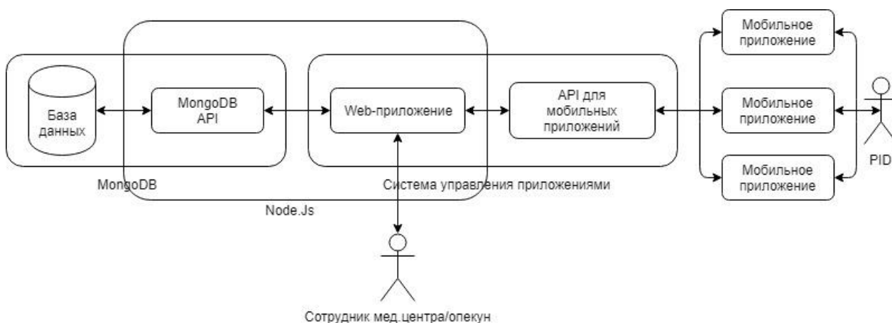
Рисунок 1 Архитектура системы
