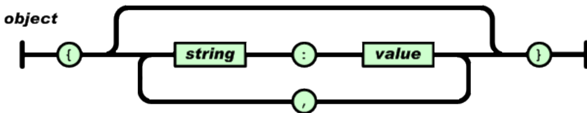
Рисунок 1. JSON Объект
