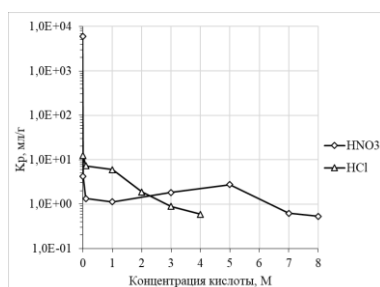
Рис.1. Зависимость коэффициентов распределения свинца от концентрации азотной и соляной кислоты для сорбента на основе ФП
