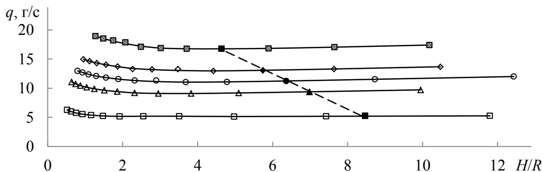
Рисунок 1. Зависимость средней производительности емкостей от отношения H/R □ – V=1,0 м 3 ; △ – V=2,0 м 3 ; ○ – V=2,5 м 3 ; ◇ – V=3,0 м 3 ; ■ – V=4,0 м 3
