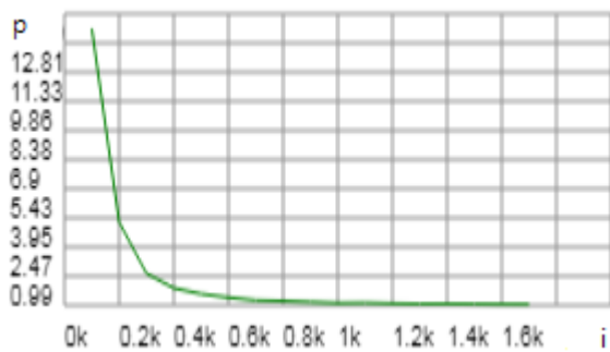
Рис. 2. График зависимости перплексии от итерации в первом эксперименте
