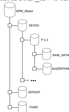
Рис. 2. Физическая структура базы данных информационной системы
