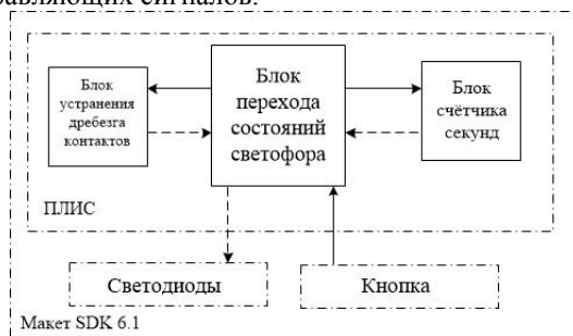
Рис. 4. Структурная схема светофора с кнопкой
