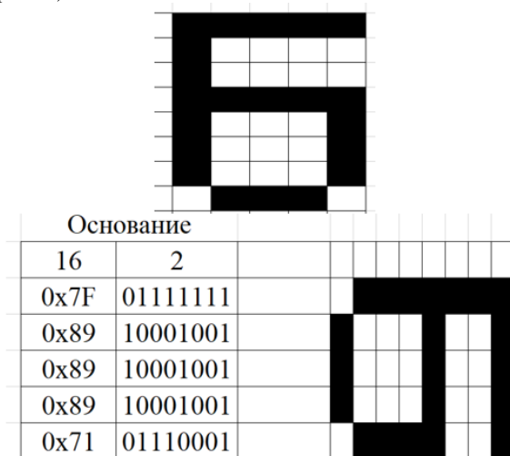
Рис. 4. Принцип создания спрайта символа
