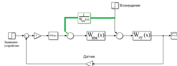
Рис. 2. Компенсация по возмущению
