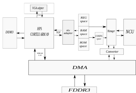
Рис. 1. Функциональная схема устройства из [1]
