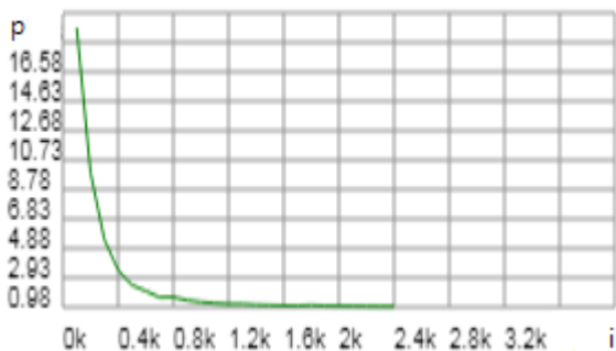
Рис. 3. График зависимости перплексии от итерации во втором эксперименте
