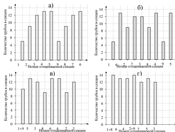
а) действующая последовательность сброса; б) сброса без совместного отпаривания; в) последовательность сброса с одним совместным отпариванием; г) последовательность сброса с двумя совместным отпариванием.
