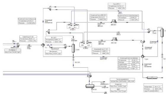
Рис. 2 Технологическая схема УОГ
