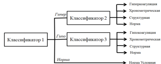
Рис. 2. Схема работы дифференциального классификатора
