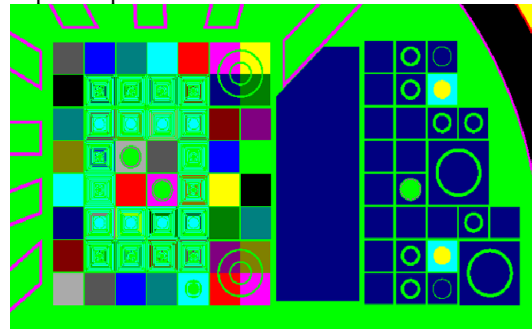
Рис. 2. Расчетная модель активной зоны реактора ИРТ-Т, созданная в MCU-PTR
