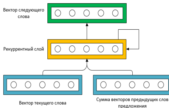
Рис. 1. Модель нейронной сети
