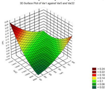
Рис. 2. График зависимости переменной Var1 от Var28 и Var30 (пример)
