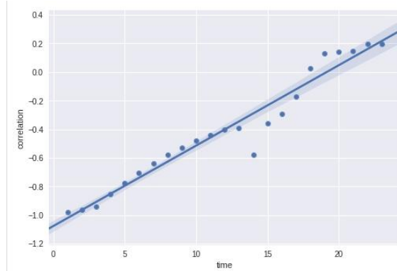
Рис. 3. Диаграмма рассеяния коэффициента корреляции для температуры и средней скорости вертикального ветра (на оси x показано время в часах, по оси y – коэффициент корреляции)
