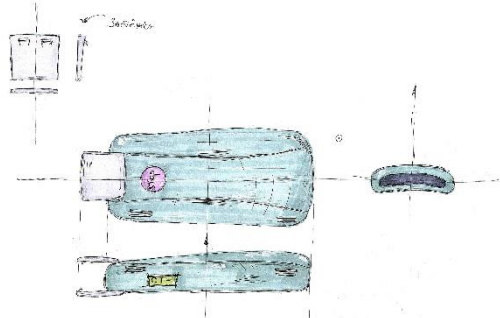
Рис. 3. Модуль управления
