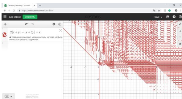
Рис. 3. Изображение в Desmos для примера 3.
