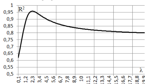
Рис. 2. Зависимость R^2 от \lambda
