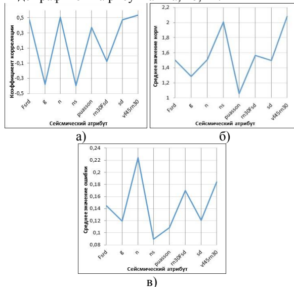
Рис. 1. а - Среднее значение коэф. корреляции; б - средняя норма разности решений систем; в - средняя ошибка прогноза
