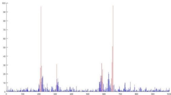
Рис. 1. Обнаружение аномальных наблюдений.
