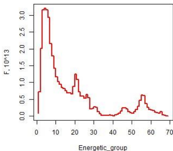
Рис. 1. Зависимость спектра нейтронов
