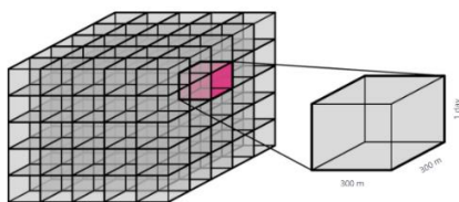
Рис. 1. Представление вокселя
