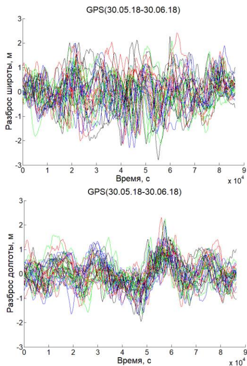
Рис. 1. Суточные вариации широты и долготы для приемника GPS (30.05.18 – 30.06.18)
