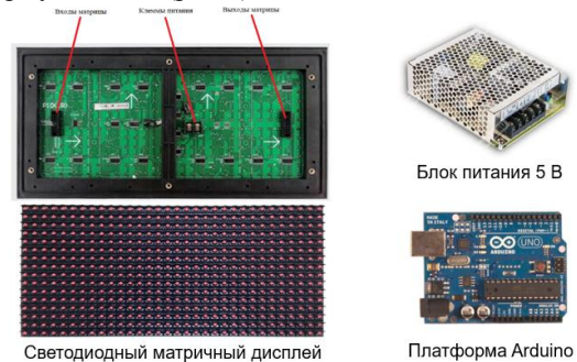
Рис. 2. Компоненты системы
