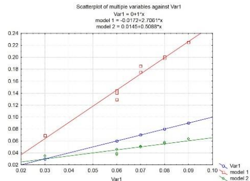
Рис. 4. Регрессионные модели распределения пористости
