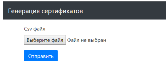
Рис. 2. Форма
