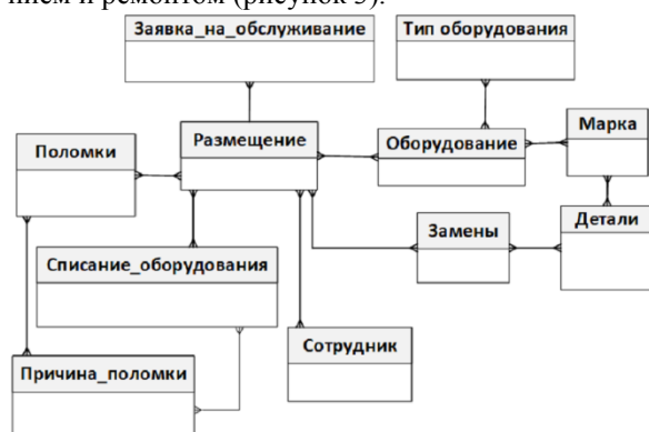
Рис. 3. ER модель
