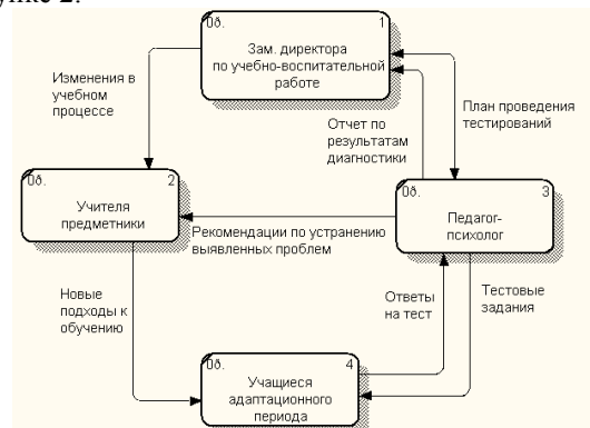
Рис. 2. Схема документооборота
