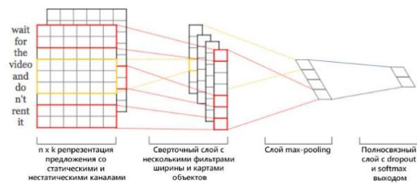
Рис. 2. Кодирование слов
