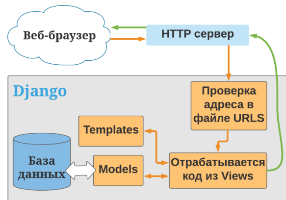
Рис. 1. Модель HTTP-запроса
