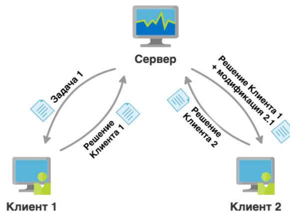
Рис. 2. Процесс проверки решения задачи.
