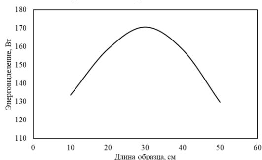
Рис. 3. Распределение энерговыделения по длине образца
