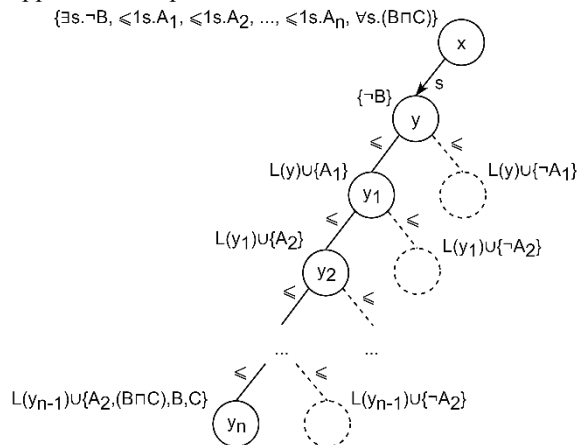
Рис. 1. Пример работы техники backjumping в предлагаемом алгоритме вывода
