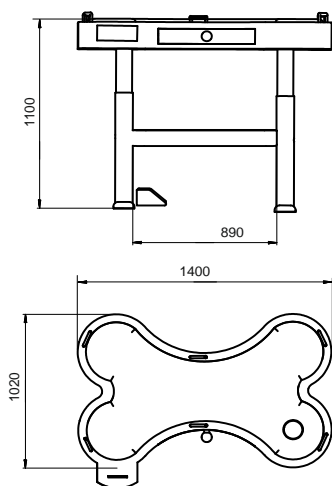
Рис. 1. Габаритный чертеж рабочего стола
