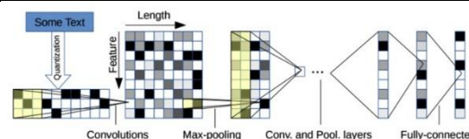
Рис. 2. Визуальное представление модели нейронной сети
