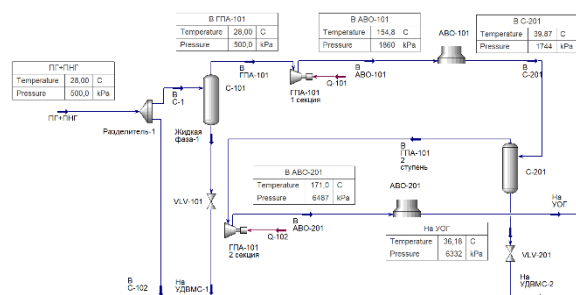
Рис. 1. Технологическая схема КС
