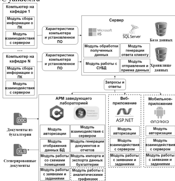
Рис. 1. Архитектура программного комплекса
