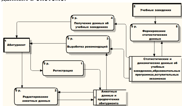
Рис. 1. Диаграмма потоков данных системы
