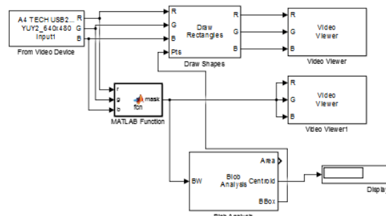
Рис. 1. Схема Simulink, применённая для распознавания объектов
