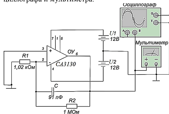
Рис. 1. Схема для моделирования шумовых характеристик OU типа CA3130
