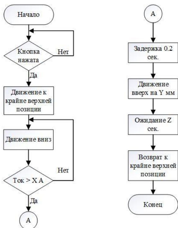
Рис. 2. Блок-схем алгоритма управления
