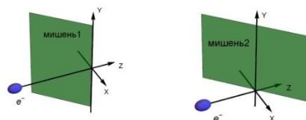
Рис. 1. Примеры геометрий мишеней ДИ от одной пластины (№1 – слева и №2 – справа), электрон движется вдоль оси Z, пластины наклонены под углом 45^\circ к оси Z
