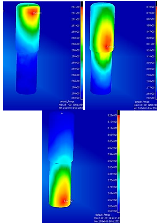
Рис. 3. Визуализация расчета температурных полей при моделировании процесса сушки изоляции пальца электродвигателей ИК-лазером
