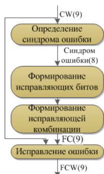
Рис. 6. Структурная схема устройства декодирования исправляющего до четырех независимых ошибок, реализующегося табличным методом
