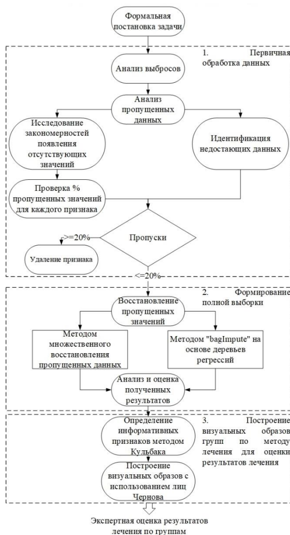
Рис. 2. Алгоритм ИТ анализа результатов лечения детей
