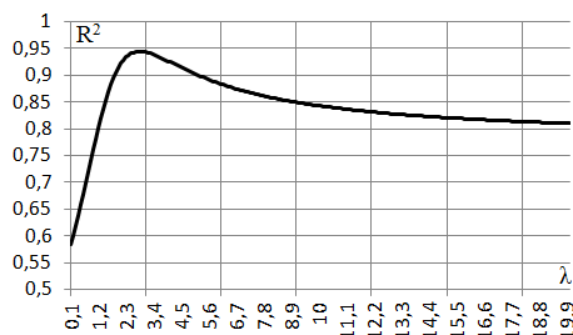
Рис. 1. Зависимость R^2 от \lambda
