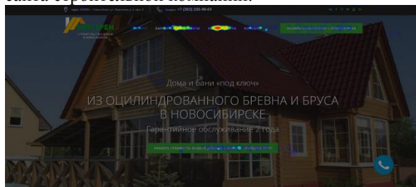
Рис. 2. Карта кликов
