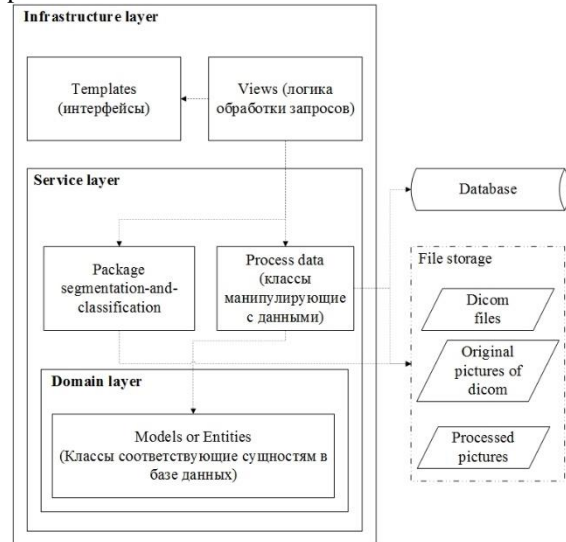
Рис. 1. Архитектура приложения
