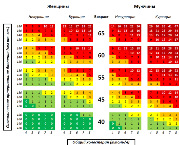
Рис. 1. Шкала SCORE
