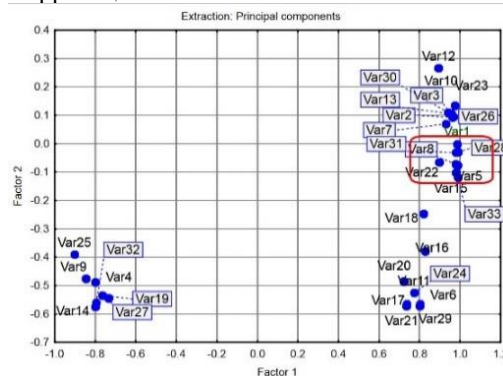
Рис. 1. График факторных нагрузок
