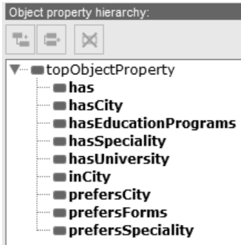
Рис. 3. Свойства объектов
