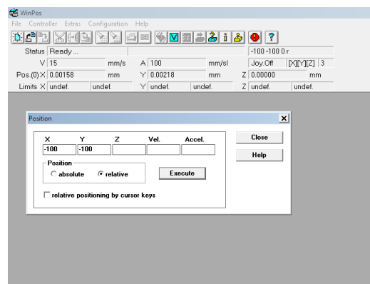
Рис. 3. Интерфейс программы
