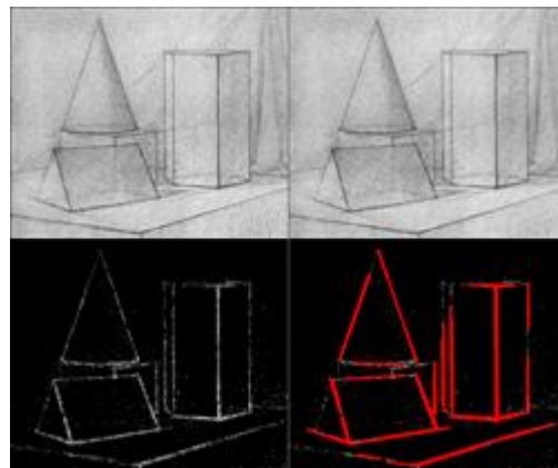
Рис. 2 Результат работы программы для зашумлённого изображения с использованием средств библиотеки OpenCV
