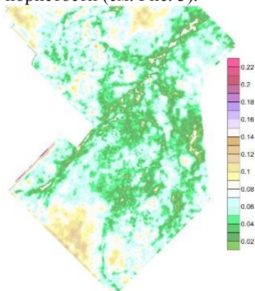
Рис. 3. Карта пористости продуктивного пласта, построенная с применением наилучшей регрессионной модели
