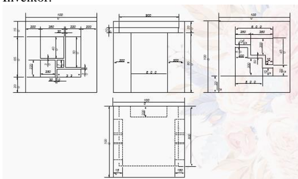
Рис. 4. Сборочный чертеж в AutoCAD одного из модулей рабочего места
