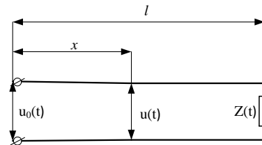
Рис. 2. Схема замещения рельсовой линии
