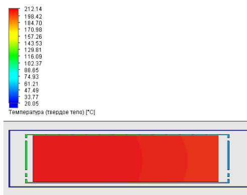
Рис. 5. Распределение температур в твердых телах при охлаждении
