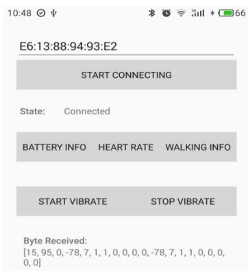
Рис. 1. Окно тест-активности при сопряжении с MiBand2 посредством API
