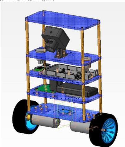
Рис. 1. Общий вид стенда
