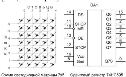
Рис. 3. Устройство светодиодной матрицы
