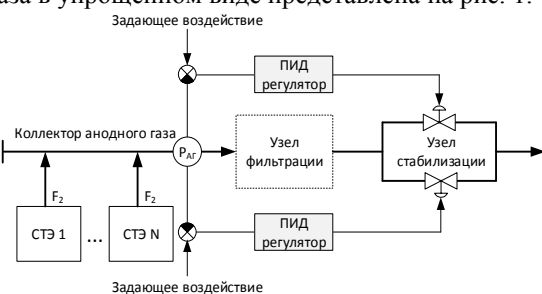
Рис. 1. Структурная схема транспортировки анодного газа
