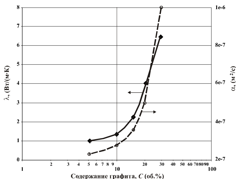
Рисунок 3.17 – Зависимости коэффициентов теплопроводности \lambda и температуропроводности \alpha от содержания графита для композиций ЛПЭНП/Г
