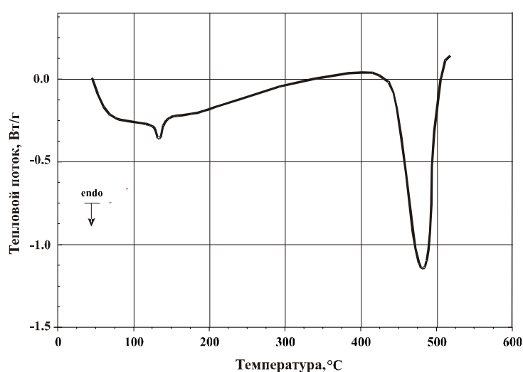
Рисунок 3.21 – Типичная ДСК-термограмма для ЛПЭНП
