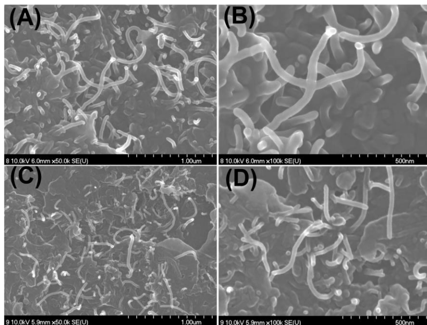
Рисунок 1.8 – СЭМ изображения, показывающие дисперсию УНТ в полимерной матрице при 0,5 вес.% (А, В) и 3 вес.% (С, D)
