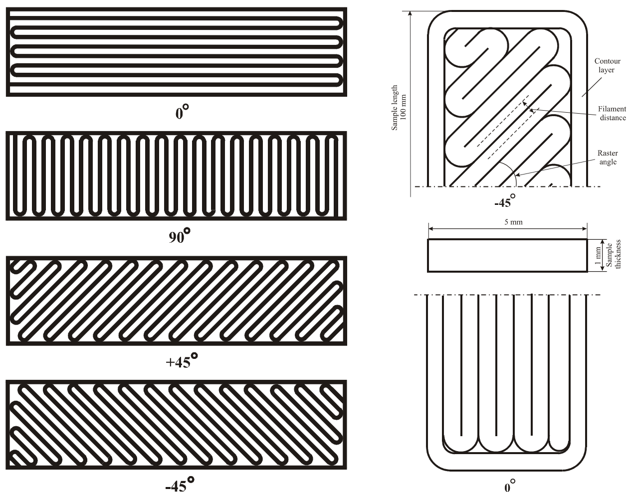
Рисунок 4.12 – Схемы наложения слоев филамента
