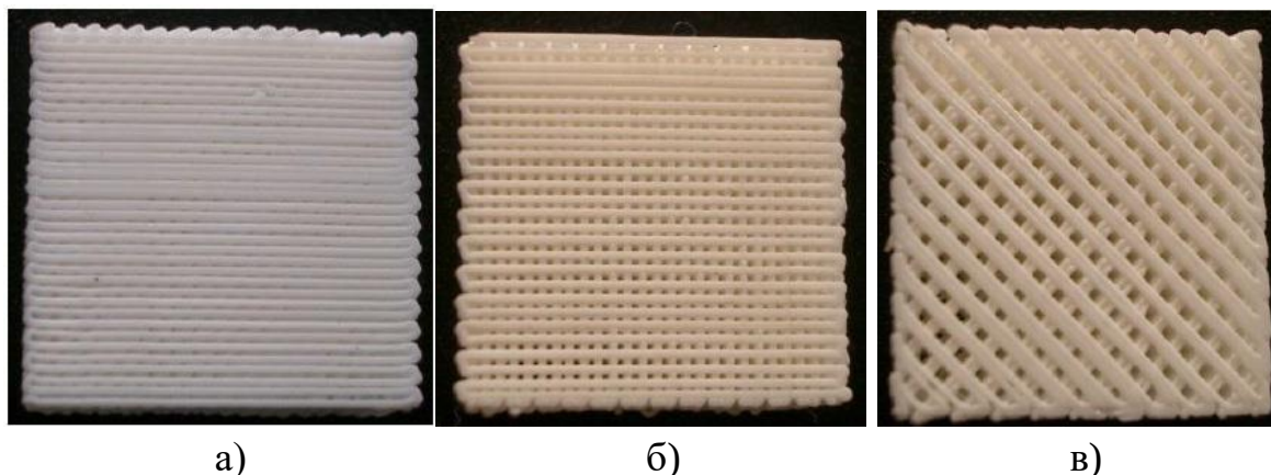
Рисунок 1.10 – Скэффолды, изготовленные в RepRap 3D-машине:
