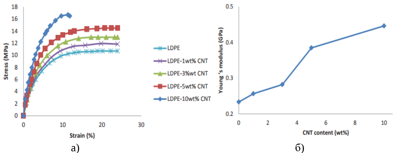
Рисунок 1.4 – Кривые напряжение-деформация (а) и модуль Юнга (б) для композиций с различным содержанием УНТ в ПЭВП
