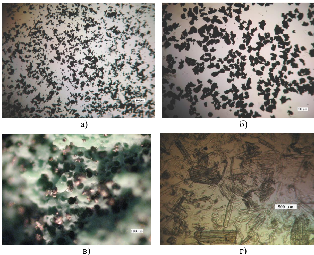
Рисунок 4.11 – Микрофотографии наполнителей: а) порошок бронзы; б) порошок меди; в) порошок карбонильного железа; г) древесная мука
