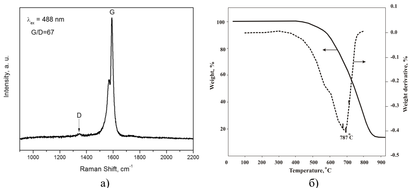
Рисунок 3.2 – ИК-спектр (а) и результаты ТГА-анализа (б) ОУНТ
