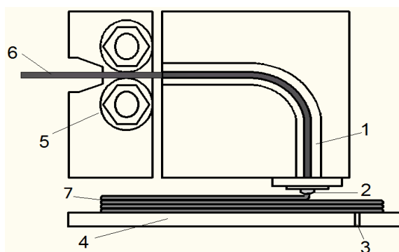
Рисунок 2.17 – Схема 3Д-печати методом послойного наплавления:
