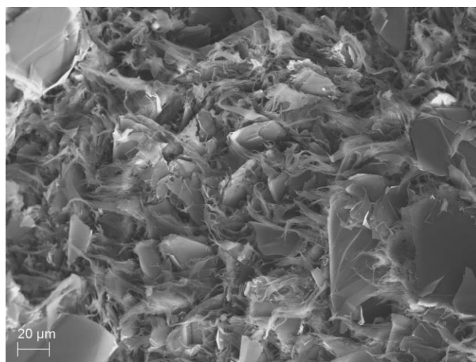
Рисунок 3.18 – СЭМ микрофотография поверхности скола образца ЛПЭНП/Г с 30 об.% графита
