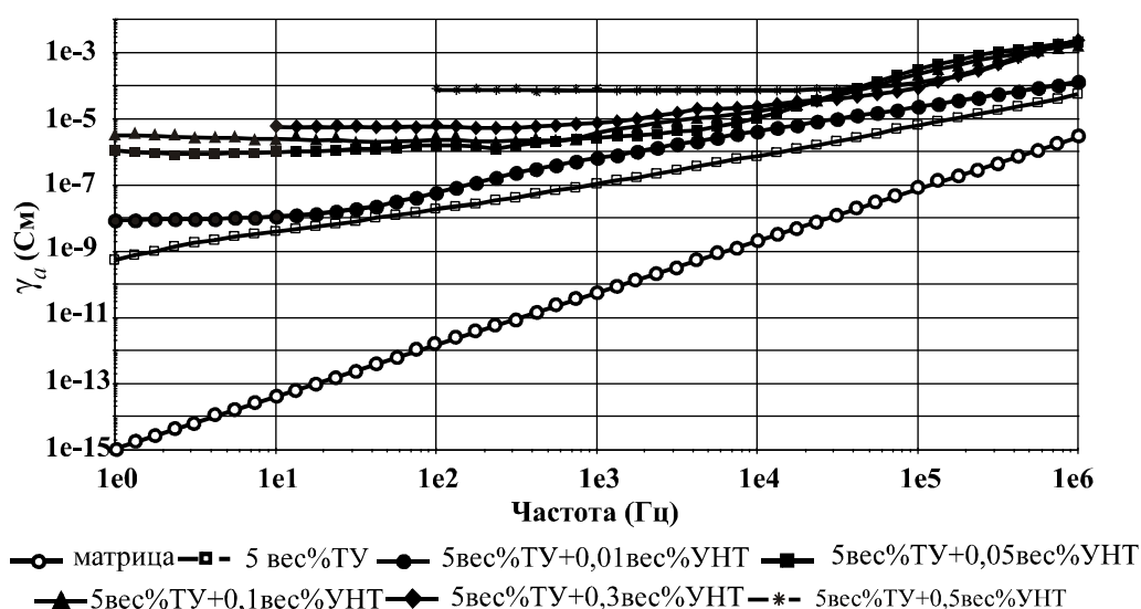
Рисунок 3.5 – Частотные зависимости \gamma_a для полимерной матрицы и композиций ЛПЭНП/ТУ/УНТ при 5 вес.% ТУ
