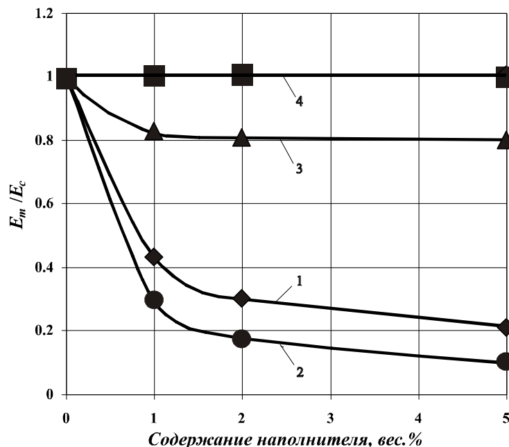
Рисунок 4.17 – Зависимости энергии смешения от содержания наполнителей в композициях: 1 – ПЛА/W; 2 – ПЛА/Pb; 3 – ПЛА/Cu; 4 – ПЭВП/W
