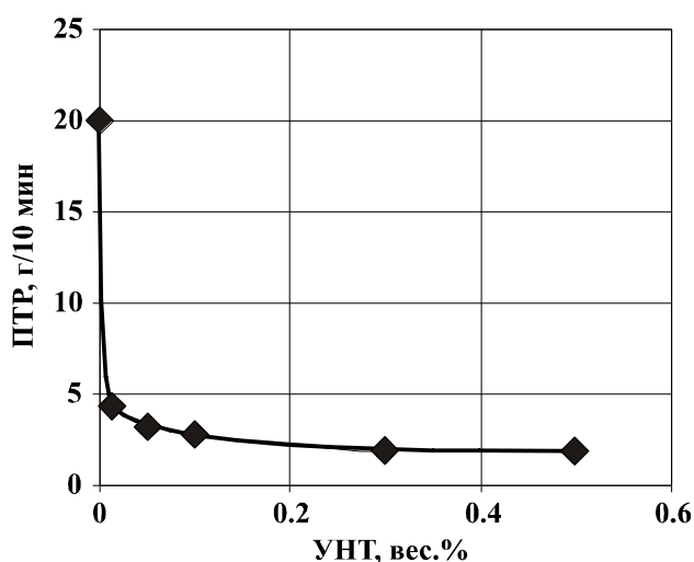
Рисунок 3.8 – Изменение величины ПТР для композиций ЛПЭНП/ТУ/УНТ при 15 вес.% ТУ от содержания УНТ
