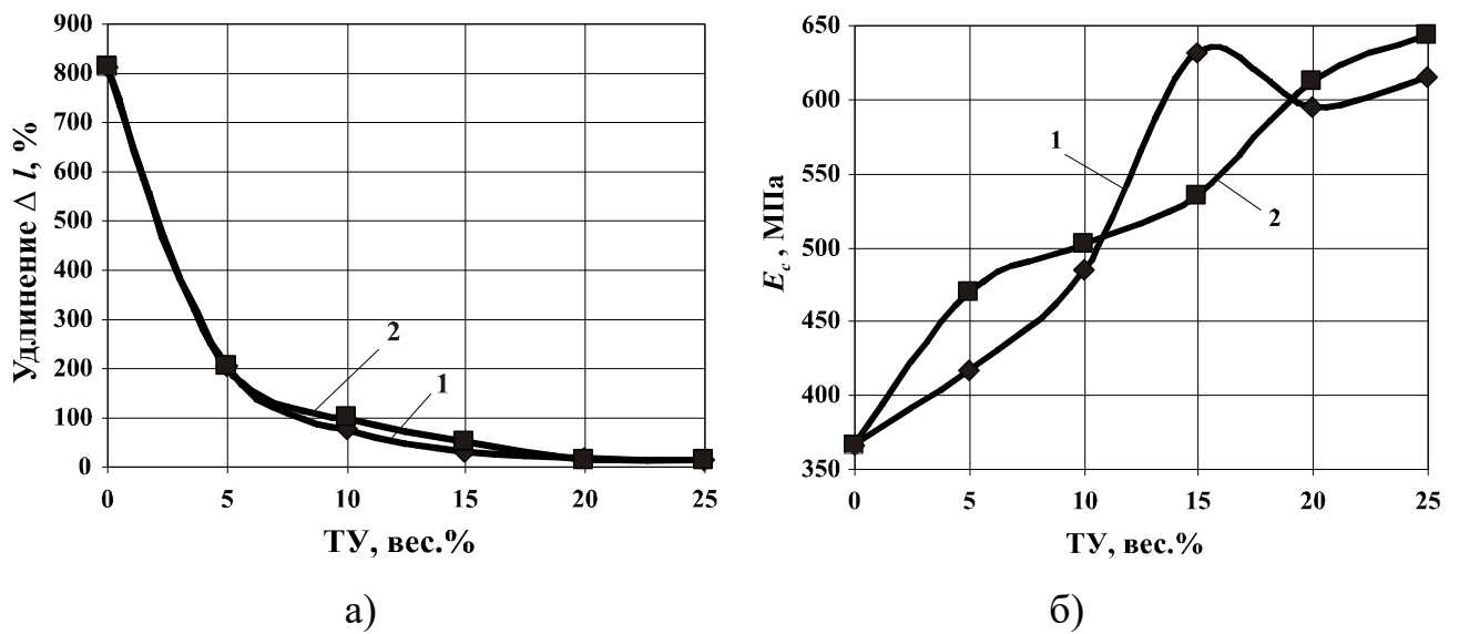
Рисунок 3.12 – Изменение удлинения при разрыве (а) и модуля Юнга (б) от содержания ТУ: 1 – для композиций ЛПЭНП/ТУ/УНТ при 0,1 вес.% УНТ; 2 – для композиций ЛПЭНП/ТУ
