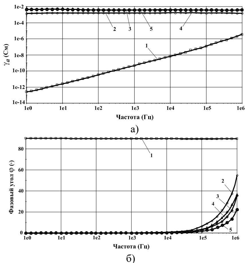
Рисунок 4.6 – Частотные зависимости \gamma_a (а) и \varphi (б) для ПЛА (1) и ПЛА/Г/УНТ композиций (2-5) с добавлением 1,0 вес.% УНТ при различном содержании графита: 2 – 5 вес.%; 3 – 10 вес.%; 4 – 20 вес.%; 5 – 30 вес.%
