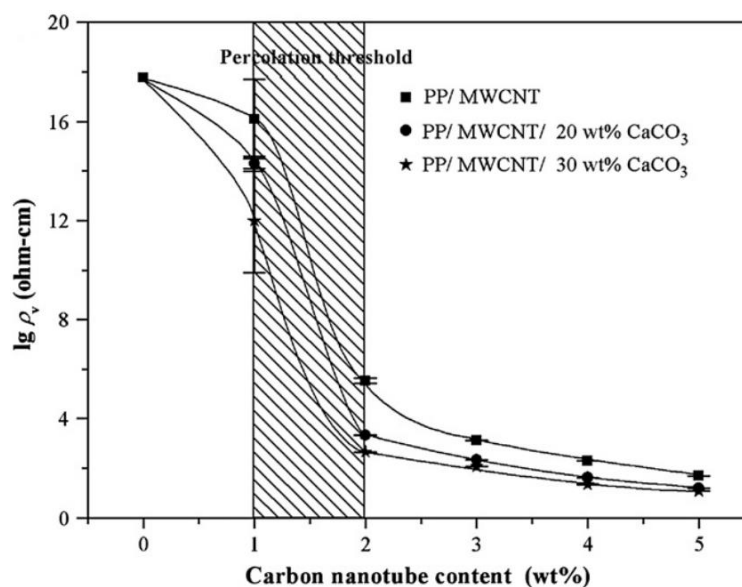
Рисунок 1.2 – Влияние CaCO 3 на электропроводность ПП/МУНТ композитов
