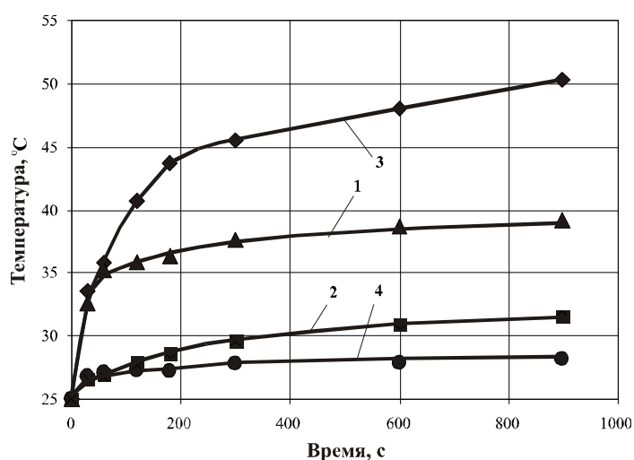
Рисунок 3.20 – Временные зависимости температуры на поверхности для образцов: 1 и 2 для ТПК с 30 об.% графита; 3 и 4 для ЛПЭНП; 1 и 3 – максимальная температура; 2 и 4 – температура на краю образца
