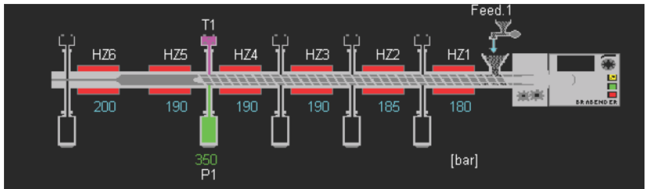
Рисунок 4.23 – Зоны нагрева двухшнекового экструдера
