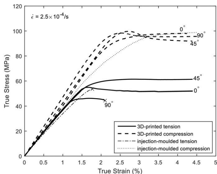
Рисунок 1.12 – Физико-механические испытания на растяжение и сжатие для всех образцов
