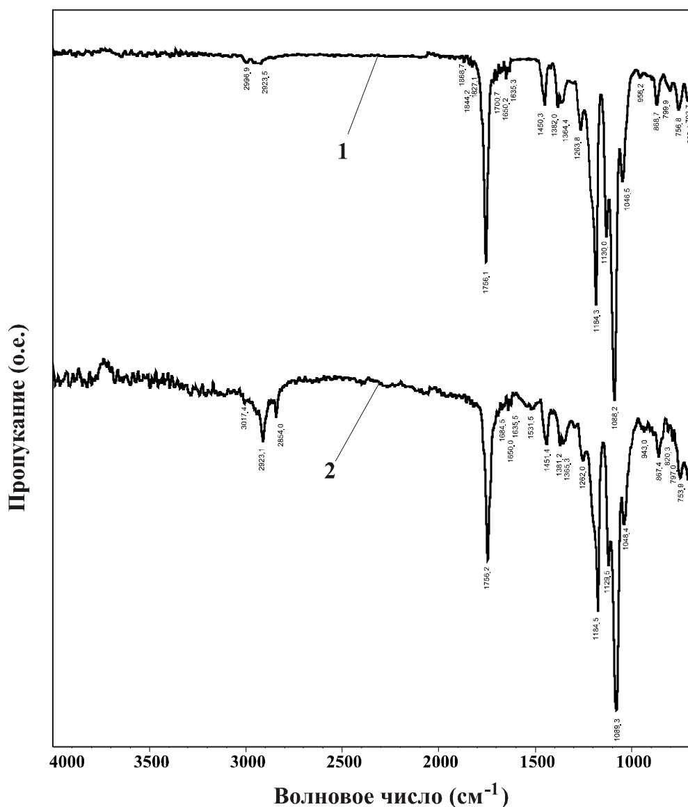
Рисунок 4.21 – ИК-спектры для ПЛА (1) и ПЛА+5,0 вес.% W (2)
