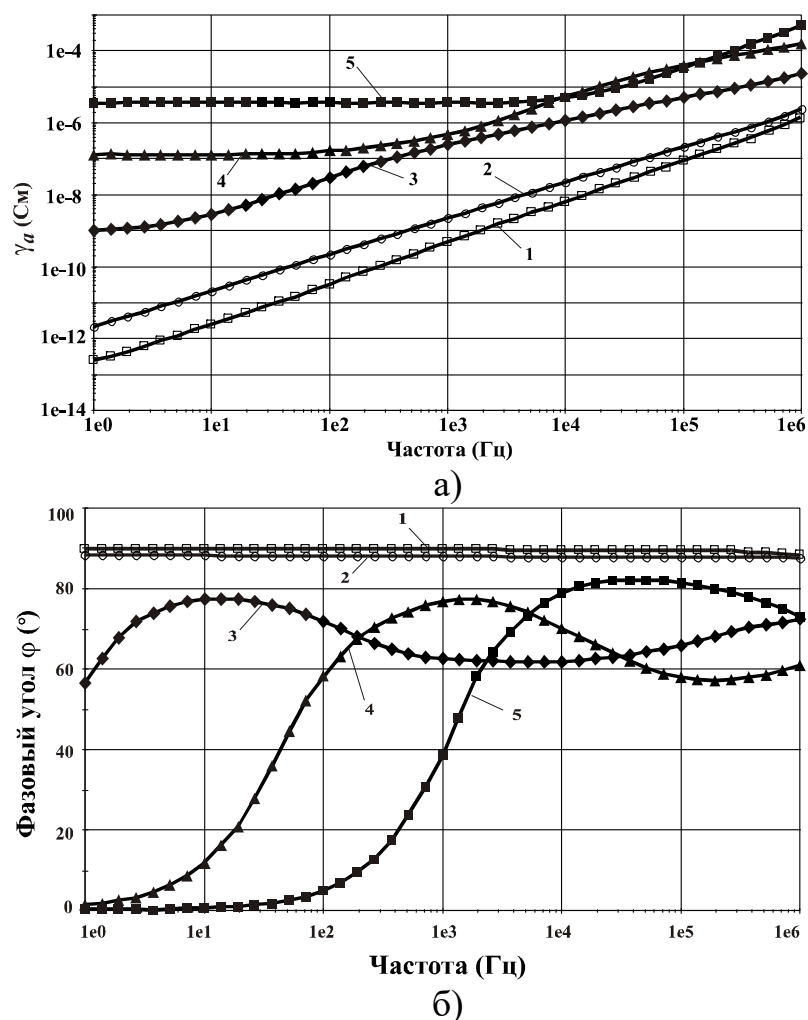
Рисунок 4.5 – Частотные зависимости \gamma_a (а) и \varphi (б) для ПЛА (1) и ПЛА/Г композиций (2-5) при различном содержании графита: 2 – 5 вес.%; 3 – 10 вес.%; 4 – 20 вес.%; 5 – 30 вес.%
