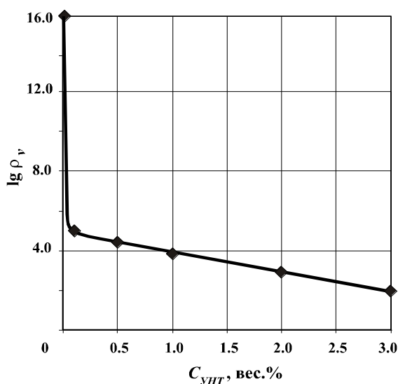
Рисунок 4.2 – Зависимость lg \rho_v = f(C_{УНТ}) для композиции ПЛА/УНТ
