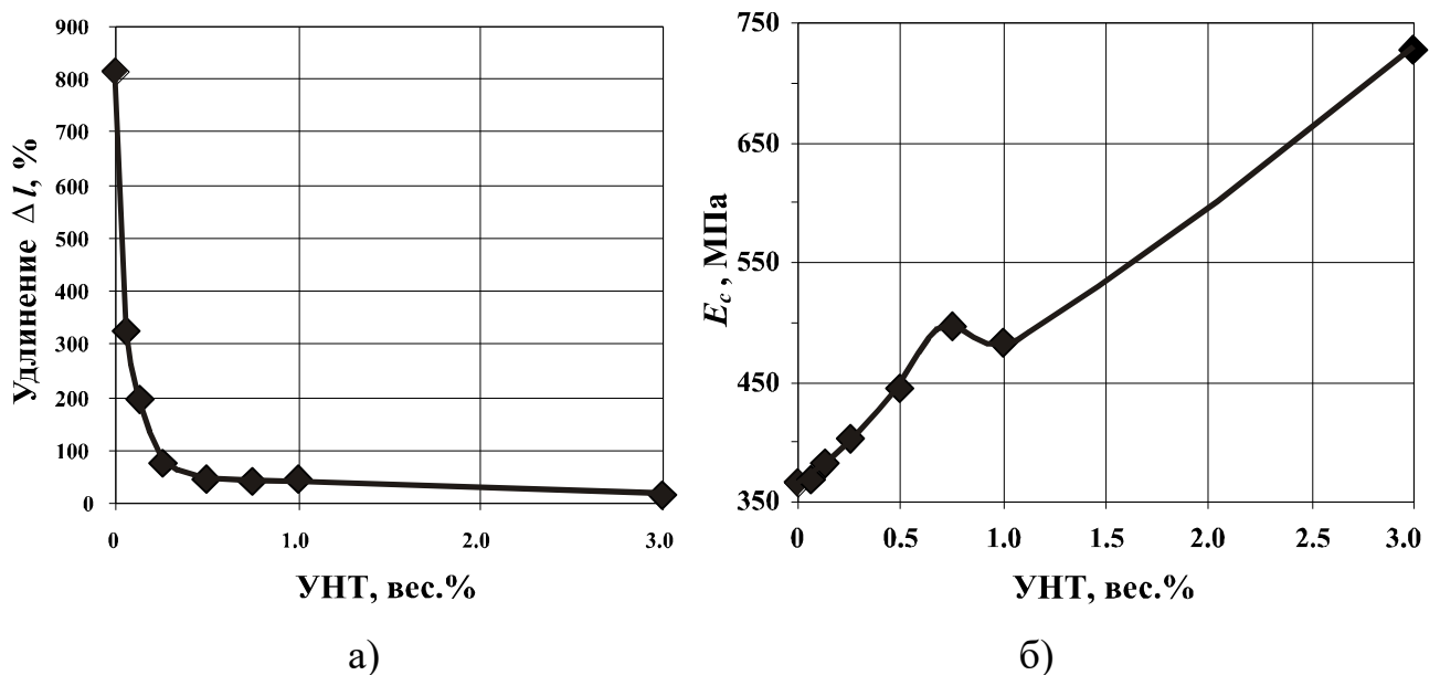
Рисунке 3.13 – Зависимости \Delta l (а) и E_c (б) от содержания УНТ для композиций ЛПЭНП/УНТ
