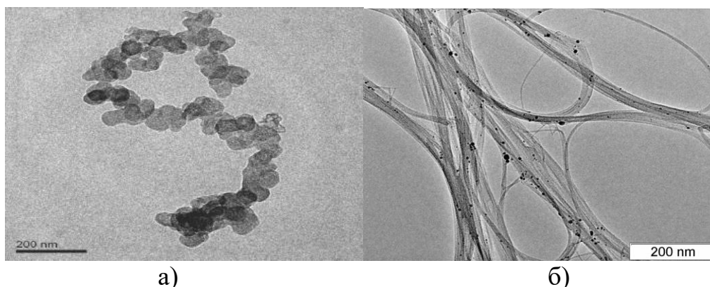
Рисунок 3.1 – Микрофотографии наполнителей: технический углерод (а); ОУНТ (б)
