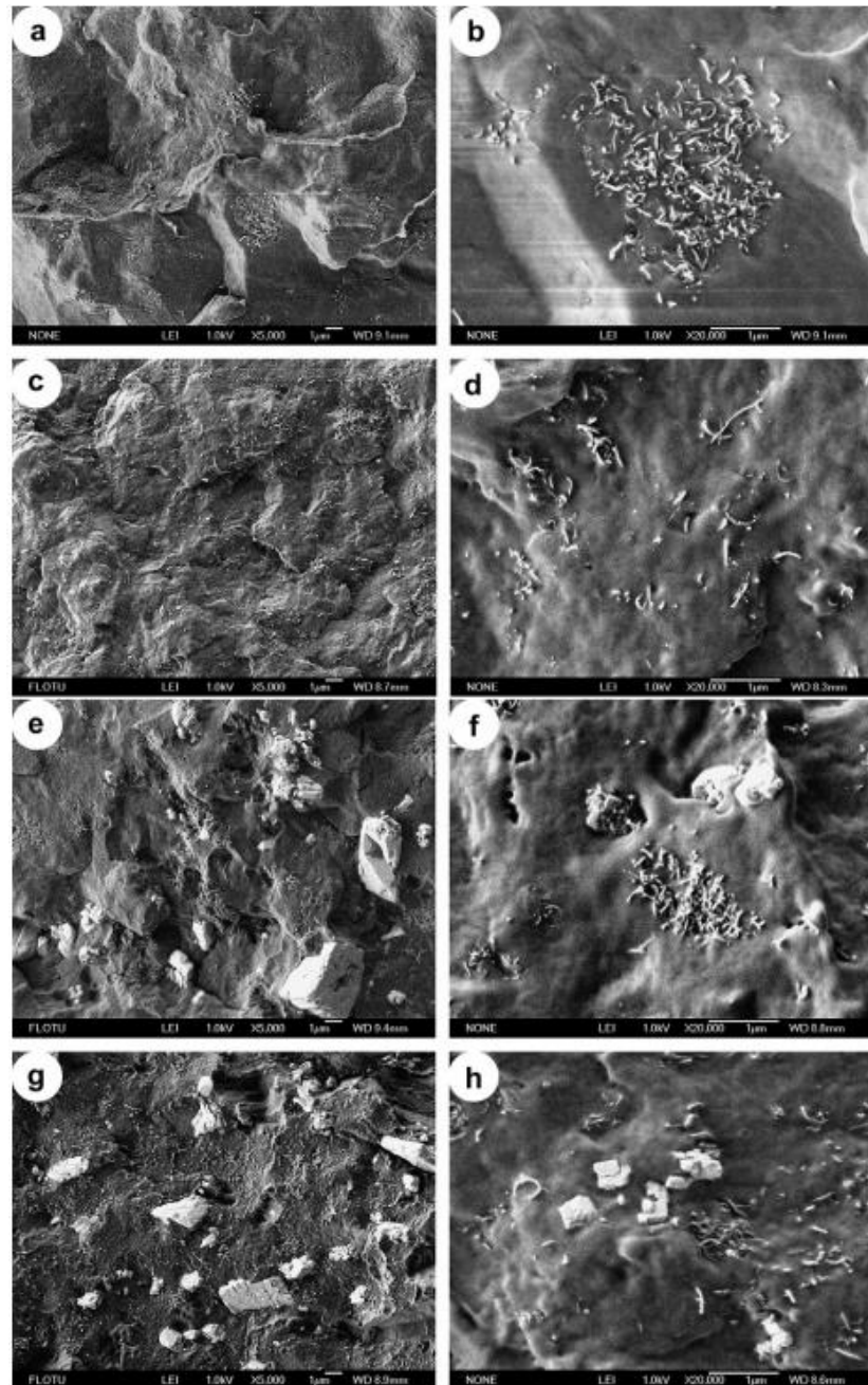
Рисунок 1.3 – СЭМ фотографии, показывающие дисперсионное состояние МУНТ: композиты ПП/5 вес.% МУНТ, полученные на самодельном оборудовании (а, b) и с помощью реометра (с, d); композиты ПП/5 вес.% МУНТ/20 вес.% \text{CaCO}_3 , полученные на самодельном оборудовании (е, f) и в реометре (g, h)
