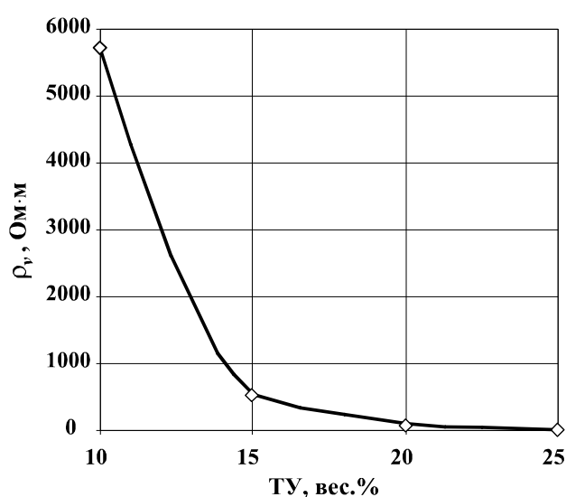
Рисунок 3.9 – Зависимость удельного объемного сопротивления композиций ЛПЭНП/ТУ от содержания ТУ
