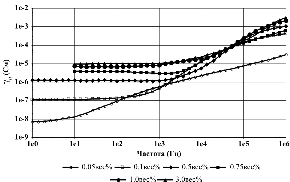
Рисунок 3.4 – Частотные зависимости \gamma_a для полимерной матрицы и композиций ЛПЭНП/ОУНТ
