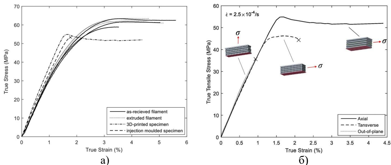
Рисунок 1.11 – Кривые напряжение–деформация для филамента и образцов (а) и для 3Д-образцов, напечатанных в X , Y и Z направлениях (б)
