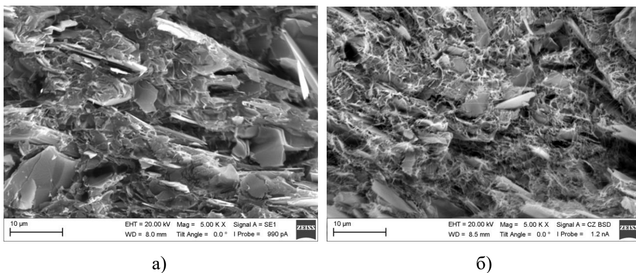
Рисунок 4.8 – СЭМ микрофотографии композиций ПЛА/Г (а) и ПЛА/Г/УНТ (б)
