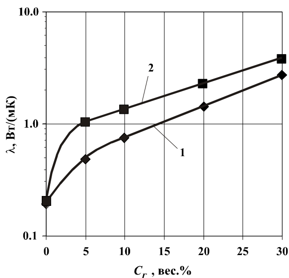
Рисунок 4.7 – Зависимость \lambda от содержания графита: 1 – без УНТ; 2 – с 1,0 вес.% УНТ
