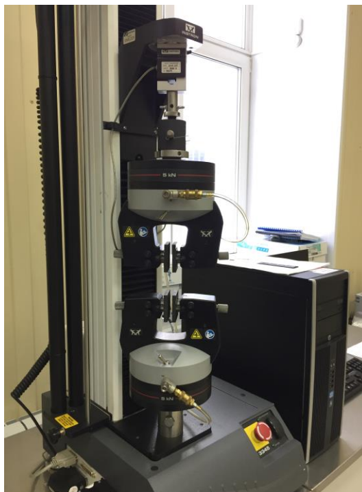
Рисунок 2.11 – Разрывная машина Instron 3345
