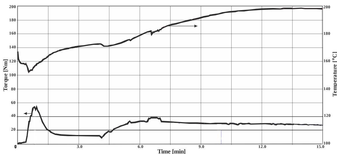
Рисунок 2.2 – Типичные зависимости нагрузки на валу смесителя и температуры переработки при подготовке композиций КПМ
