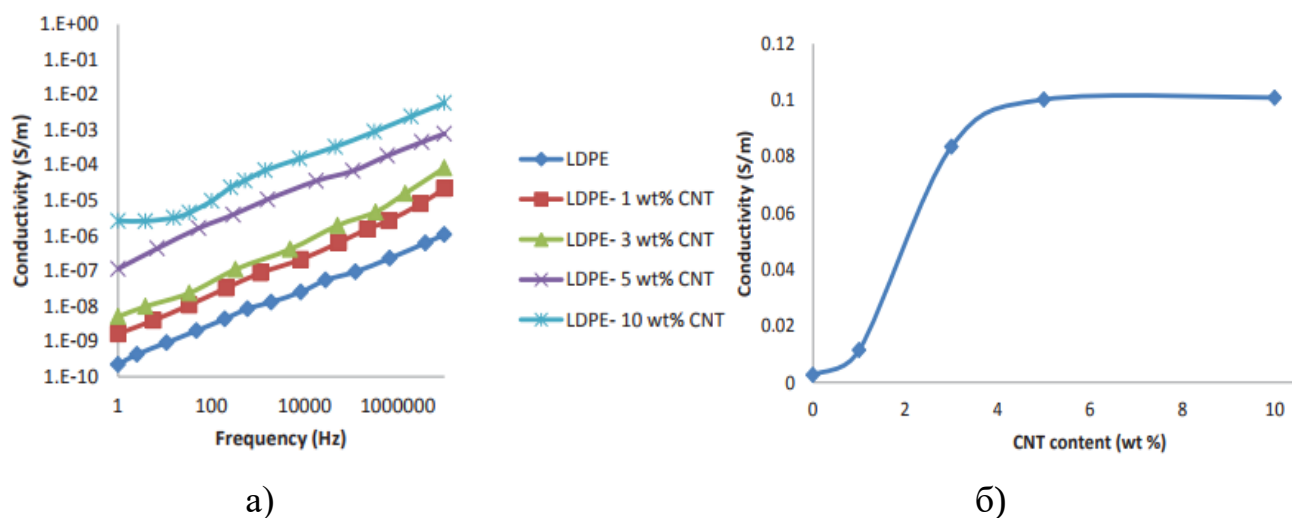
Рисунок 1.5 – Частотная зависимость электропроводности ПЭВП и композиций ПЭВП/УНТ (а) и электропроводность как функция содержания УНТ (б)
