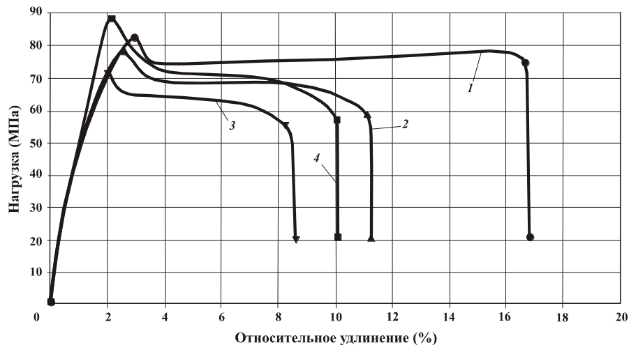
Рисунок 4.15 – Кривая нагрузка-деформация для образцов, изготовленных методом горячего прессования: 1 – исходный ПЛА; 2 – ПЛА+30 вес.% бронза; 3 – ПЛА+10 вес.% древесная мука; 4 – ПЛА+0,5 вес.% УНТ
