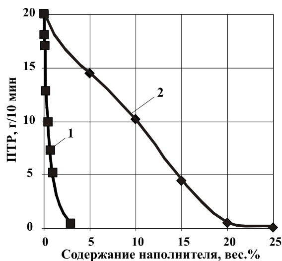
Рисунок 3.7 – Зависимости ПТР от содержания наполнителя для композиций:
