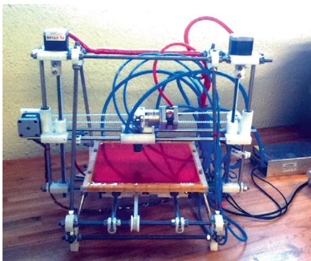
Рисунок 1.9 – RepRap Prusa 3Д-принтер
