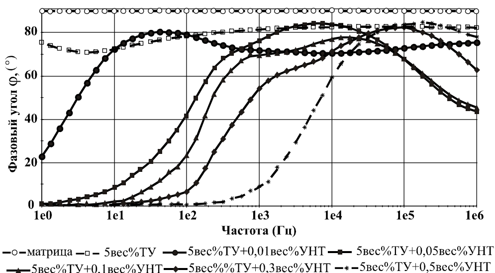
Рисунок 3.6 – Частотные зависимости фазового угла \varphi для полимерной матрицы и тройных композиций ЛПЭНП/ТУ/УНТ при содержании ТУ 5 вес.% при различном содержании УНТ
