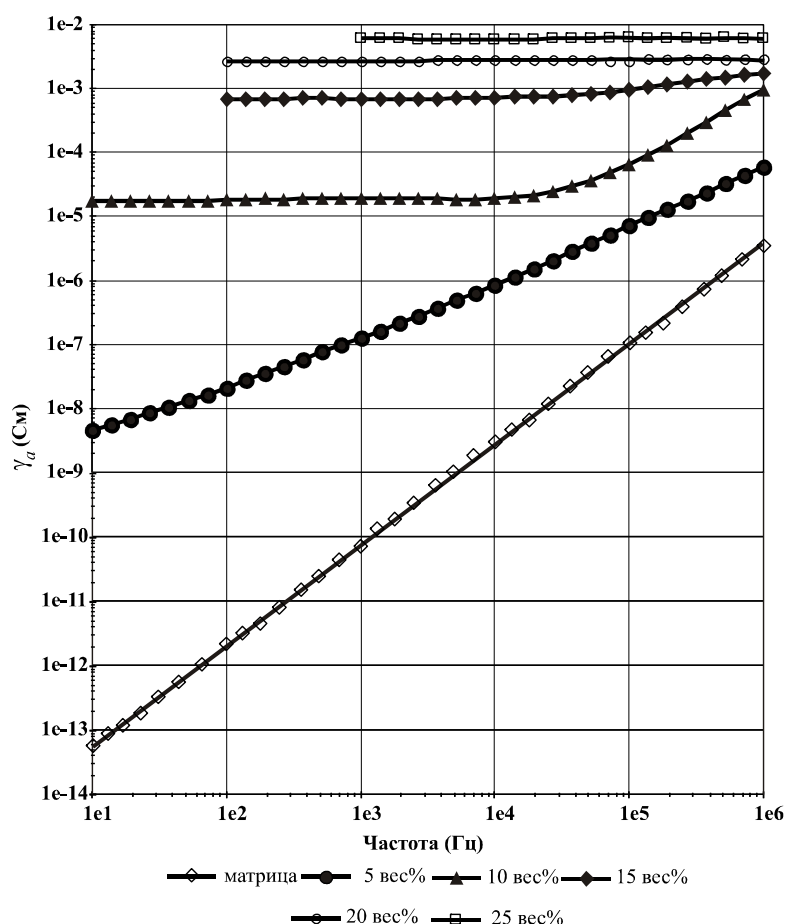
Рисунок 3.3 – Частотные зависимости \gamma_a для полимерной матрицы и композиций ЛПЭНП/ТУ
