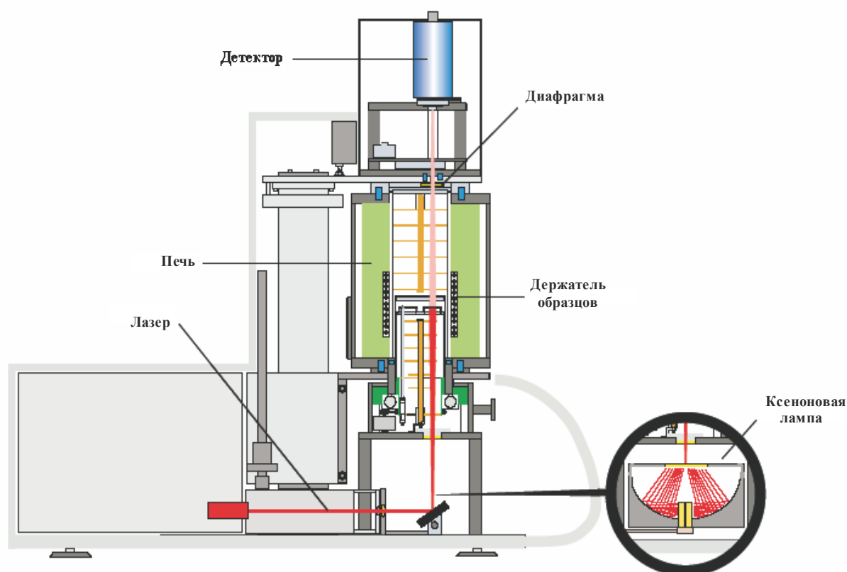
Рисунок 2.8 – Схема анализатора XFA 500 с ксеноновой лампой
