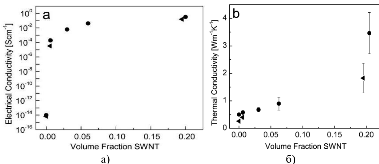
Рисунок 1.6 – Электропроводность (а) и теплопроводность(б) для композиций ОУНТ/ПЭНП(▲) и ОУНТ/ПЭВП(●) с различным содержанием ОУНТ
