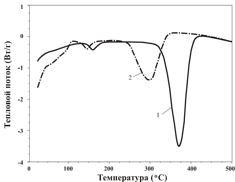
Рисунок 4.19 – Термограммы для ПЛА (1) и композиции ПЛА+5,0 вес.% W (2)
