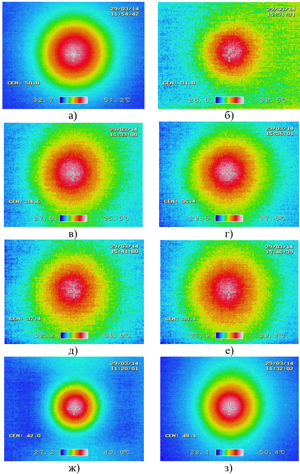
Рисунок 3.19 – Термограммы источника тепла (а), поверхности образца ТПК (б-е) и образца ЛПЭНП (ж, з) при различных временах: б – 30 с; в – 120 с; г – 300 с; д – 600 с; е – 900 с; ж – 180 с; з – 900 с
