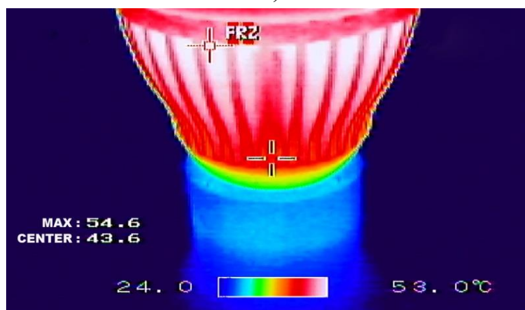
Рисунок 3.23 – ИК-термограммы поверхности СДЛ с радиаторами, изготовленными из различных ТПК: а) ТПК № 1; б) ТПК № 2; в) ТПК № 3
