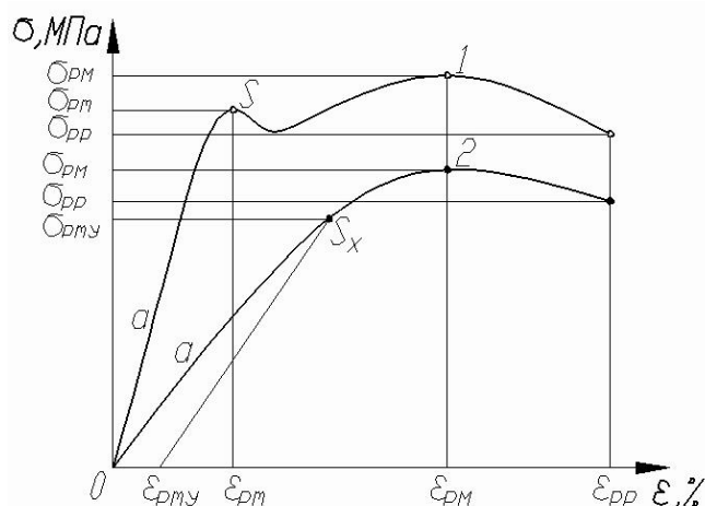
Рисунок 2.12 – Зависимости напряжение-деформация: 1 – для материала, имеющего предел текучести; 2 – для материала, не имеющего предела текучести. a – участки линейного изменения на начальном участке зависимостей напряжение-деформация; S – предел текучести; S_x – условный предел текучести [по ГОСТ 11262-80]
