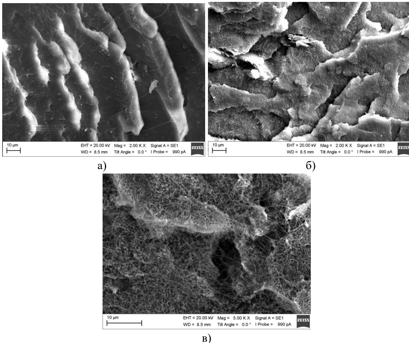
Рисунок 4.3 – СЭМ микрофотографии для композиций ПЛА/УНТ:
