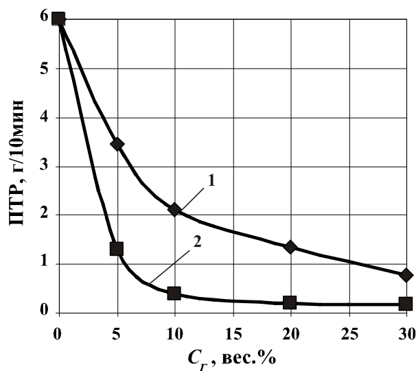
Рисунок 4.9 – Зависимость ПТР для двойных и тройных композиций на основе ПЛА от содержания графита: 1 – без УНТ; 2 – с 1.0 вес.% УНТ
