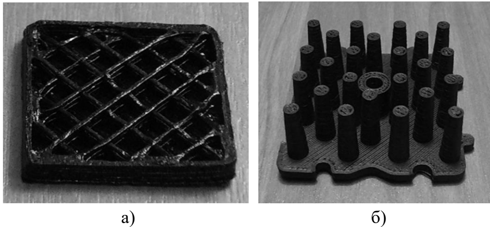
Рисунок 4.10 – Прототипы 3Д-скэффолда (а) и радиатора охлаждения (б), изготовленные методом 3Д-печати
