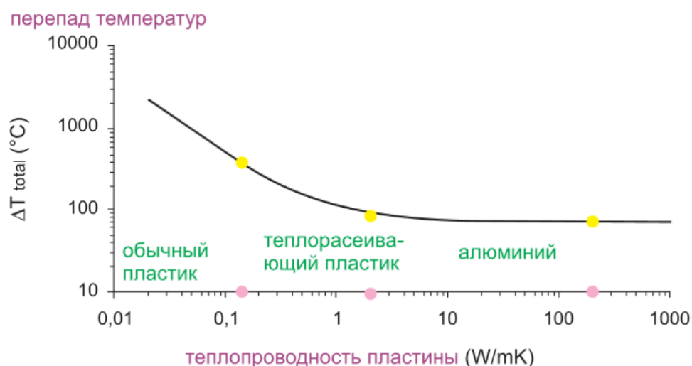
Рисунок 1.7 – Влияние теплопроводности материала пластины на неравномерность ее температурного поля при точечном нагреве
