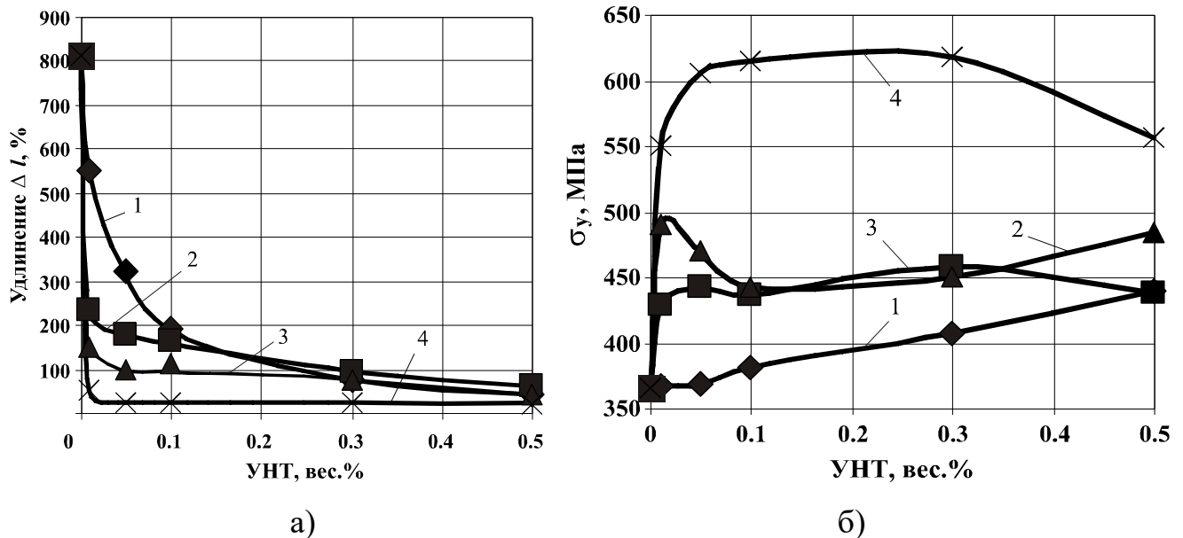
Рисунок 3.14 – Зависимости \Delta l (а) и \sigma_y (б) от содержания УНТ для композиций ЛПЭНП/ТУ/УНТ с различным содержанием ТУ:
