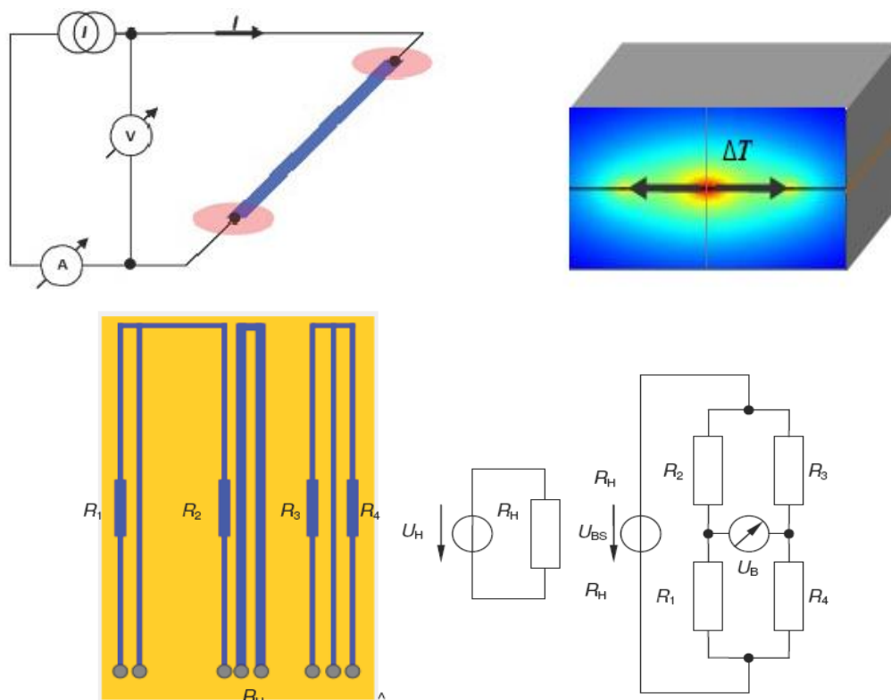
Рисунок 2.6 – Принцип измерения \lambda и \alpha с помощью анализатора ТНВ-100
