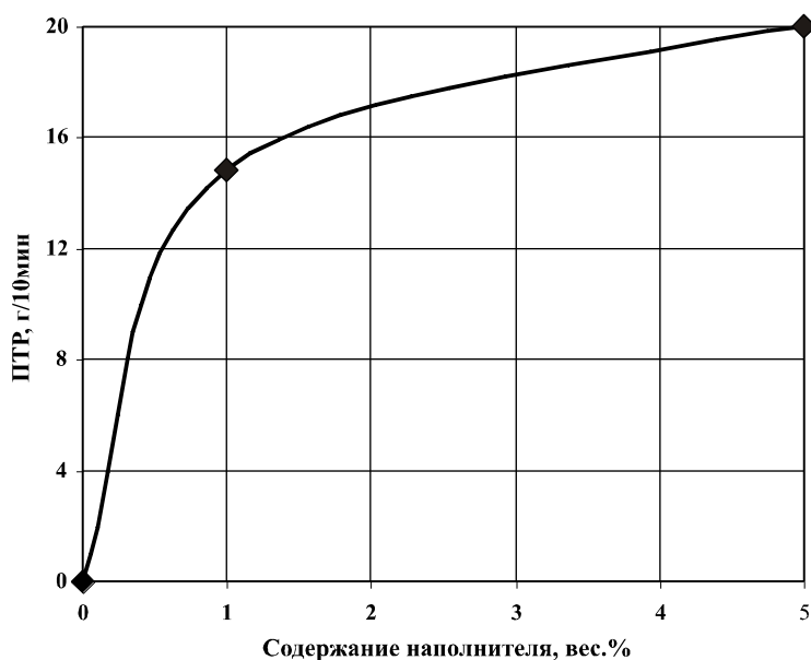
Рисунок 4.18 – Зависимость ПТР от содержания наполнителя, измеренная при 150°C
