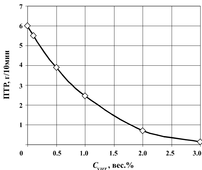
Рисунок 4.4 – ПТР для ПЛА/УНТ композиций в зависимости от содержания УНТ
