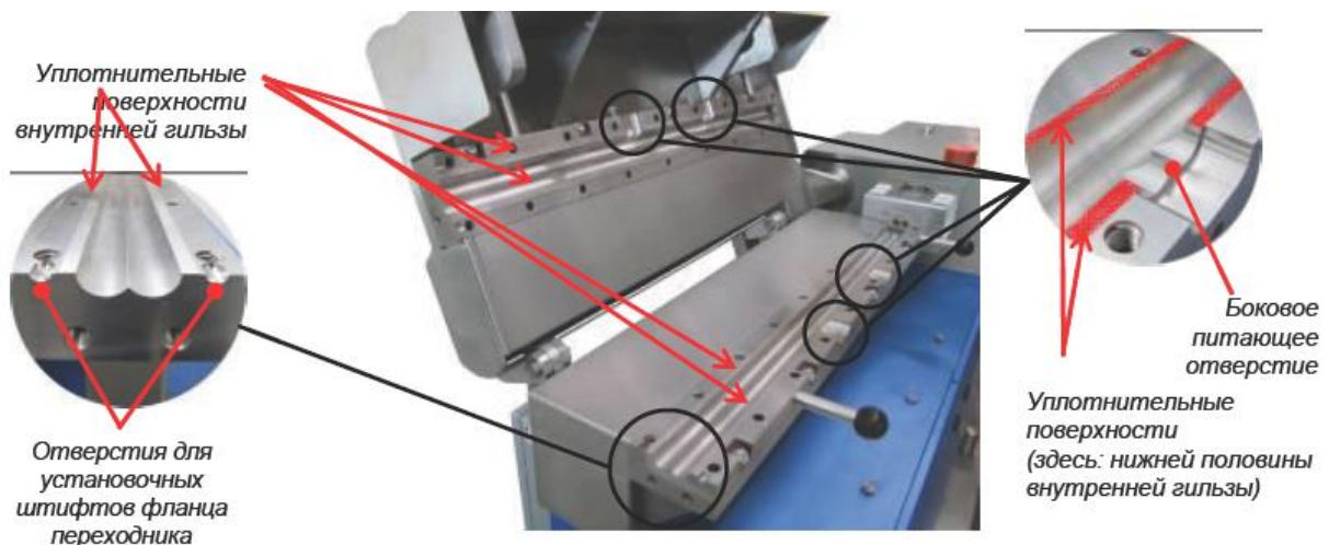
Рисунок 4.24 – Внешний вид экструдера с открытым цилиндром
