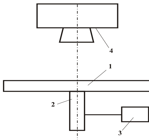
Рисунок 2.10 – Схема экспериментальной установки: 1 – образец, 2 – источник тепла, регулятор температуры (3), ИК-камера (4)
