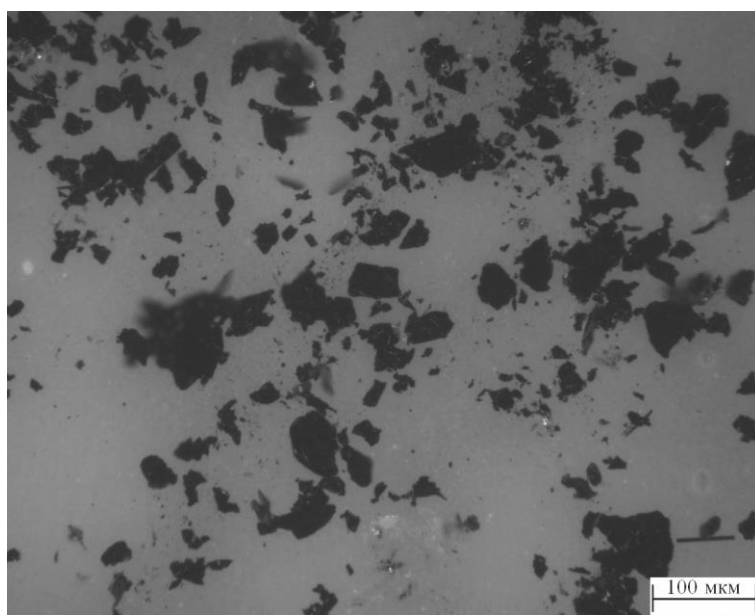
Рисунок 3.15 – СЭМ микрофотография частиц натурального графита
