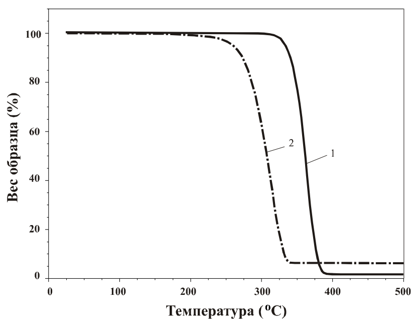
Рисунок 4.20 – Результаты ТГА-анализа для ПЛА (1) и композиции ПЛА+5,0 вес.% W (2)
