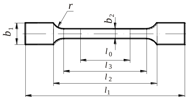
Рисунок 2.14 – Форма образца для испытаний на растяжение
