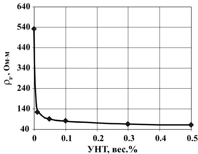
Рисунок 3.11 – Зависимость удельного объемного сопротивления композиции ЛПЭНП/ТУ/УНТ при 15 вес.% ТУ от содержания УНТ
