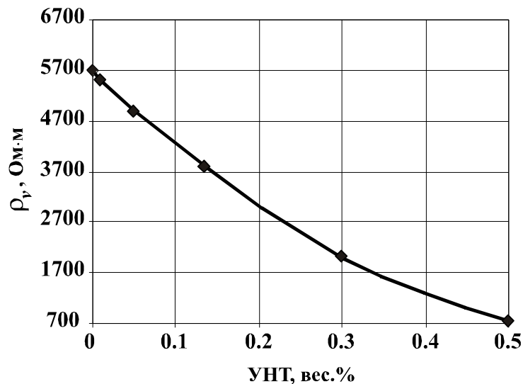
Рисунок 3.10 – Зависимость удельного объемного сопротивления композиций ЛПЭНП/ТУ/УНТ при 10 вес.% ТУ от содержания УНТ
