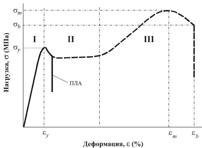
Рисунок 4.14 – Типичная кривая нагрузка-деформация для термопластов
