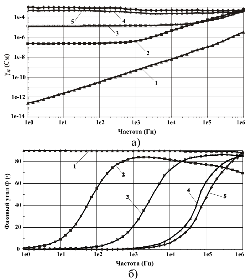
Рисунок 4.1 – Частотные зависимости \gamma_a (а) и \varphi (б) для ПЛА (1) и ПЛА/УНТ композиций (2-5) с различным содержанием УНТ: 2 – 0,1 вес.%; 3 – 1,0 вес.%; 4 – 2,0 вес.%; 5 – 3,0 вес.%
