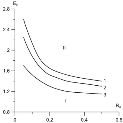
Рис. 3. Области стационарного (I) и колебательного (II) режимов распространения фронта горения при: 1 – Le = 10^{-4} , 2 – Le = 5 \cdot 10^{-5} , 3 – Le = 10^{-5} , \gamma = 0.14286 , \beta = 0.05
