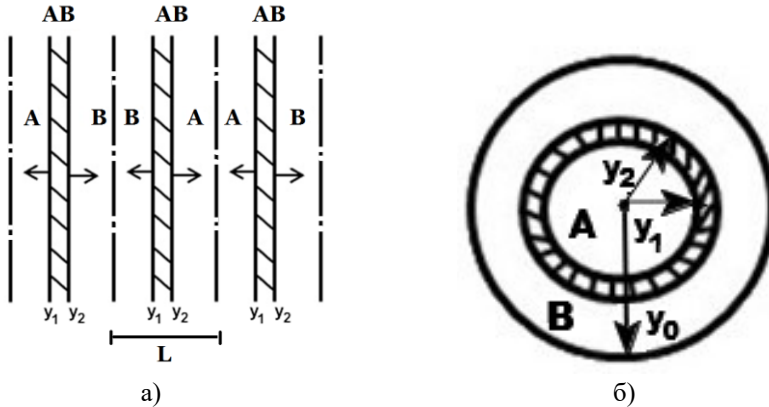
Рис. 1. Реакционные ячейки: а – плоские; б - сферические
