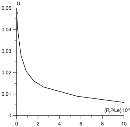
Рис. 2. Зависимость скорости горения U от отношения R_0^2/Le .
