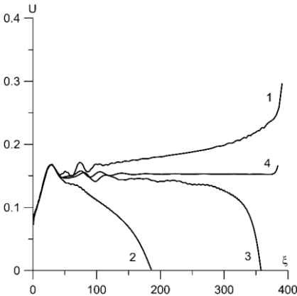
Рис. 8. Зависимость скорости пламени от координаты при значениях числа Bi :
