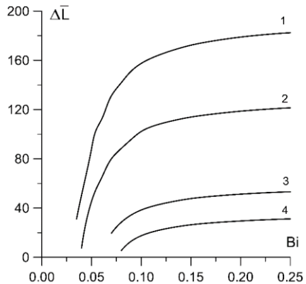
Рис. 9. Зависимость толщины недогоревшего слоя от числа Bi при углах
