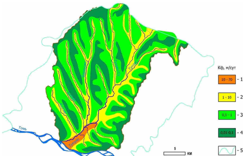
Рис. 7. Фильтрационная неоднородность водоносного комплекса юрских отложений.
