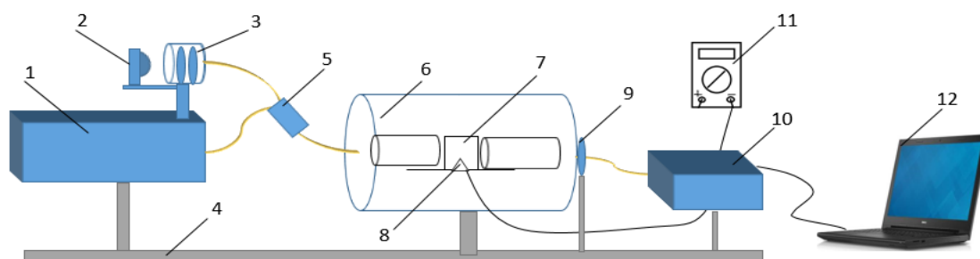
Рисунок 9 – Схема стенда ((1 – лазер, 2 – чип, 3 – телескопическая система, 4 – оптический рельс и стойки крепления (рейтеры), 5 – световод с делителем, 6 – печь, 7 – кювета для люминофора, 8 –термопара, 9 – линза, 10 – спектрофотометр, 11 – мультиметр, 12 –ноутбук)
