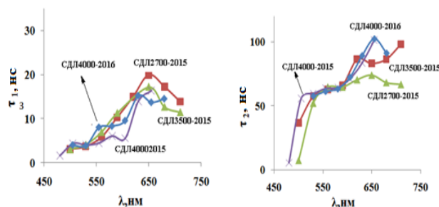
Рисунок 6 – Дисперсия времени затухания люминесценции люминофоров серии СДЛ характеристические времена короче, чем в длинноволновой области спектра. Различие возможно обусловлено различиям центров свечения.
