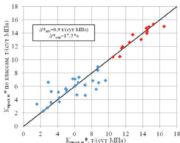
Рис. 4. Сопоставление фактических и модельных значений коэффициента продуктивности по нефти, рассчитанных по уравнениям (3) и (4) для выделенных классов (синий – 1 класс, красный – 2 класс)
