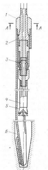
Рис.18. Снаряд СНБ-КО
