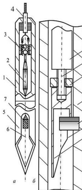
Рисунок 12 – Схема устройства ориентатора УШО (а) и положение наконечника ориентатора в переходнике над отклонителем при его ориентировании (б):
