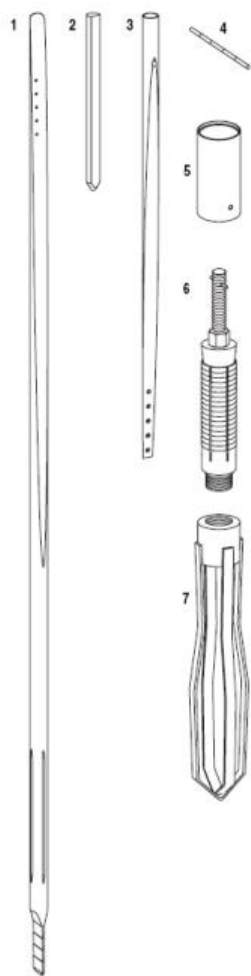
Рисунок 10 – отклоняющий клин марки BOART LONGYEAR
