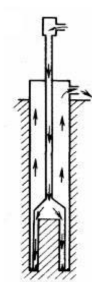
Рисунок 5 – Принципиальная схема прямой промывки скважин при бурении с отбором керна
