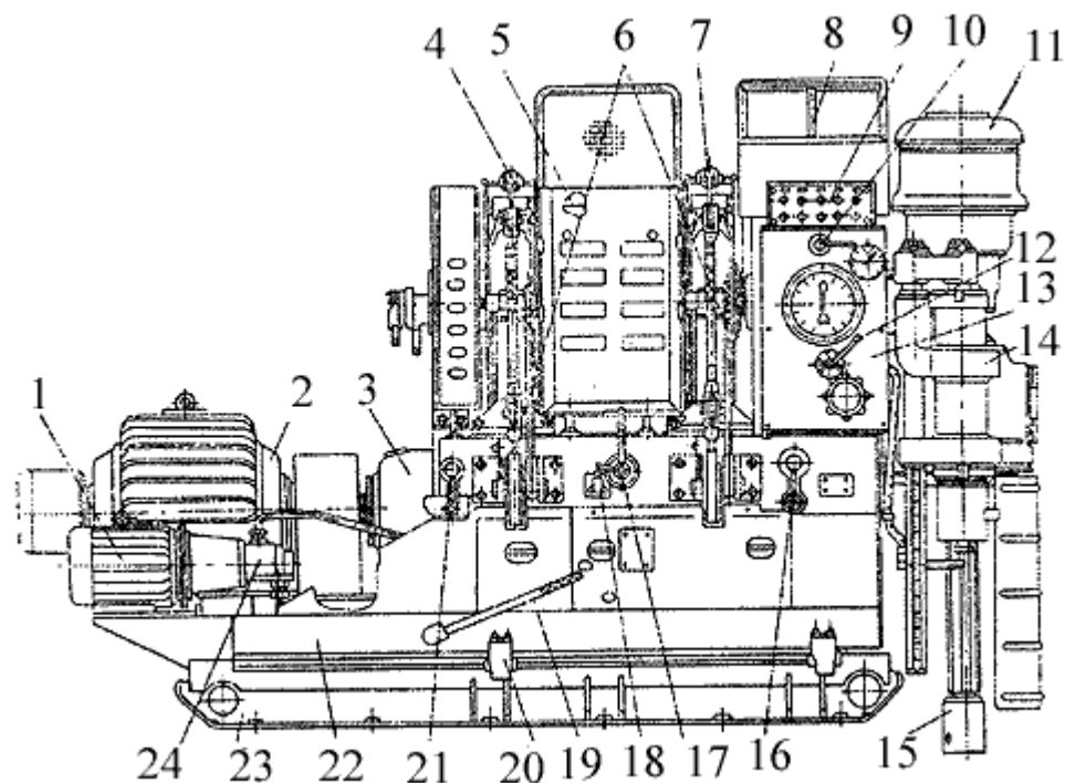
Рисунок 8 – Общий вид бурового станка ЗИФ-1200МР:
