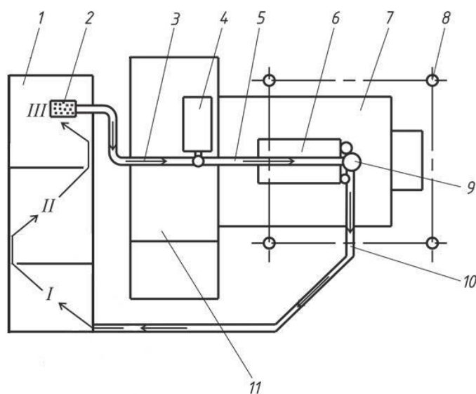
Рисунок 14 – Типовая схема циркуляционной системы очистки промывочной жидкости при бурении геологоразведочных скважин:
