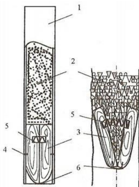
Рисунок 11 – Пробка-искусственный забой:
