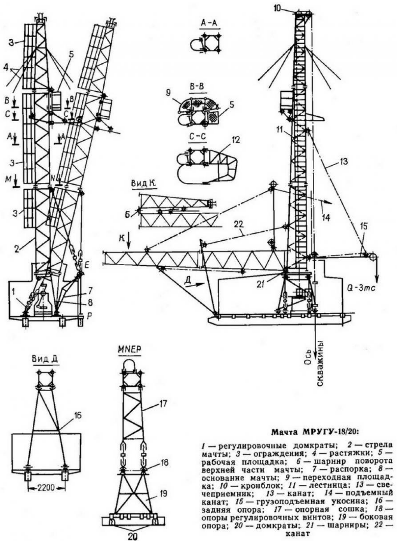
Рисунок 9 – Схема мачты МРУГУ-18/20
