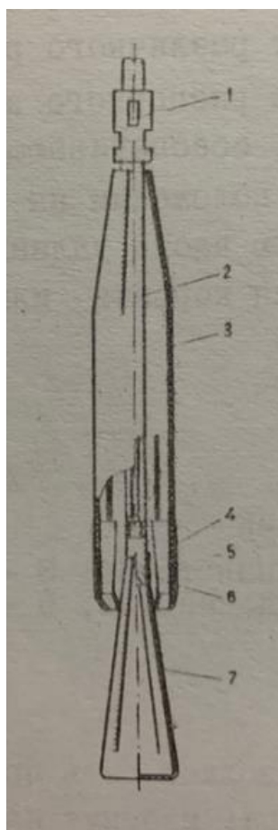
Рис.17. Пробка конструкции В.М.Шаповалова
