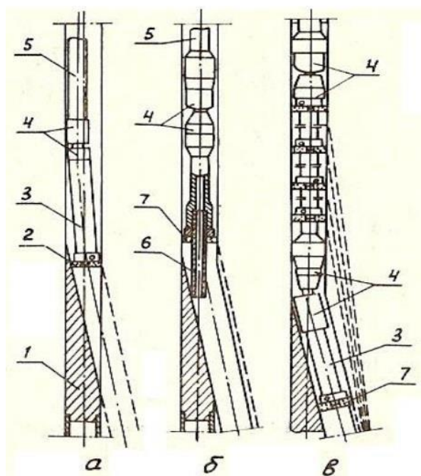
Рисунок 13 – Схема отбуривания пилот-скважины:
