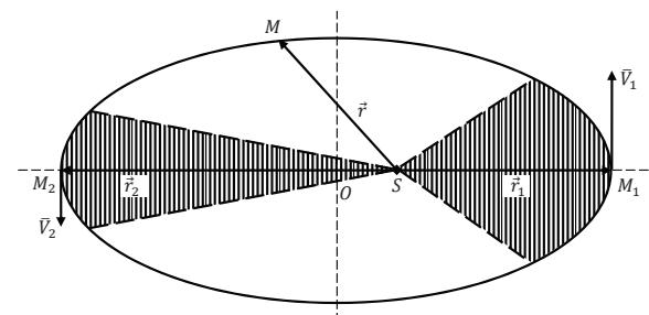
Рис. 1. Схема, поясняющая второй закон И. Кеплера (заштрихованные участки имеют равные площади)
