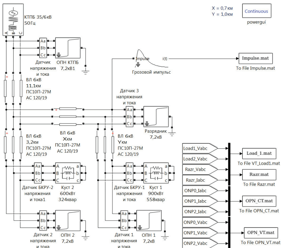
Рис. 2. Схема имитационной модели участка распределительной сети электроснабжения кустов нефтедобывающих скважин
